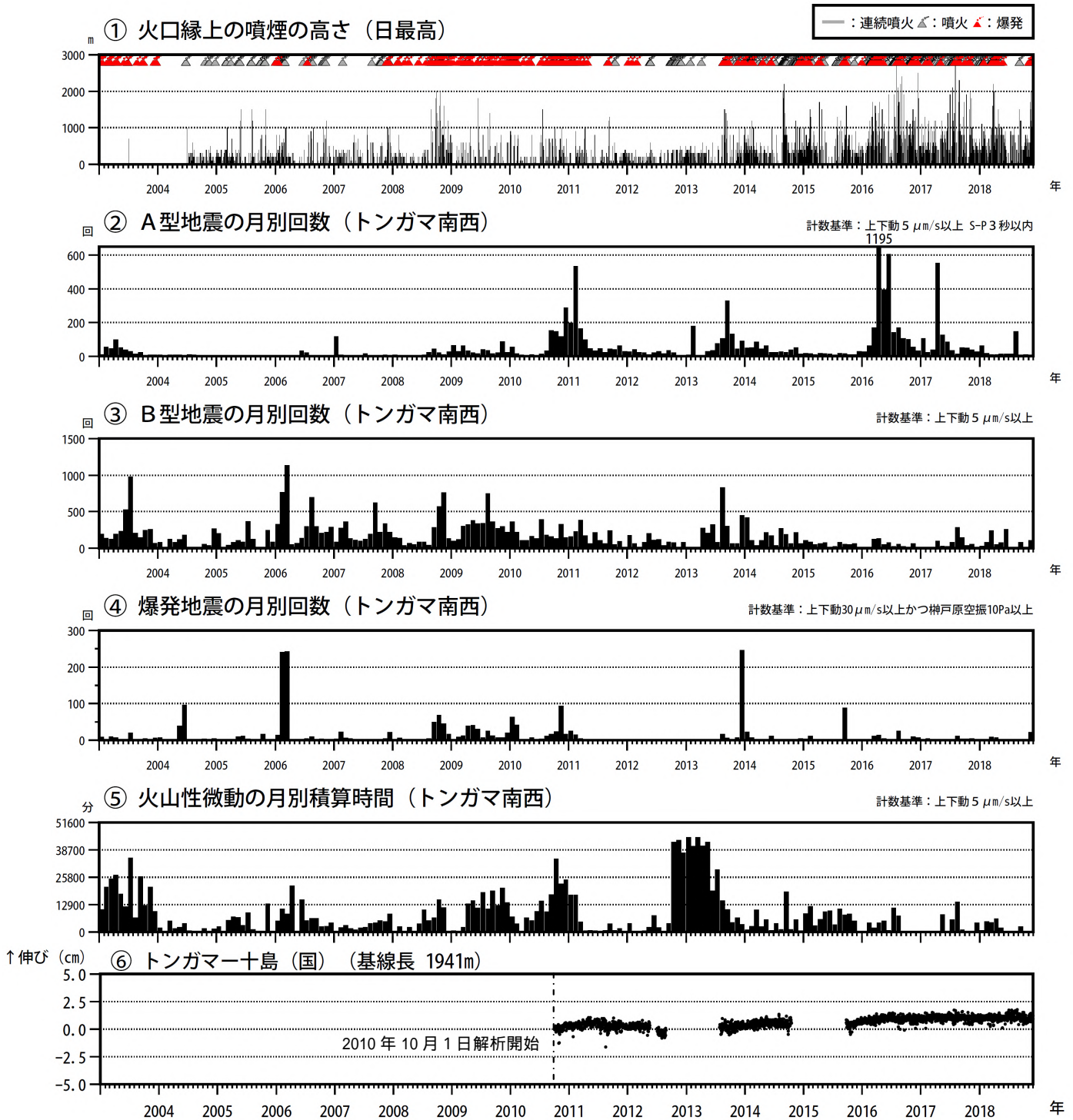
図3 諏訪之瀬島 長期の火山活動経過図（2003年1月～2018年11月）
