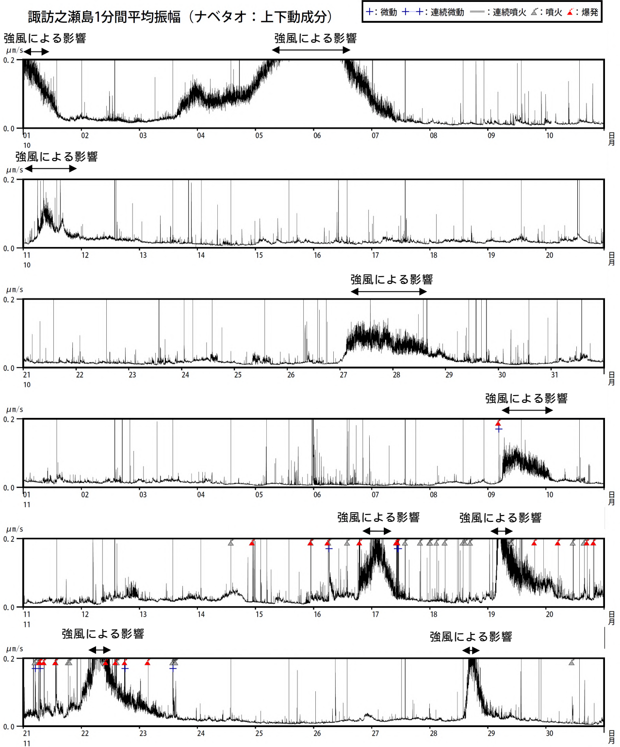
図5 諏訪之瀬島 1分間平均振幅の時間変化（ナベタオ観測点上下動成分、2018年10月～11月）
