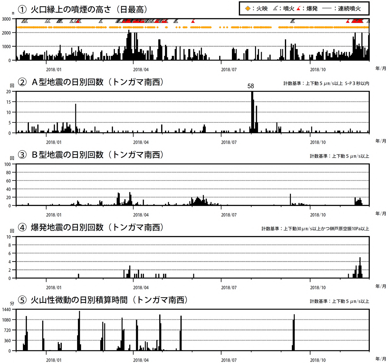
図 4 諏訪之瀬島 最近の火山活動経過図（2017 年 12 月～2018 年 11 月）
