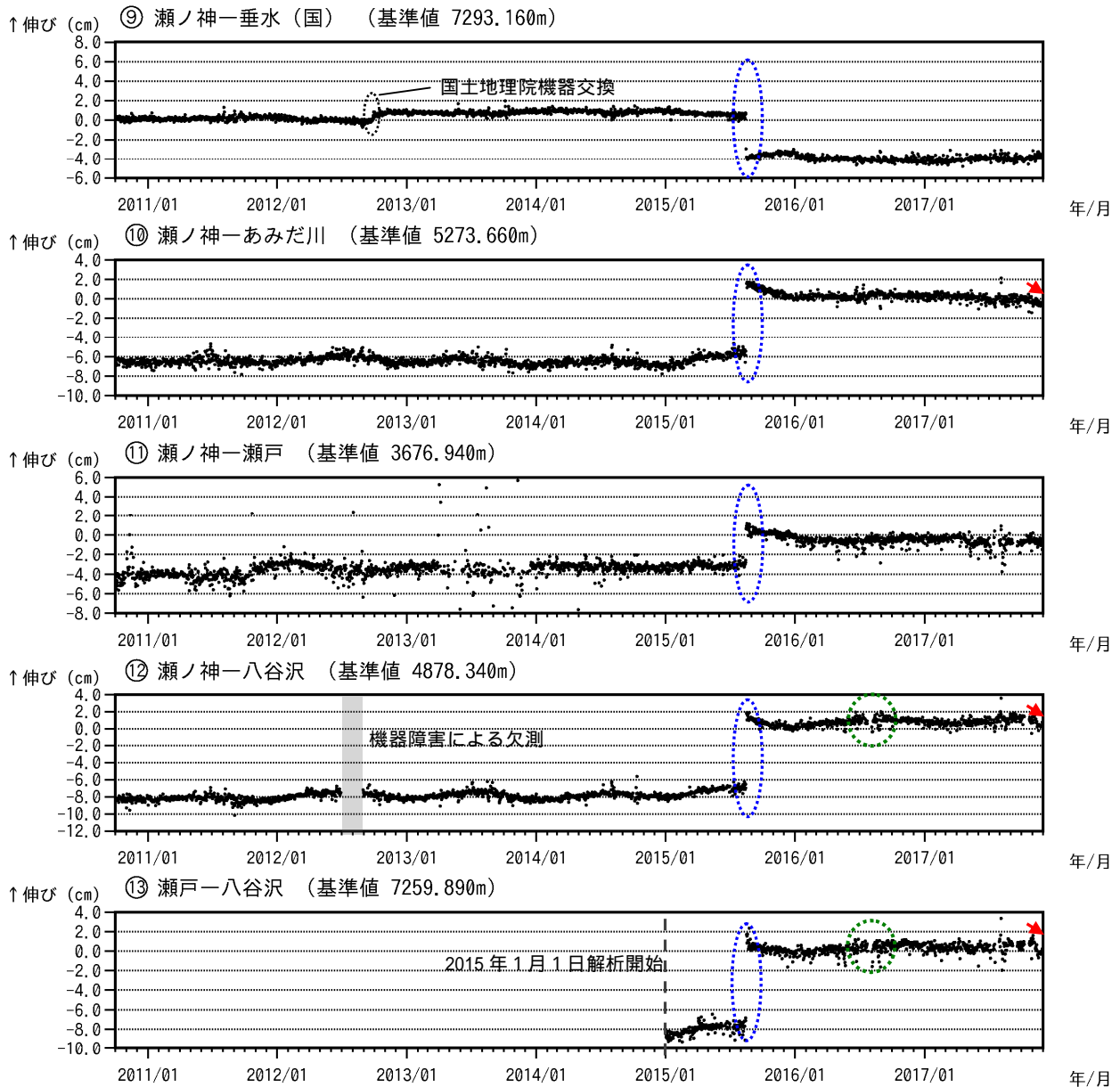
図 9-3 桜島 GNSS 連続観測による基線長変化（2010 年 10 月～2017 年 11 月）
