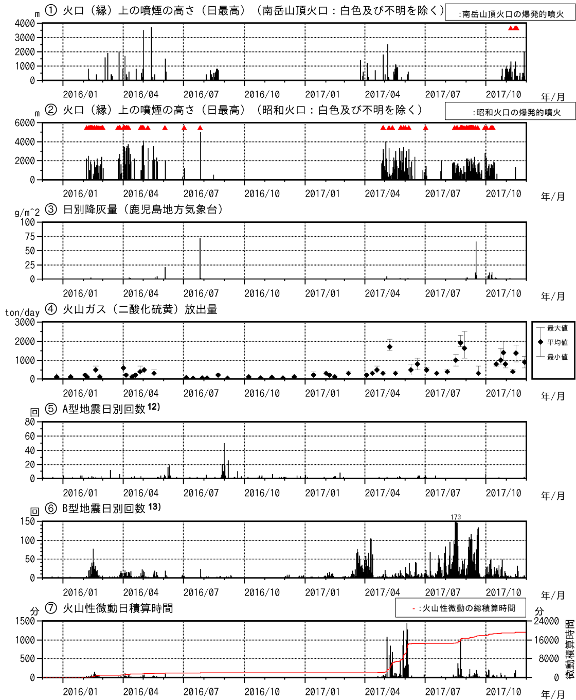
図5 桜島 最近2年間の活動経過図（2015年12月～2017年11月）
