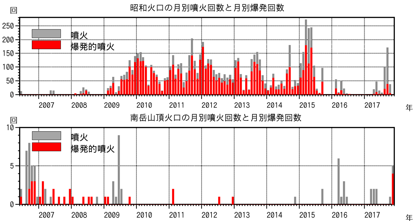
図4 桜島 昭和火口（上図）と南岳山頂火口（下図）の月別噴火回数と月別爆発回数 （2006年6月～2017年11月）
