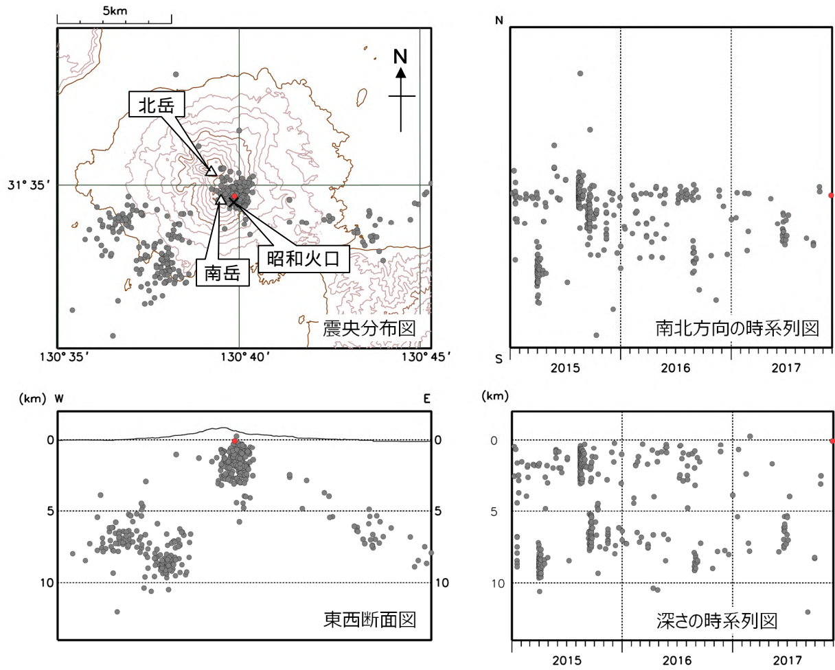
図 7 桜島 火山性地震の震源分布図（2015 年 1 月～2017 年 11 月）
