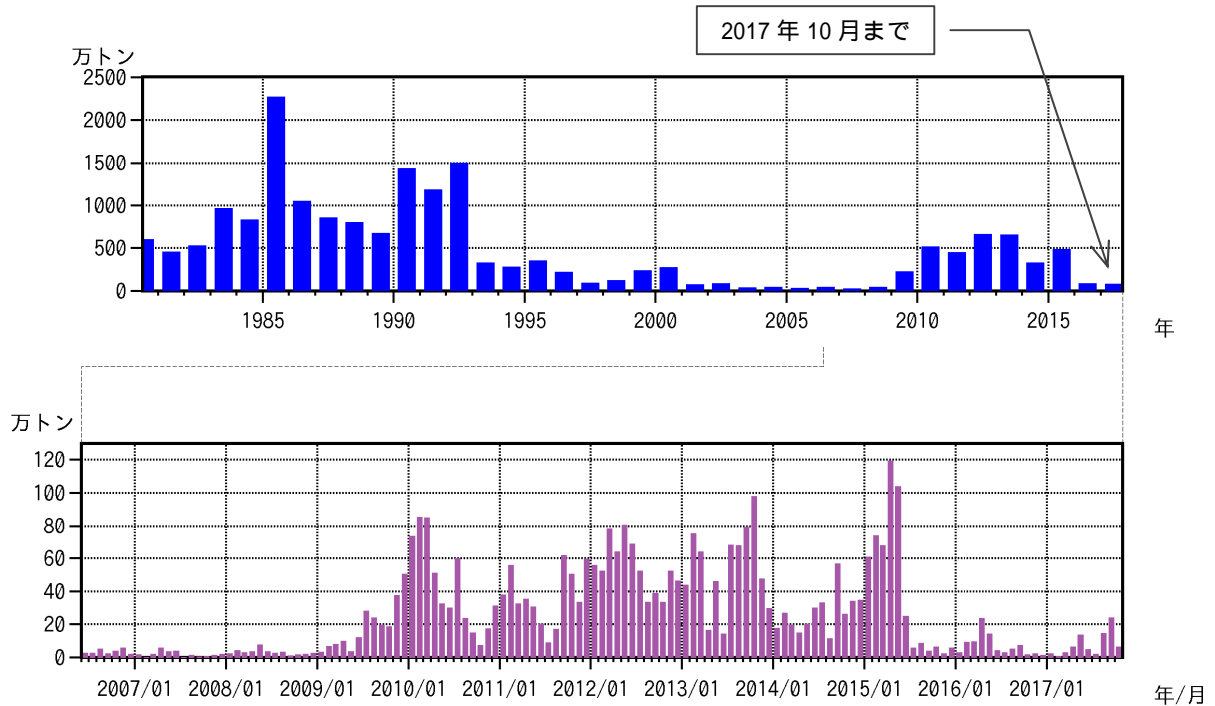
図 11 桜島 鹿児島県が実施している降灰の観測データから推定した火山灰の総噴出量（上段：1980 年 1 月～2017 年 10 月の年別値、下段：2006 年 6 月～2017 年 10 月の月別値）
