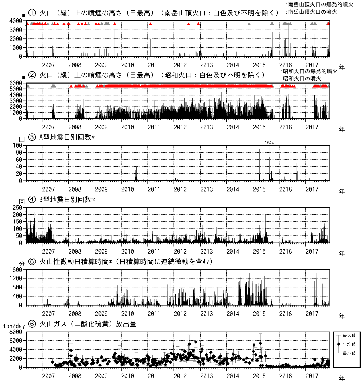
図6 桜島 昭和火口噴火活動再開（2006年6月）以降の活動経過図 （2006年6月～2017年11月）
