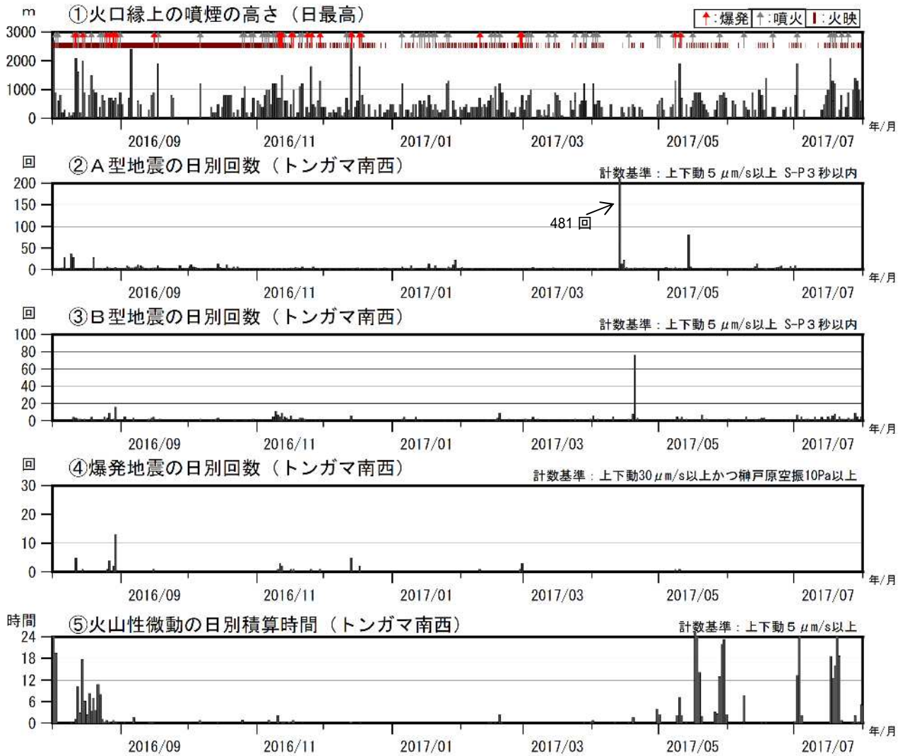
図3 諏訪之瀬島 最近の火山活動経過図（2016年8月～2017年7月）
