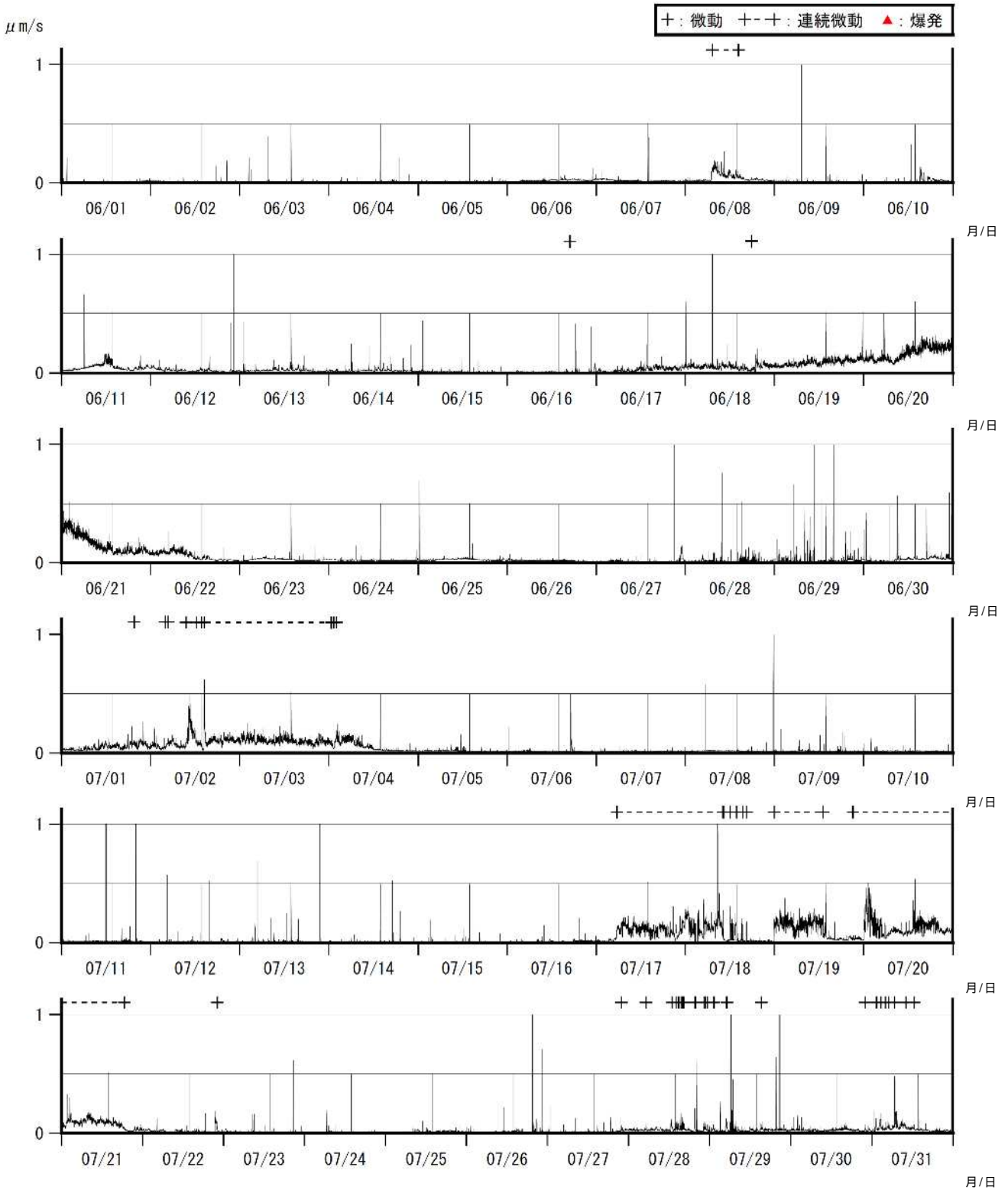
図4 諏訪之瀬島 1分間平均振幅の時間変化（ナベタオ観測点上下動成分、2017年6月～7月）
