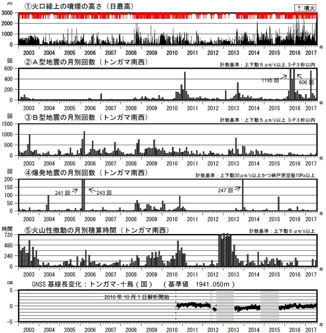
図2 諏訪之瀬島 長期の火山活動経過図（2003年1月～2017年7月）
