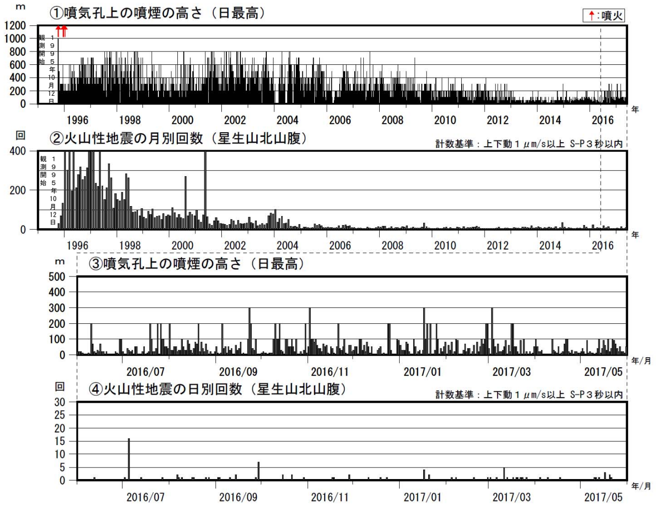
図4 九重山 火山活動経過図（1995年10月～2017年5月）
