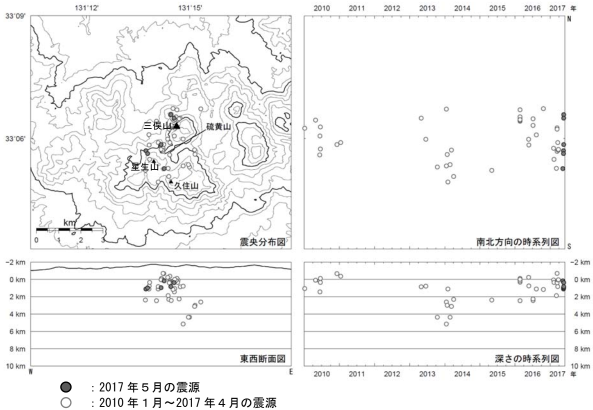
図3 九重山 震源分布図（2010年1月～2017年5月）
