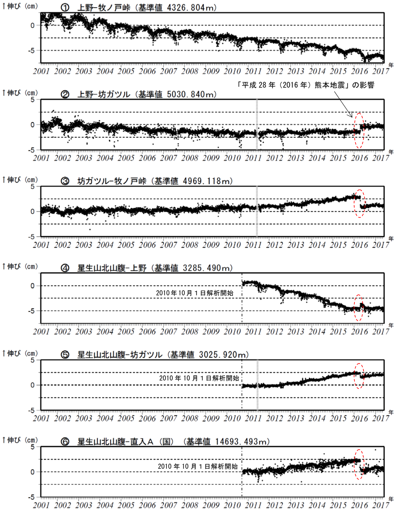
図5 九重山 GNSS 連続観測による基線長変化（2001 年 3 月～2017 年 5 月）
