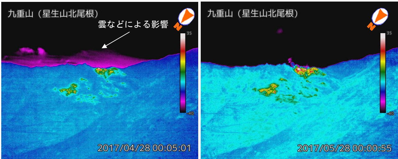
図2 九重山 赤外熱映像装置による地表面温度分布 (左：4月28日 右：5月28日、星生山北尾根監視カメラによる) 熱異常域の分布や最高温度に特段の変化は認められませんでした。
