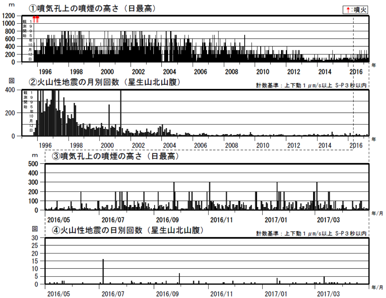
図3 九重山 火山活動経過図（1995年10月～2017年4月）
