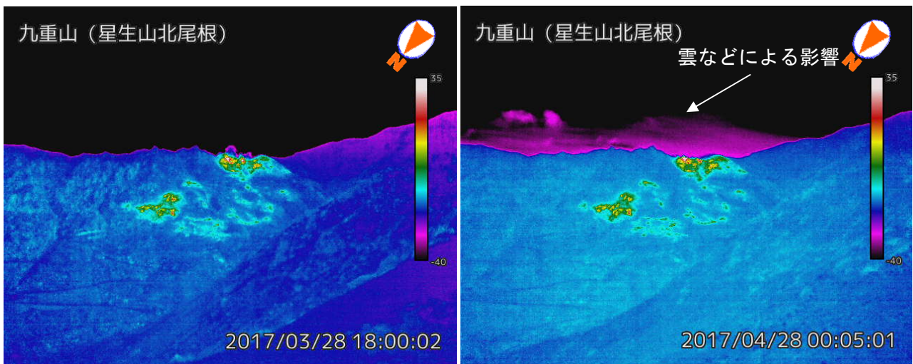
図2 九重山 赤外熱映像装置による地表面温度分布 （左：3月28日 右：4月28日、星生山北尾根監視カメラによる） 熱異常域の分布や最高温度に特段の変化は認められませんでした。
