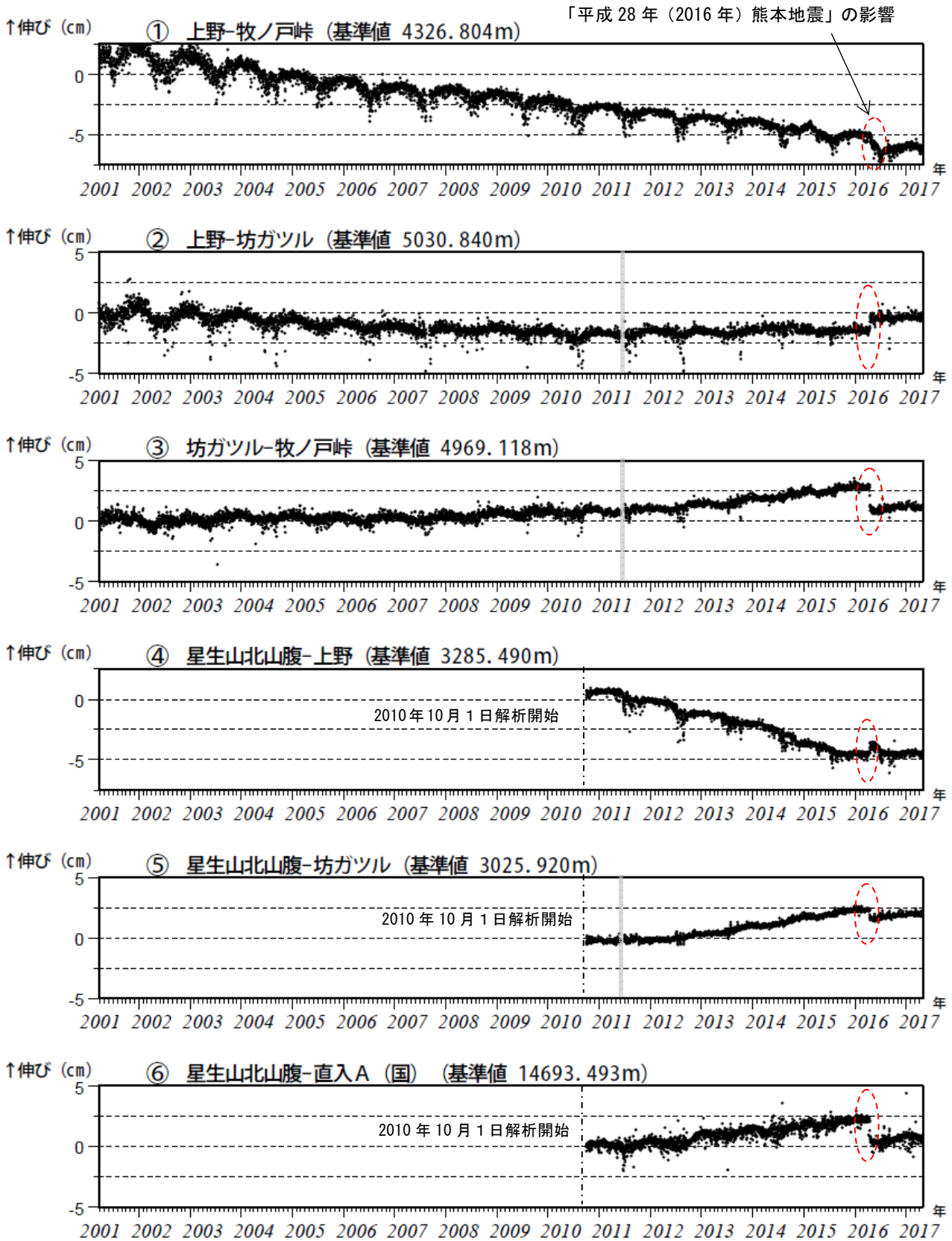
図 4 九重山 GNSS 連続観測による基線長変化（2001 年 3 月～2017 年 4 月）
