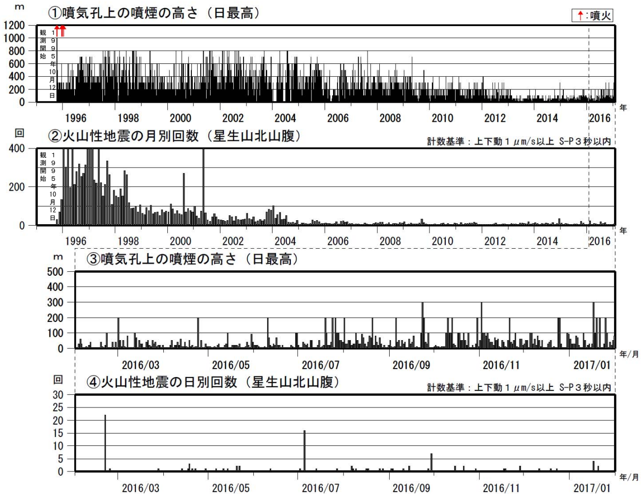
図2 九重山 火山活動経過図（1995 年 10 月～2017 年 1 月）
