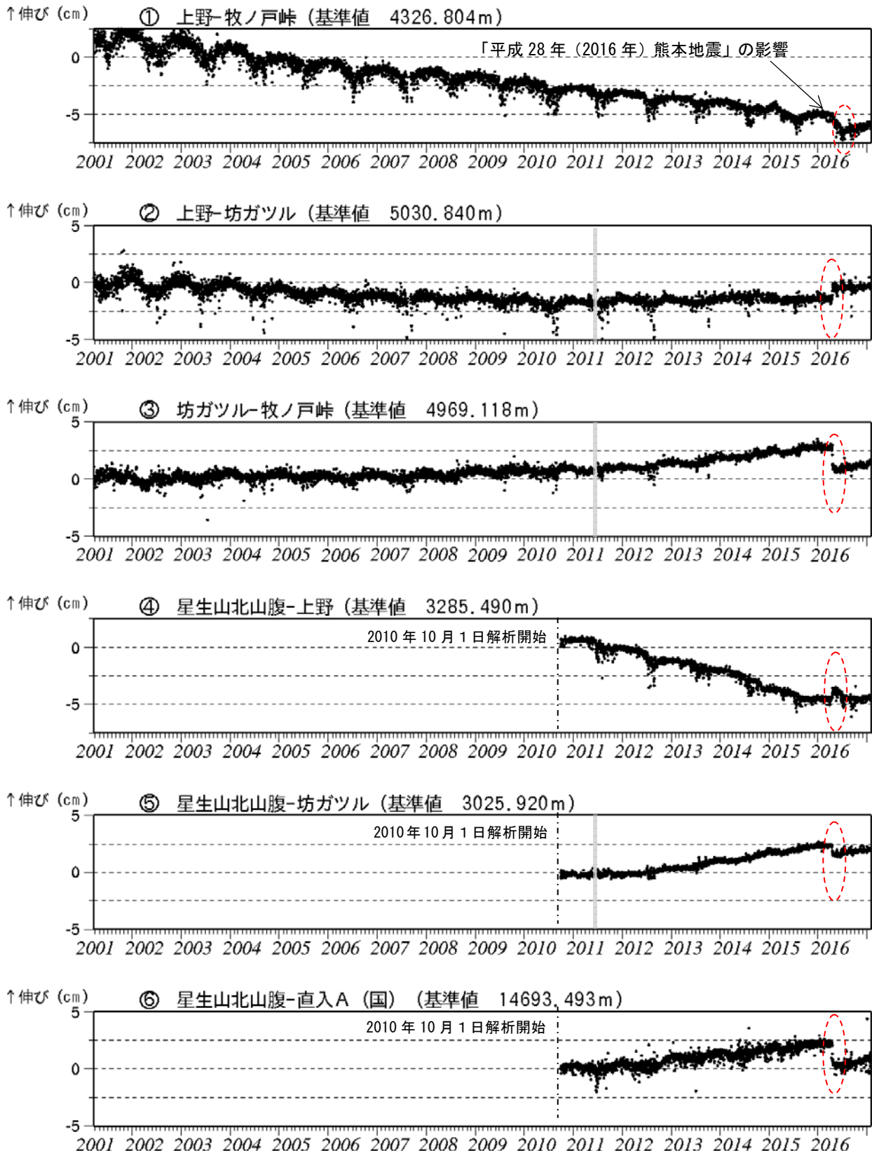
図 4 九重山 GNSS 連続観測による基線長変化 (2001 年 3 月～2017 年 1 月)
