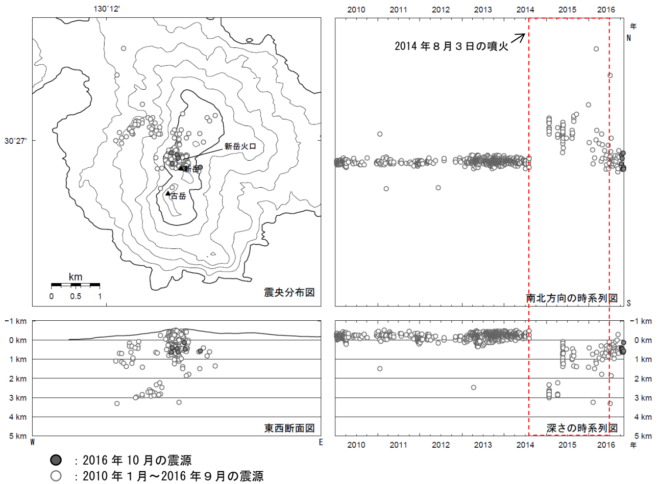
図 5 口永良部島 震源分布図（2010 年 1 月～2016 年 10 月）
