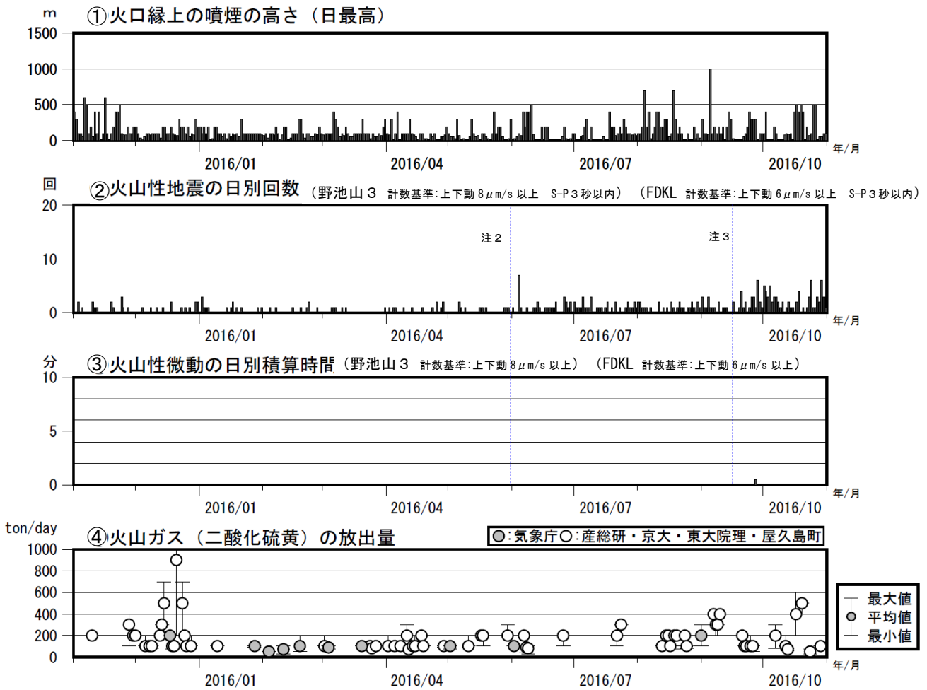
図4 口永良部島 最近の火山活動経過図（2015年11月～2016年10月）
