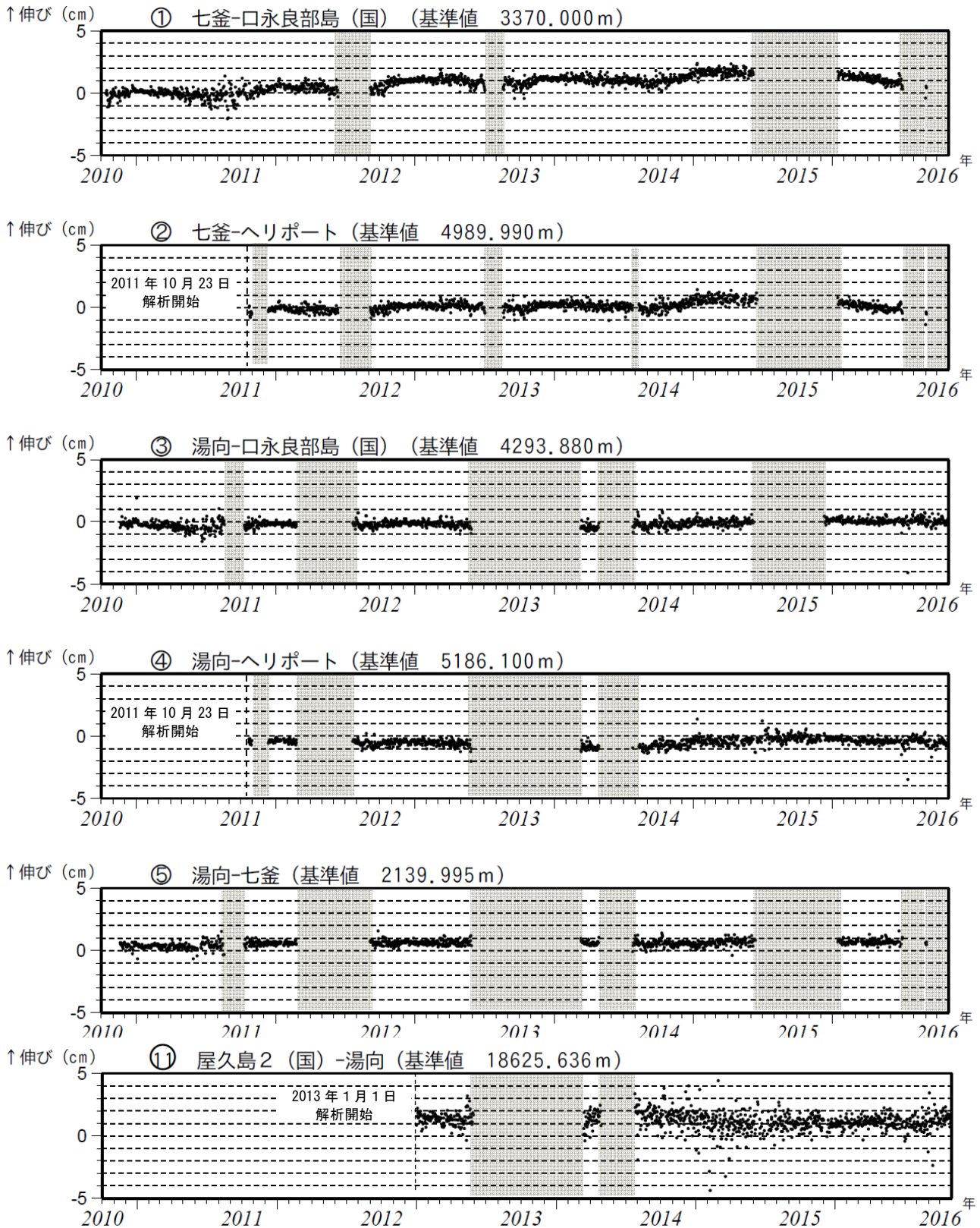
図6 口永良部島 GNSS 連続観測による基線長変化 (2010年10月~2016年10月)
