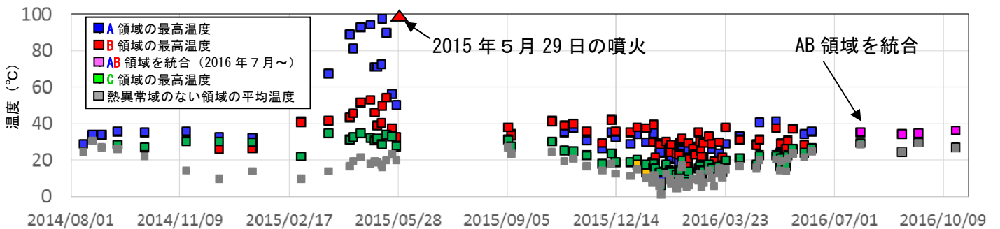
図2 口永良部島 新岳西斜面の地表面温度分布と熱異常域の温度時系列 (2014年8月～2016年10月：本村から新岳の北西側を撮影)
