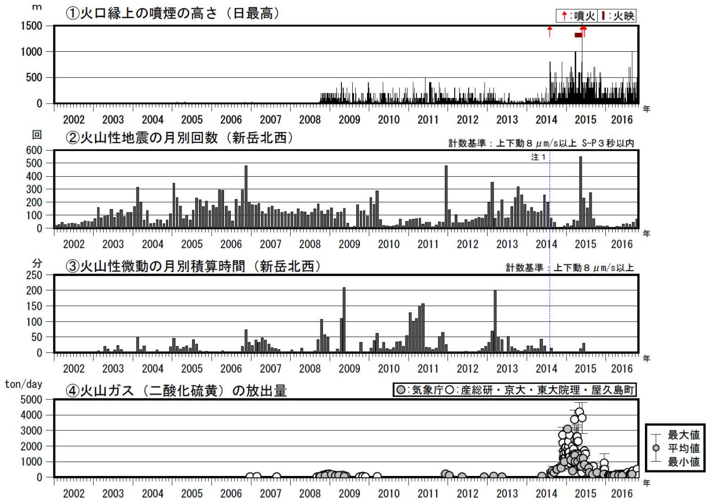
図3 口永良部島 火山活動経過図（2002年1月～2016年10月）
