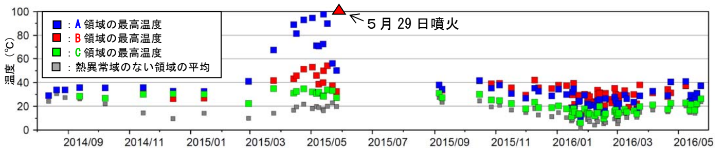
図4 口永良部島 新岳西斜面の地表面温度分布と熱異常域の温度時系列 （本村から新岳の北西側を撮影、2014年8月～2016年5月）
