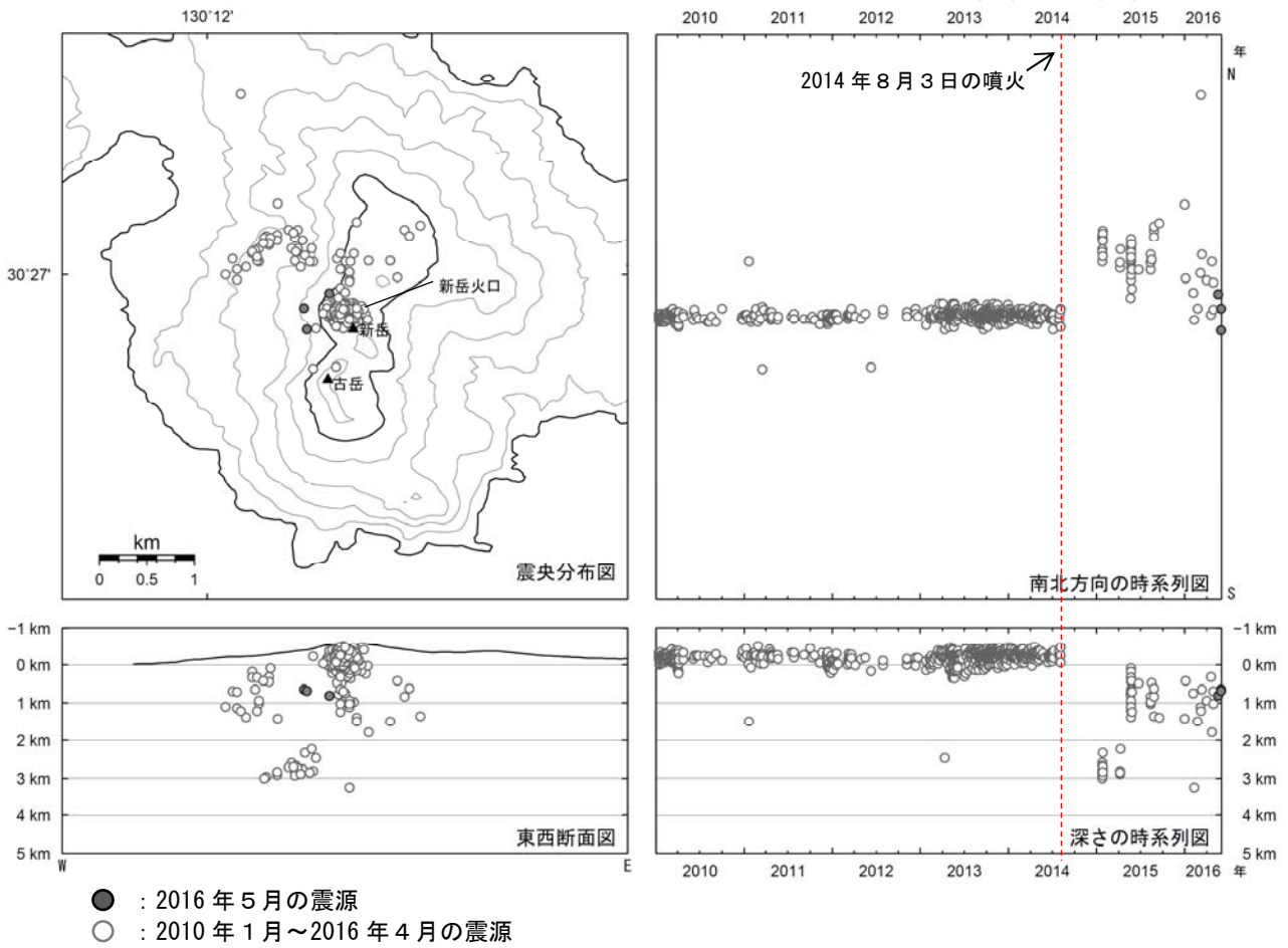
図 6 口永良部島 震源分布図（2010 年 1 月～2016 年 5 月）
