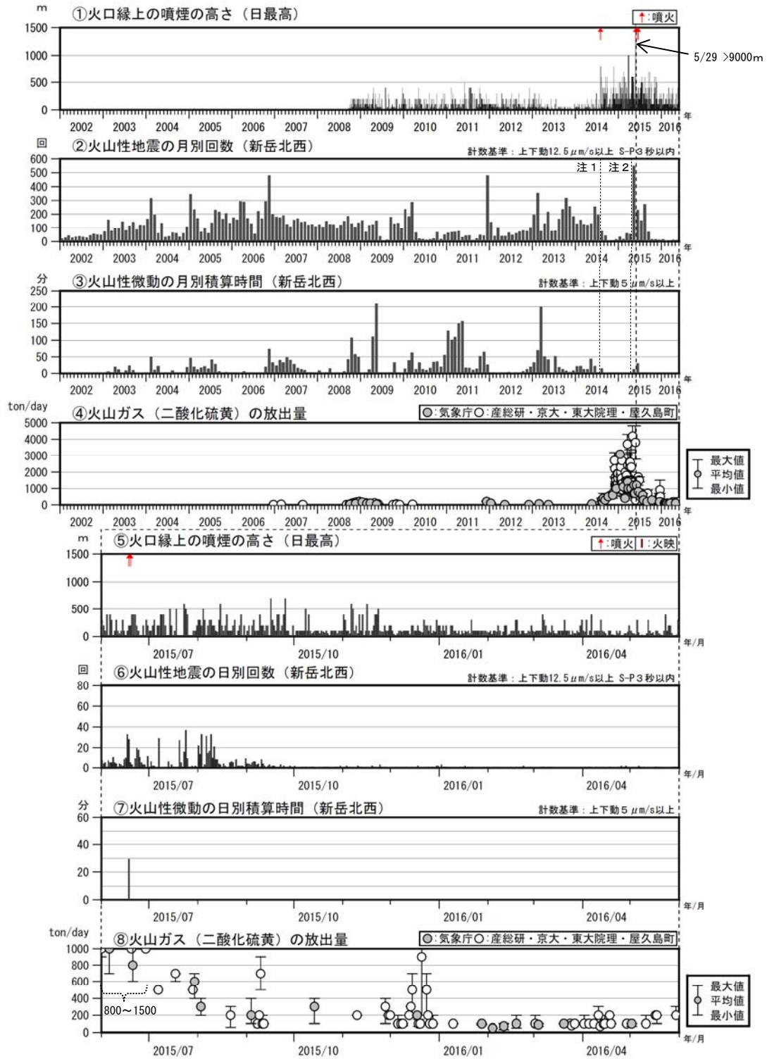
図5 口永良部島 火山活動経過図（2002年1月～2016年5月）
