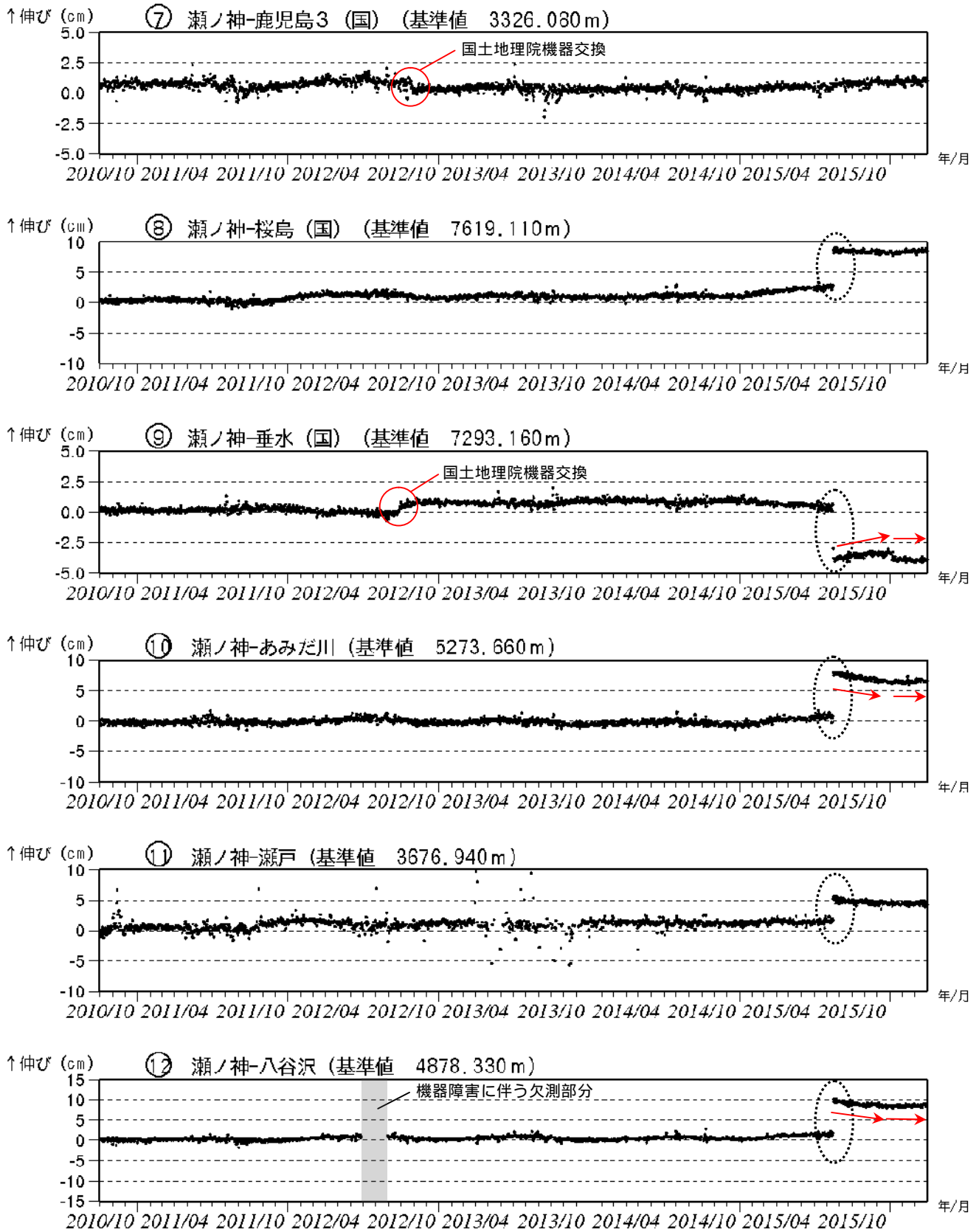
図 13-2 桜島 GNSS 連続観測による基線長変化 (2010年10月~2016年3月)
