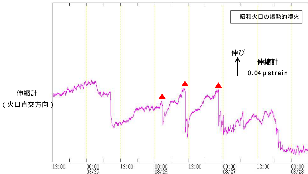
図 12 桜島 爆発的噴火に伴う有村観測坑道伸縮計（火口直交成分）の変動 （2016 年 3 月 24 日 12 時～3 月 28 日 06 時）
