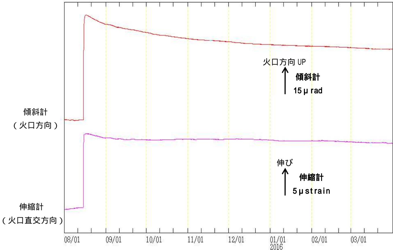
図 11 桜島 有村観測坑道の傾斜計及び伸縮計の変化（2015 年 8 月 1 日～2016 年 3 月 31 日） 2015 年 8 月の急激な変動以降、山体膨張を示す規模の大きな地殻変動はみられていません。
