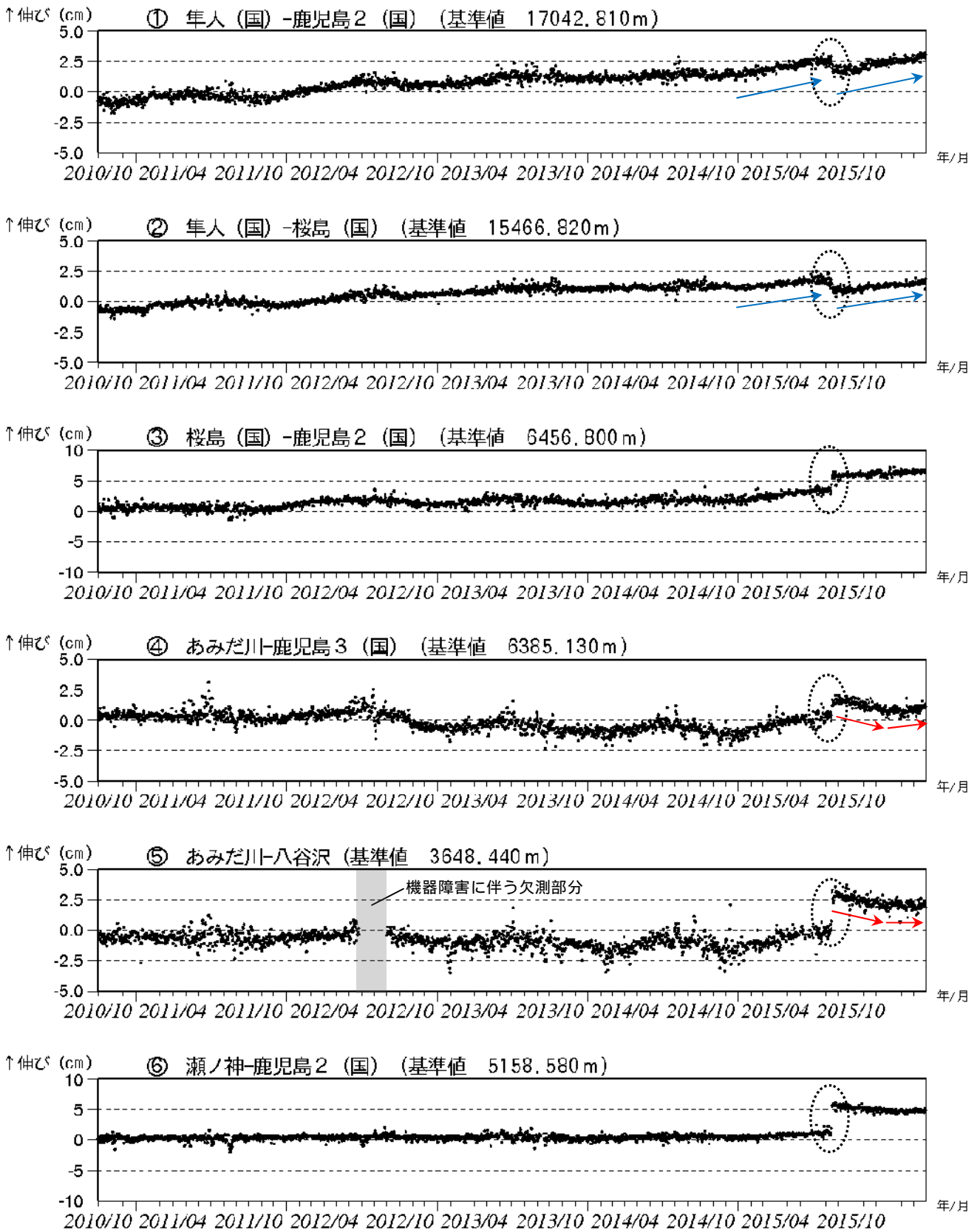
図 13-1 桜島 GNSS 連続観測による基線長変化(2010 年 10 月~2016 年 3 月)
