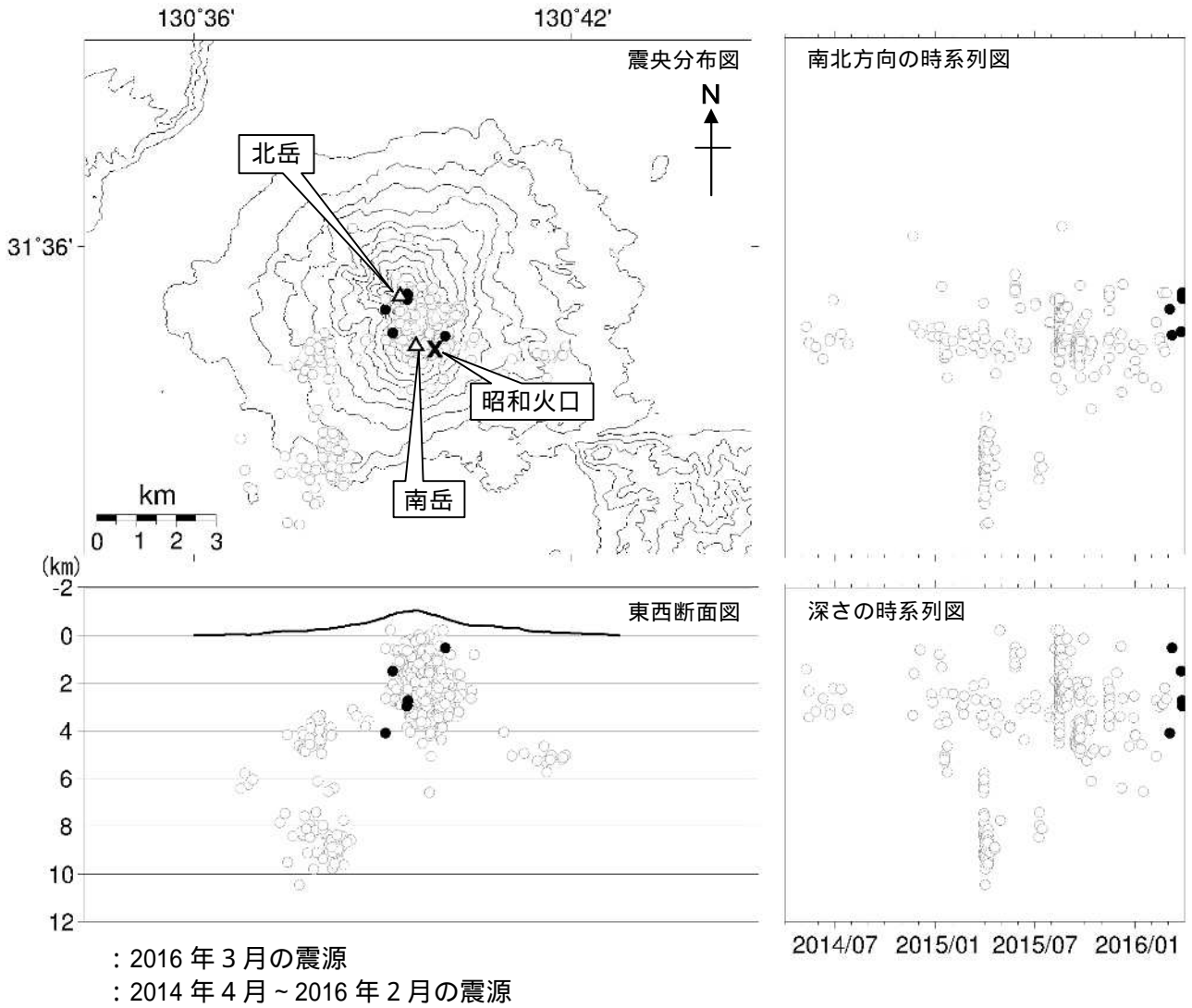
図 10 桜島 震源分布図 (2014 年 4 月 ~ 2016 年 3 月) < 3 月の状況 >
