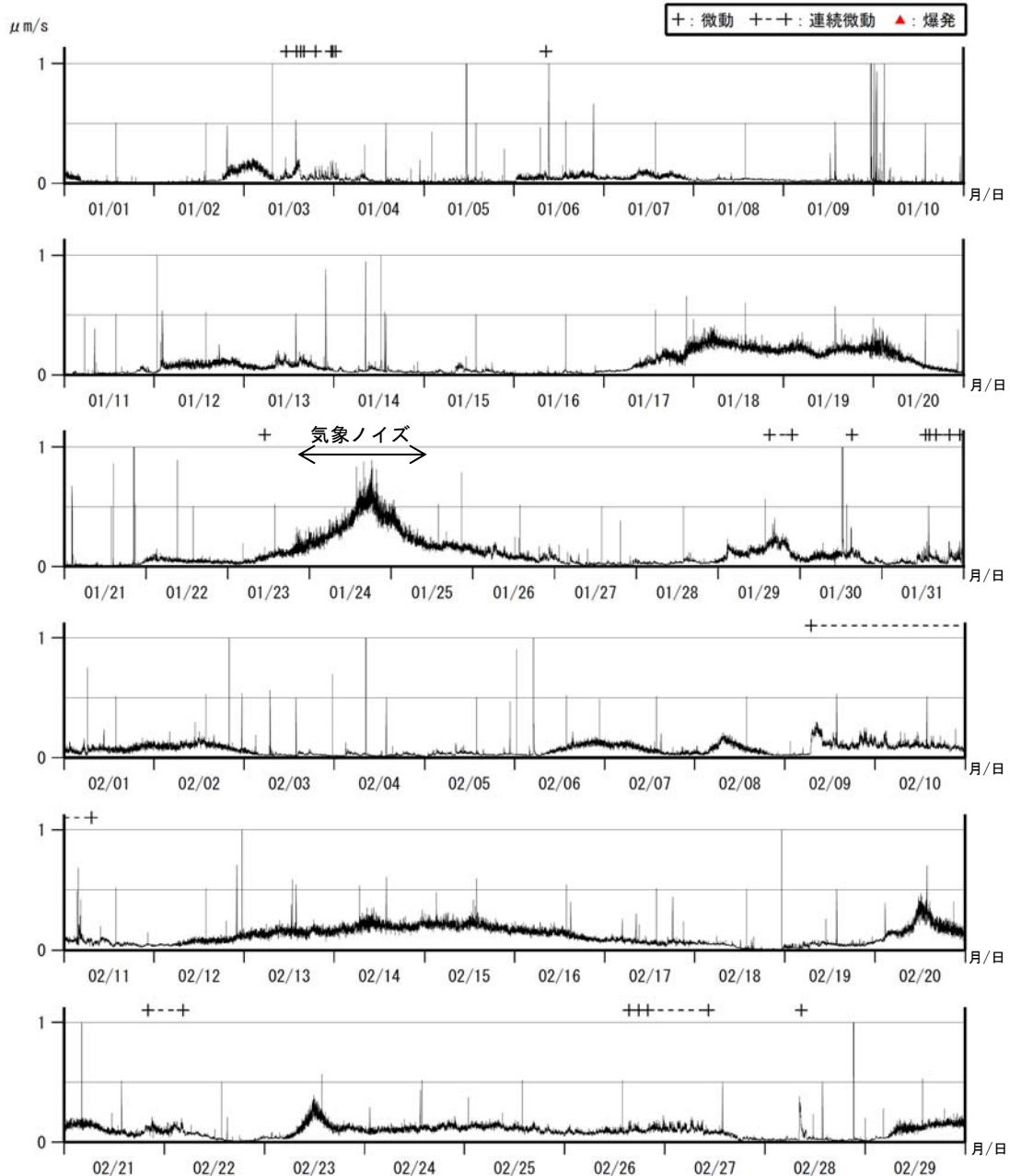
図 5 諏訪之瀬島 1 分間平均振幅の時間変化（ナベタオ観測点上下動成分、1 月～2 月）
