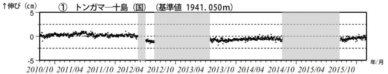
図 6 諏訪之瀬島 GNSS 連続観測による基線長変化（2010 年 10 月～2016 年 2 月）
