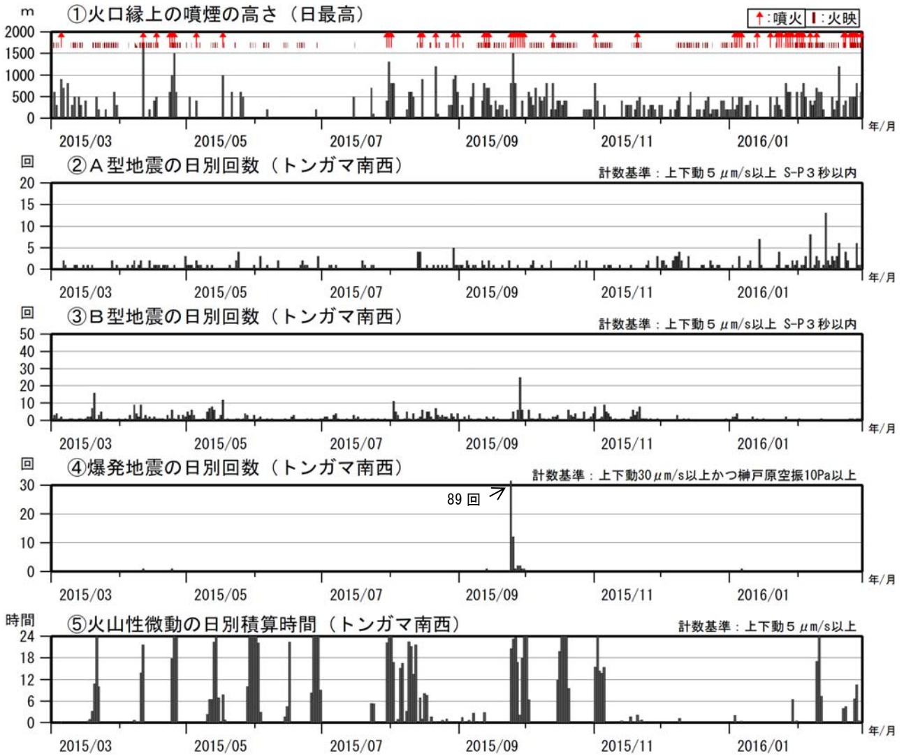
図4 諏訪之瀬島 最近の火山活動経過図（2015年3月～2016年2月）
