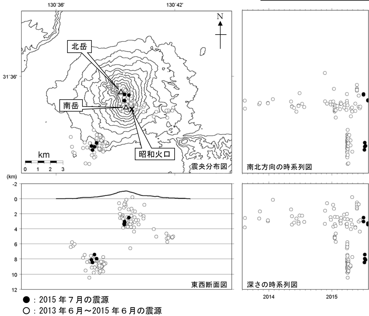
図 8 桜島 震源分布図 (2013 年 6 月～2015 年 7 月)
