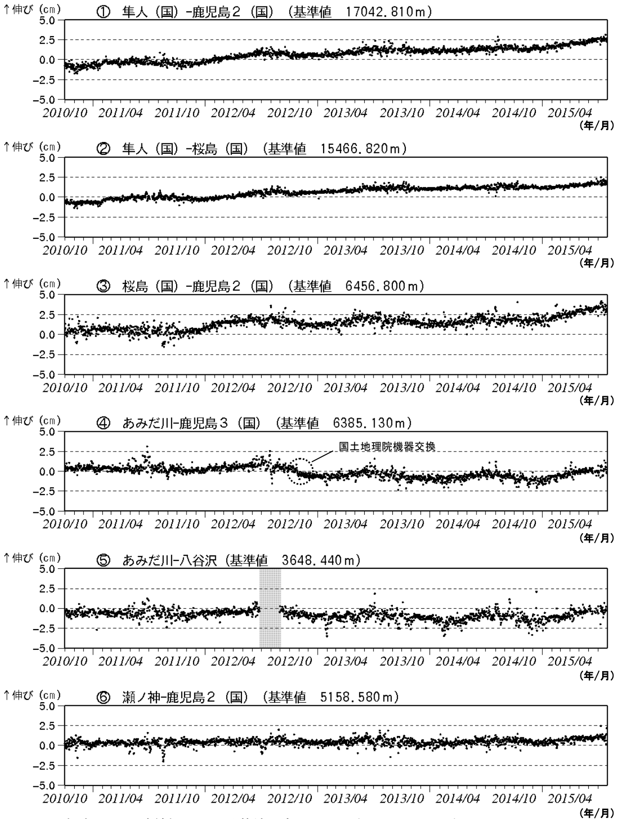
図 9-1 桜島 GNSS 連続観測による基線長変化 (2010 年 10 月～2015 年 7 月)
