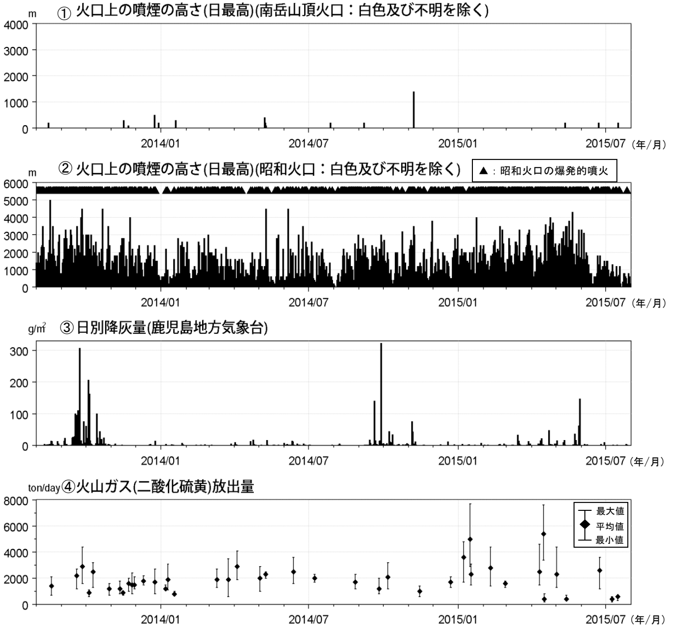
図5 桜島 最近2年間の噴煙、降灰、火山ガス（2013年8月～2015年7月）
