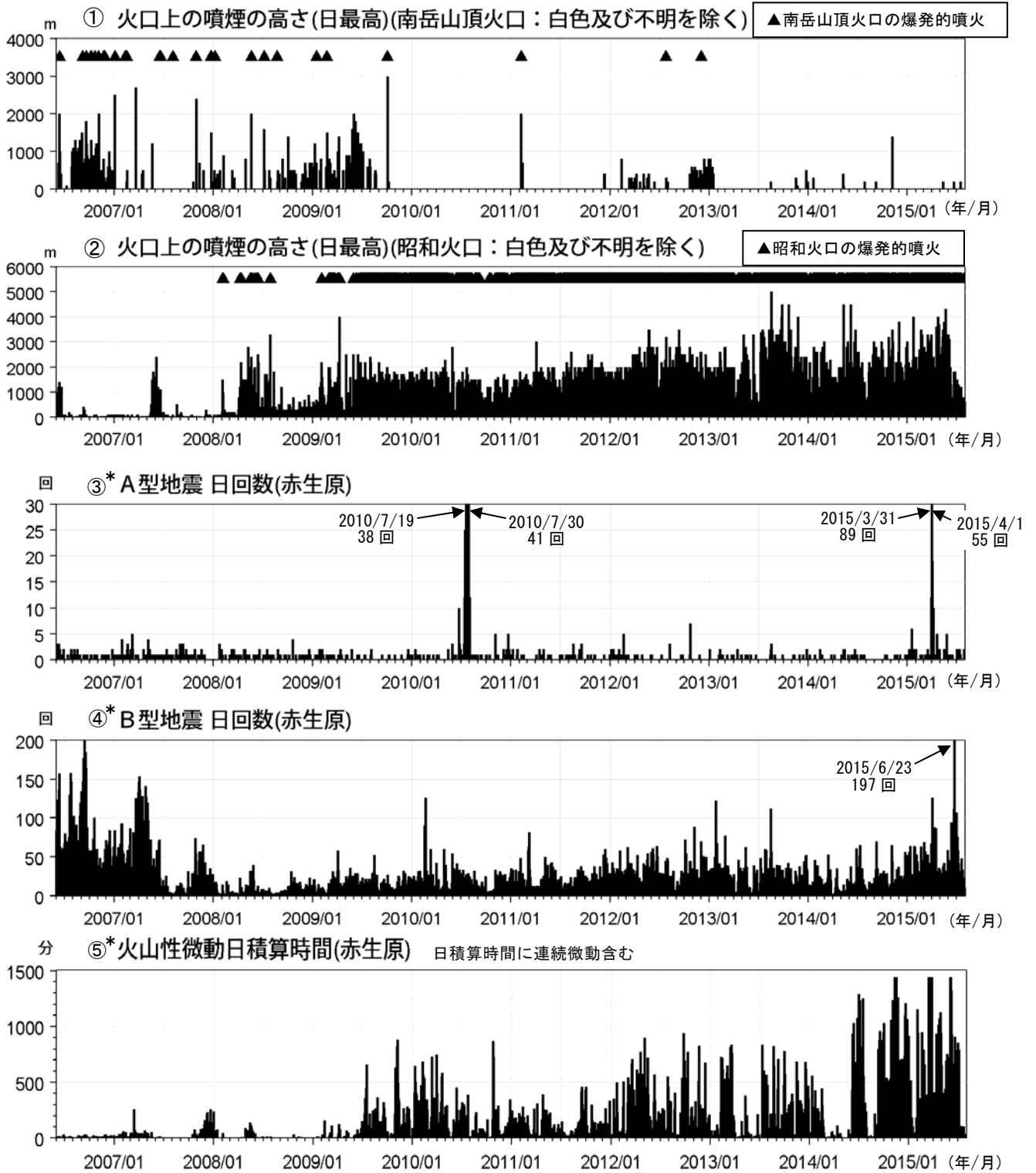
図7 桜島 昭和火口噴火活動再開（2006年6月）以降の爆発的噴火、噴煙、火山性地震の状況（2006年6月～2015年7月）
