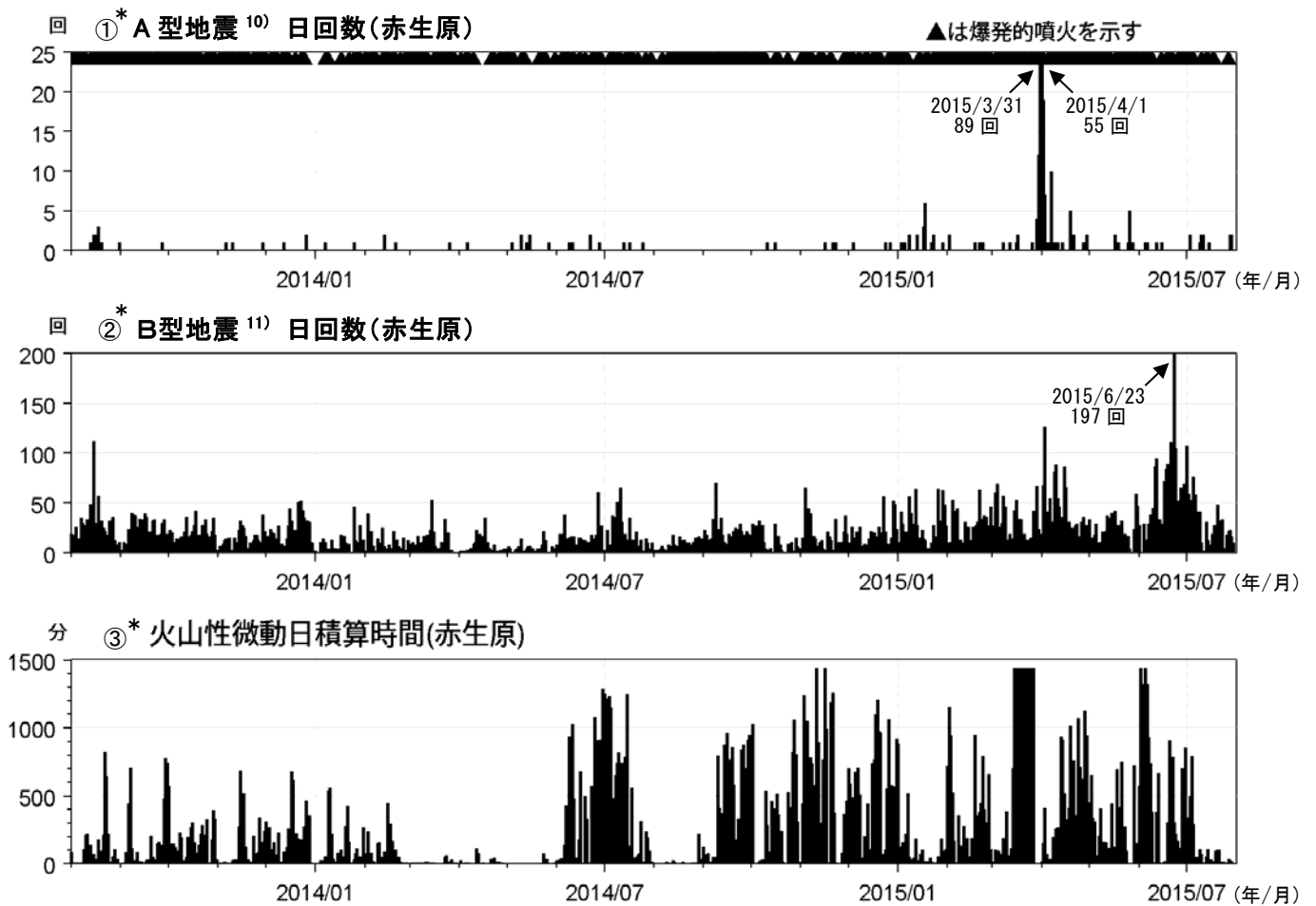
図6 桜島 最近2年間の火山性地震、火山性微動（2013年8月～2015年7月）
