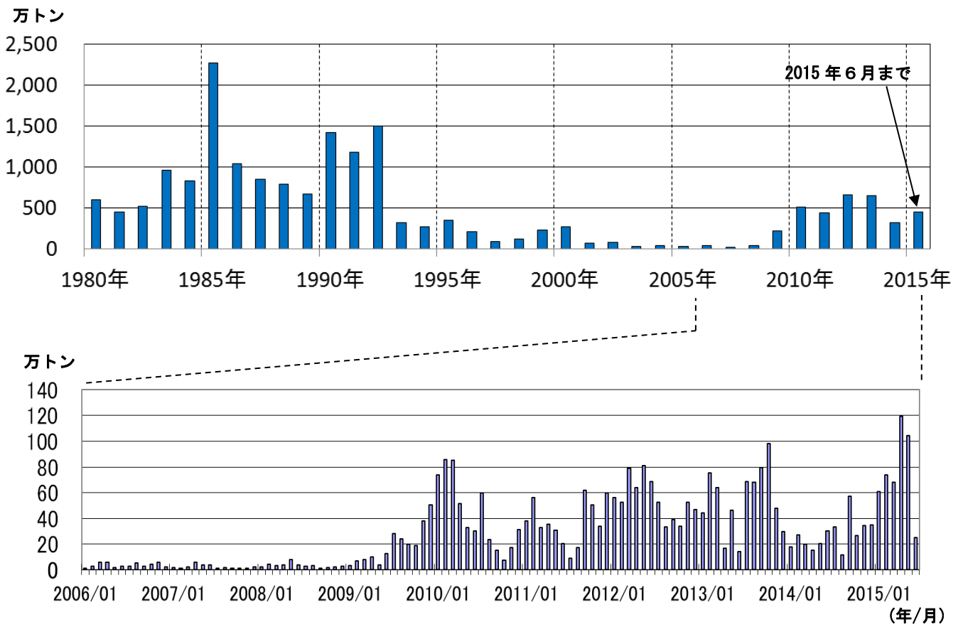
図4 桜島 鹿児島県が実施している降灰の観測データから推定した火山灰の総噴出量 （1980年1月～2015年6月、上段：年別値 下段：月別値）
