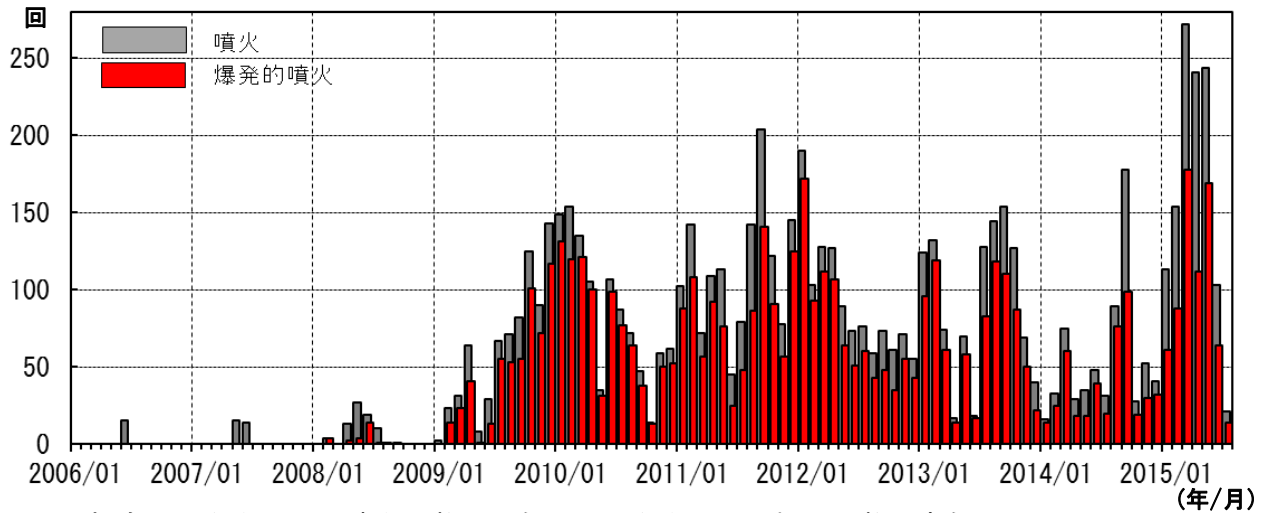
図3 桜島 昭和火口月別噴火回数（灰色）と昭和火口月別爆発回数（赤色） （2006年1月～2015年7月）
