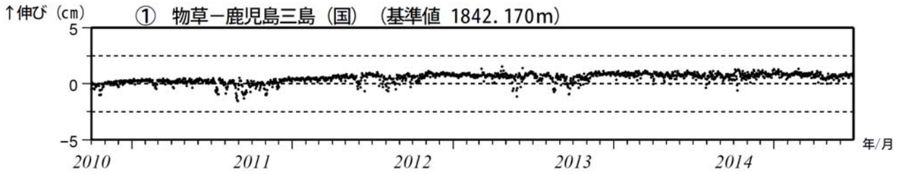
図 3 薩摩硫黄島 GNSS連続観測による基線長変化 (2010 年 10 月～2015 年 6 月)
