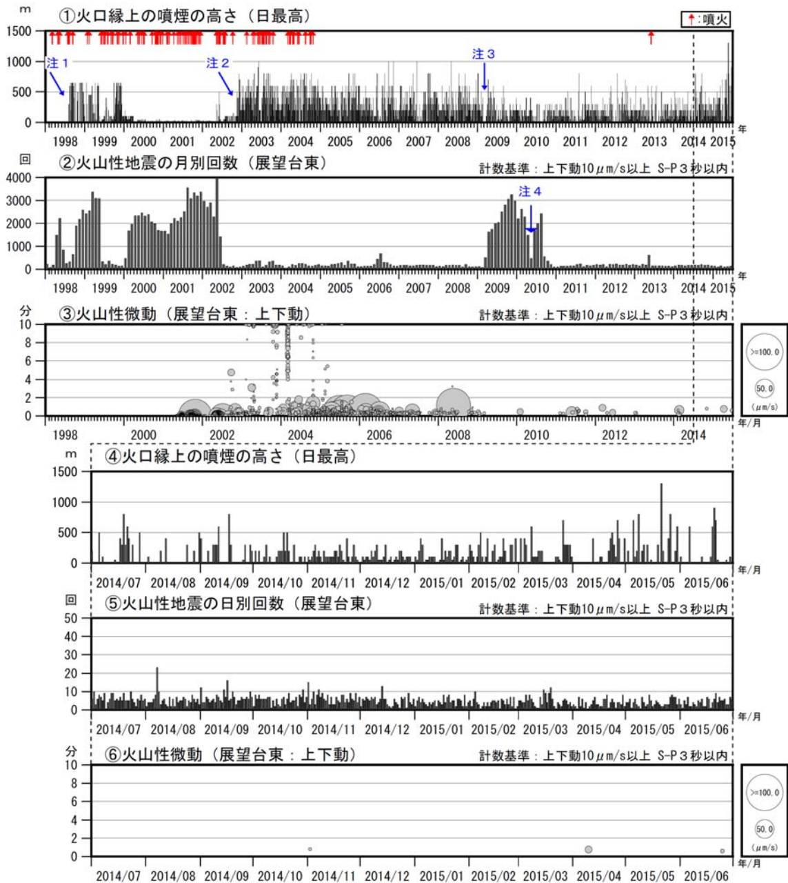
図 2 薩摩硫黄島 火山活動経過図（1998 年 1 月～2015 年 6 月）
