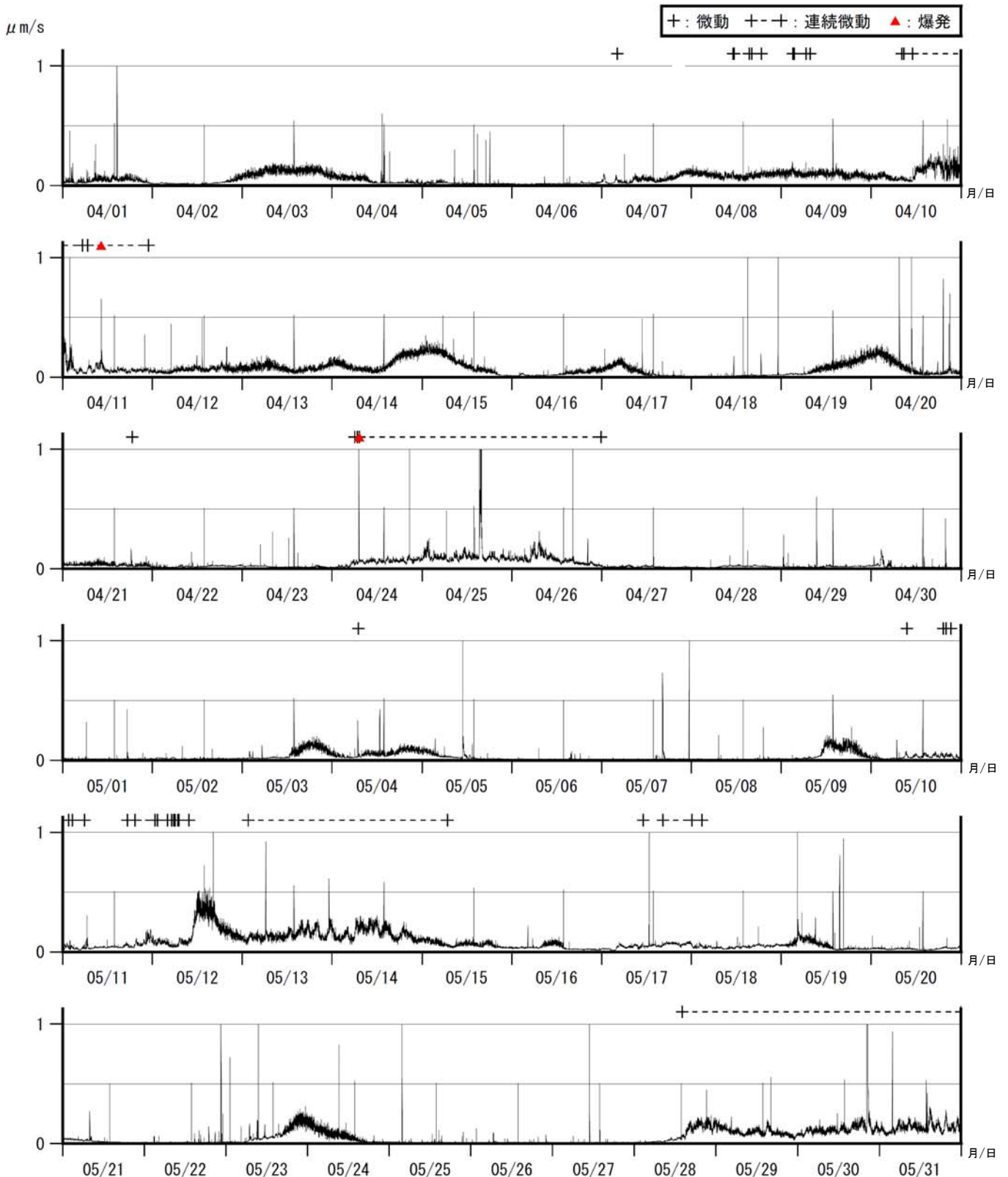
図 4 諏訪之瀬島 1 分間平均振幅の時間変化 （トンガマ南西観測点上下動成分）（2015 年 4 月～5 月）
