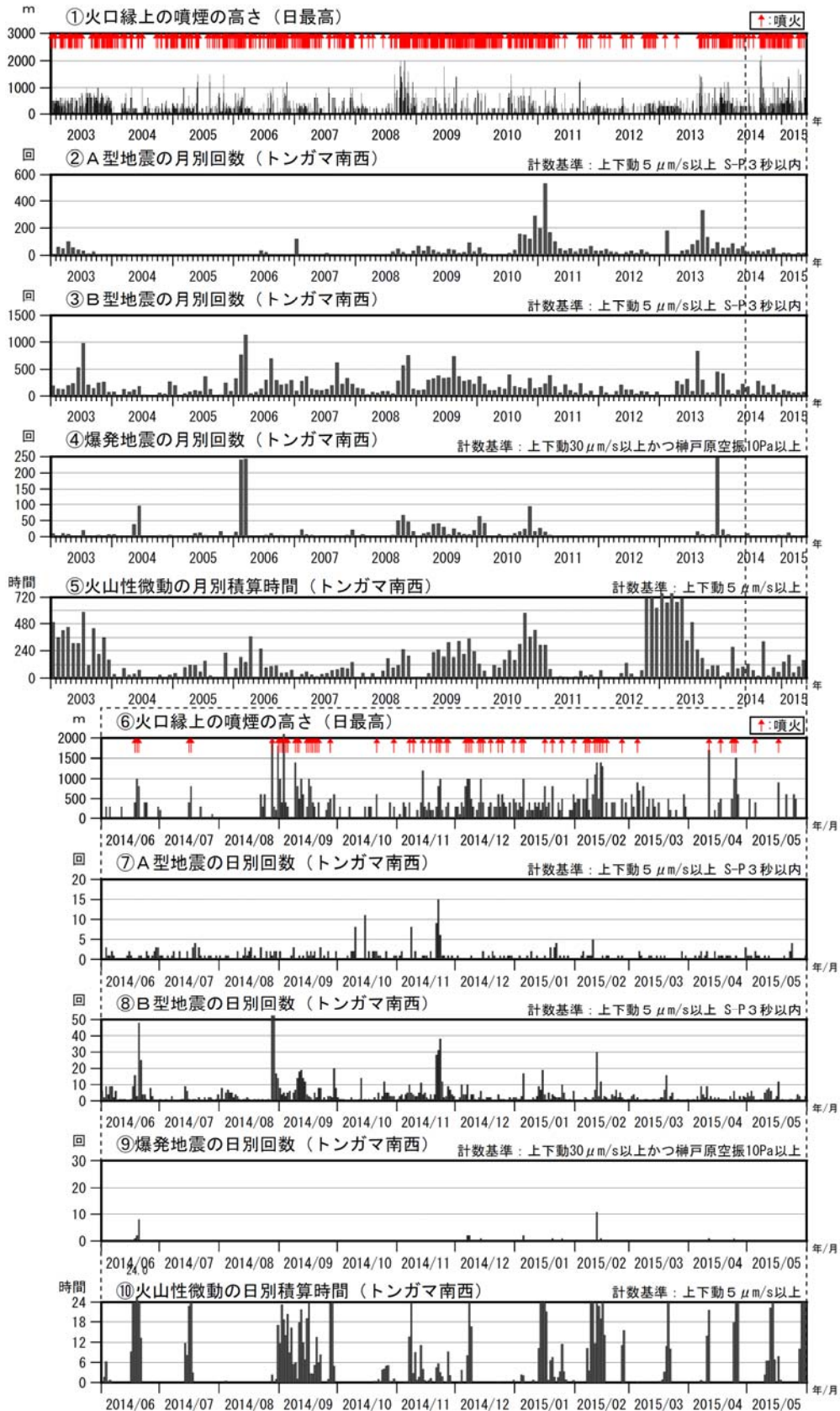
図3 諏訪之瀬島 火山活動経過図（2003年1月～2015年5月）
