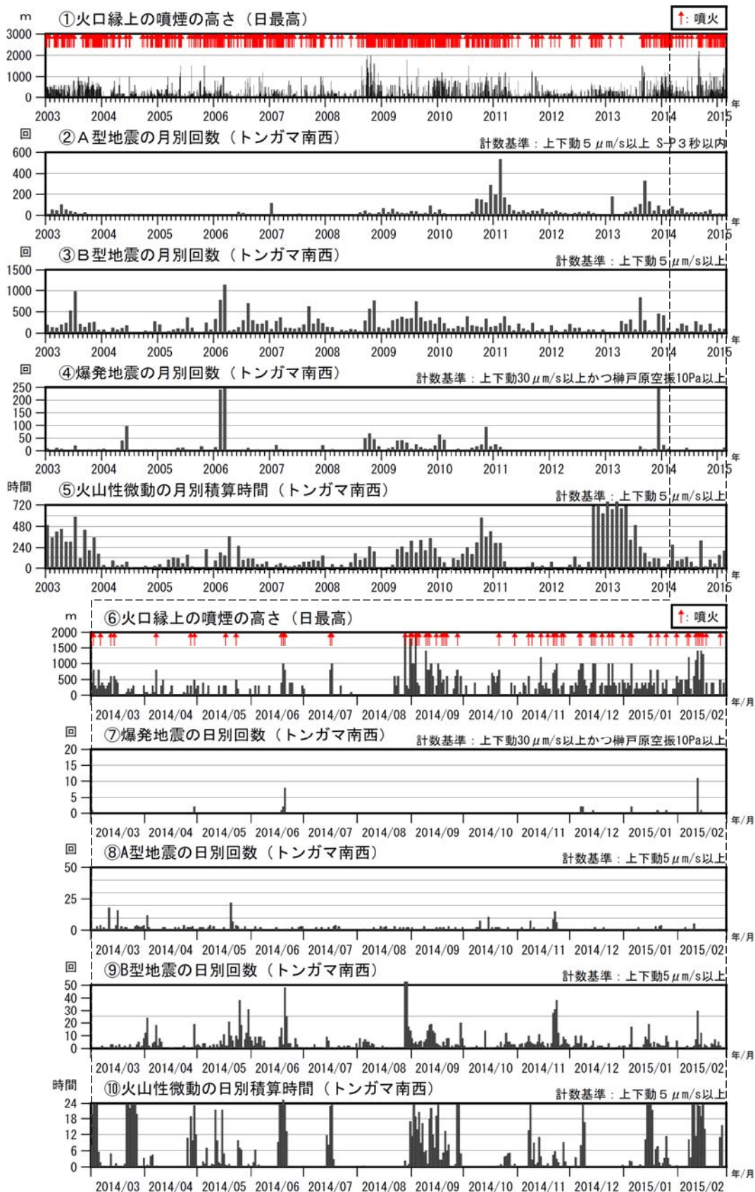
図3 諏訪之瀬島 火山活動経過図（2003年1月～2015年2月）
