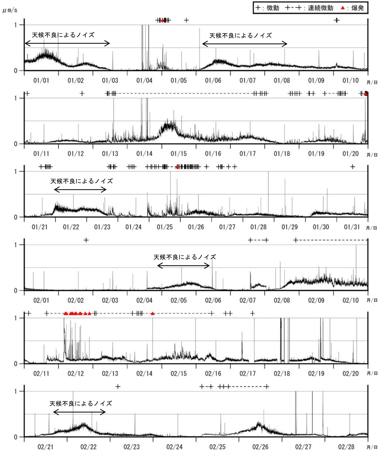
図4 諏訪之瀬島 1分間平均振幅の時間変化 (トンガマ南西観測点上下動成分) (2015年1月～2月)
