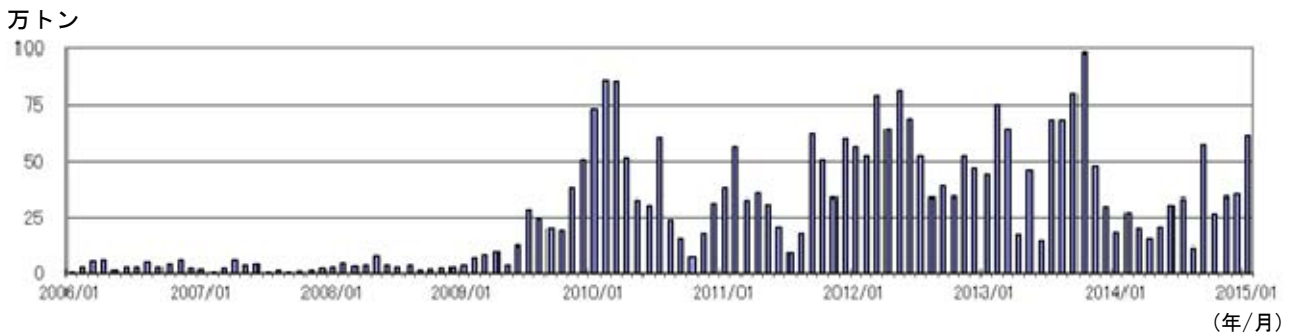
図4 桜島 鹿児島県が実施している降灰の観測データから推定した火山灰の月別総噴出量 （2006年1月～2015年1月）
