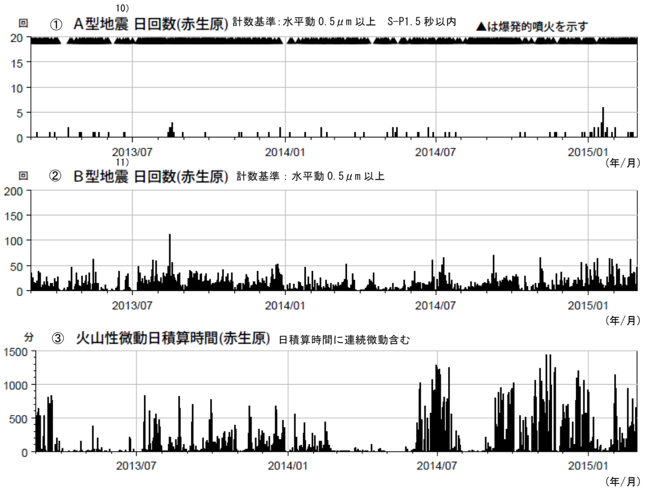
図7 桜島 最近2年間の火山性地震、火山性微動（2013年3月～2015年2月）
