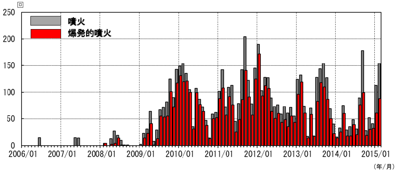
図3 桜島 昭和火口月別噴火回数（灰色）と昭和火口月別爆発回数（赤色） （2006年1月～2015年2月）
