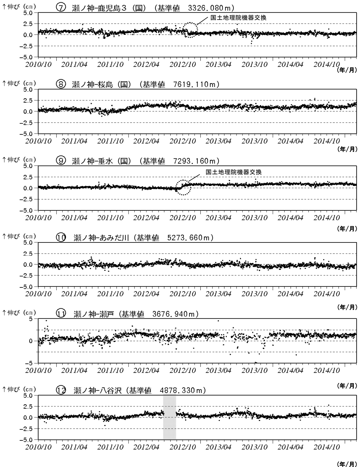
図 11-2 桜島 GNSS 連続観測による基線長変化 (2010 年 10 月～2015 年 2 月)
