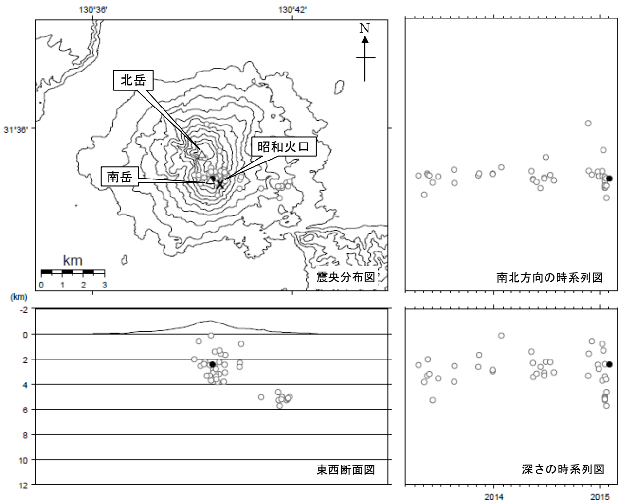
図 8 桜島 震源分布図（2013 年 3 月～2015 年 2 月）
