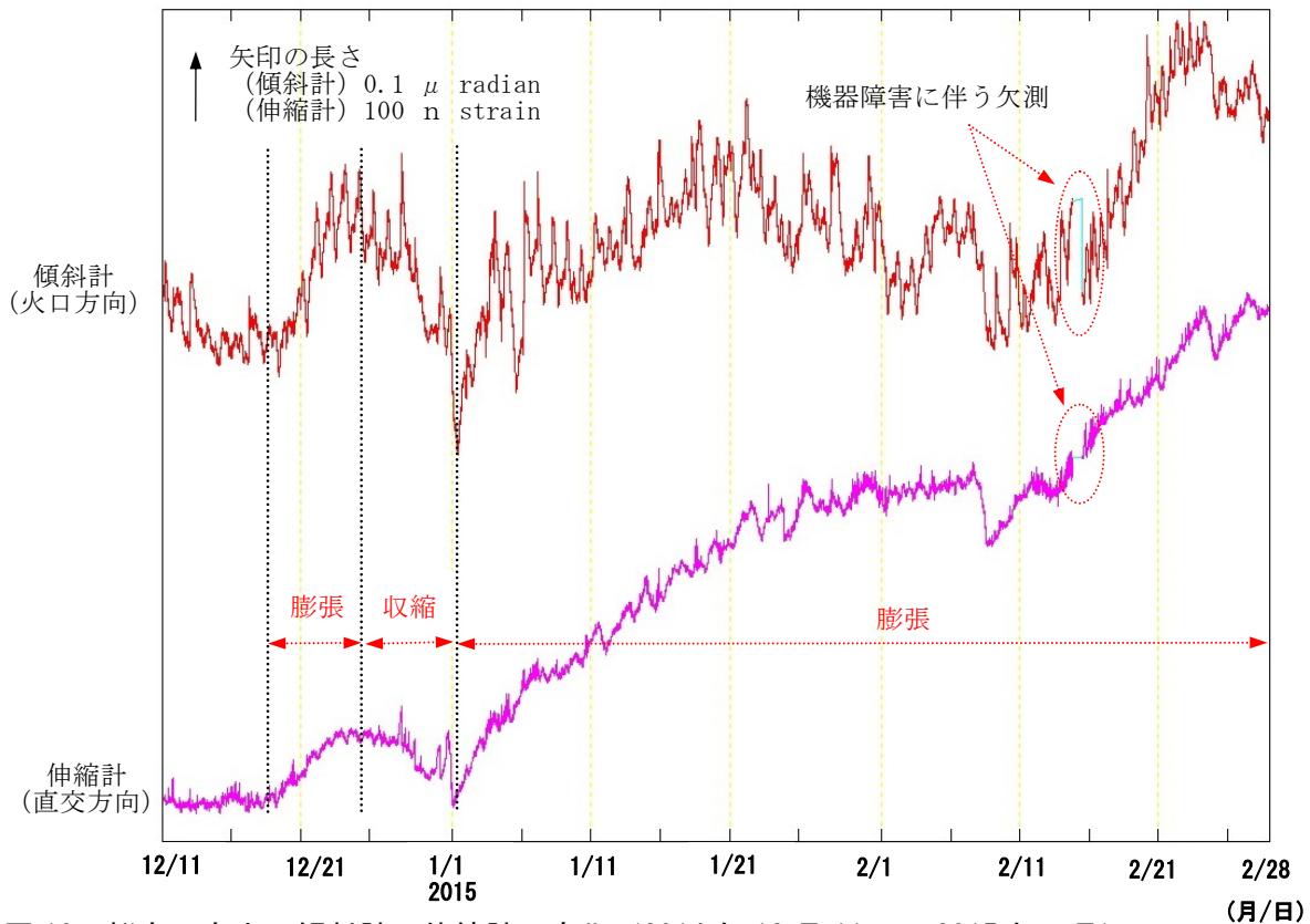
図10 桜島 島内の傾斜計・伸縮計の変化（2014年12月11日～2015年2月） （有村観測坑道の水管傾斜計及び伸縮計（大隅河川国道事務所設置））
