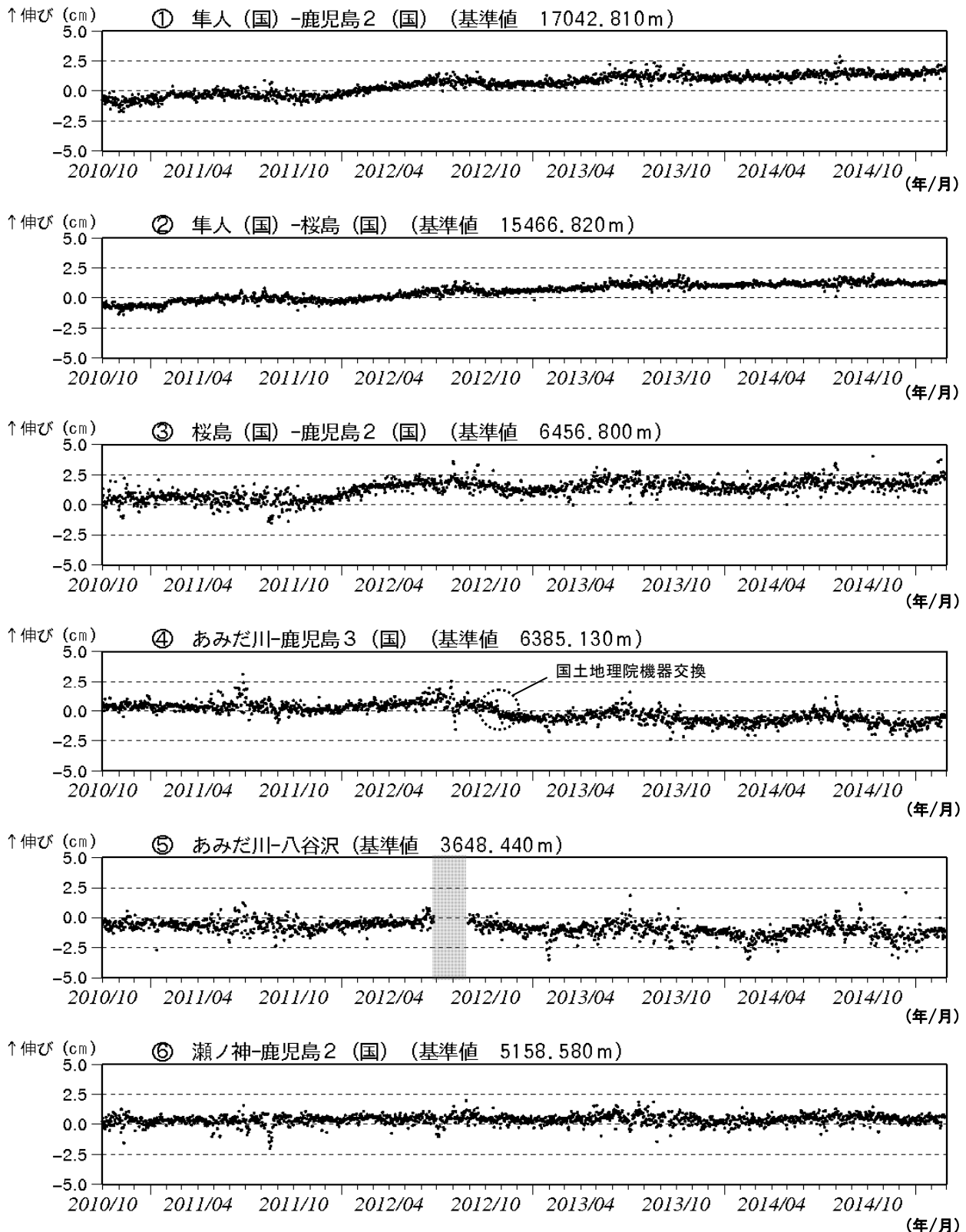
図 11-1 桜島 GNSS 連続観測による基線長変化 (2010 年 10 月～2015 年 2 月)
