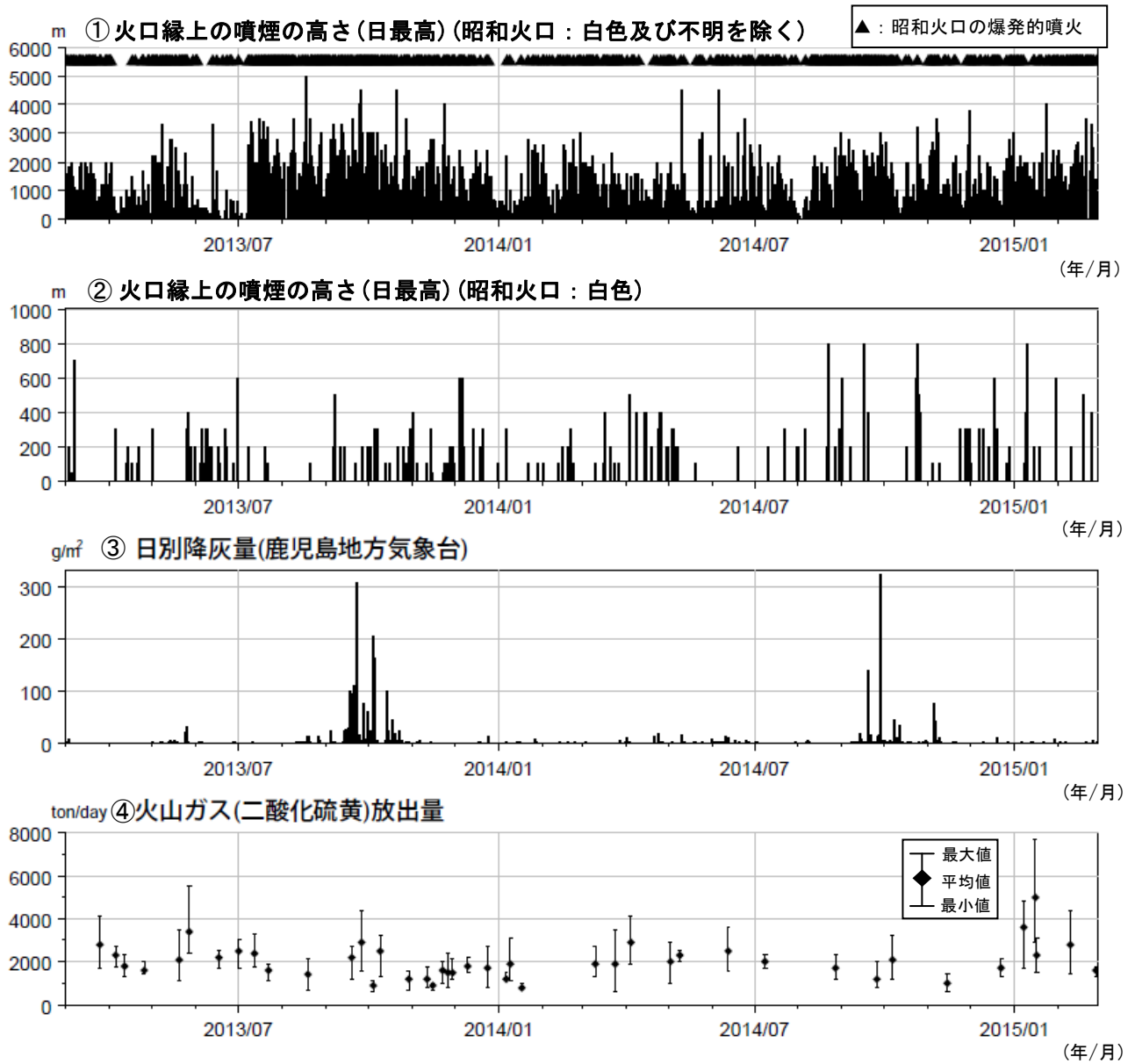
図 6 桜島 最近 2 年間の噴煙、降灰、火山ガス（2013 年 3 月～2015 年 2 月）
