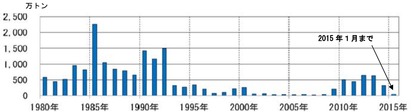
図5 桜島 鹿児島県が実施している降灰の観測データから推定した火山灰の年別総噴出量 （1980年～2015年1月）
