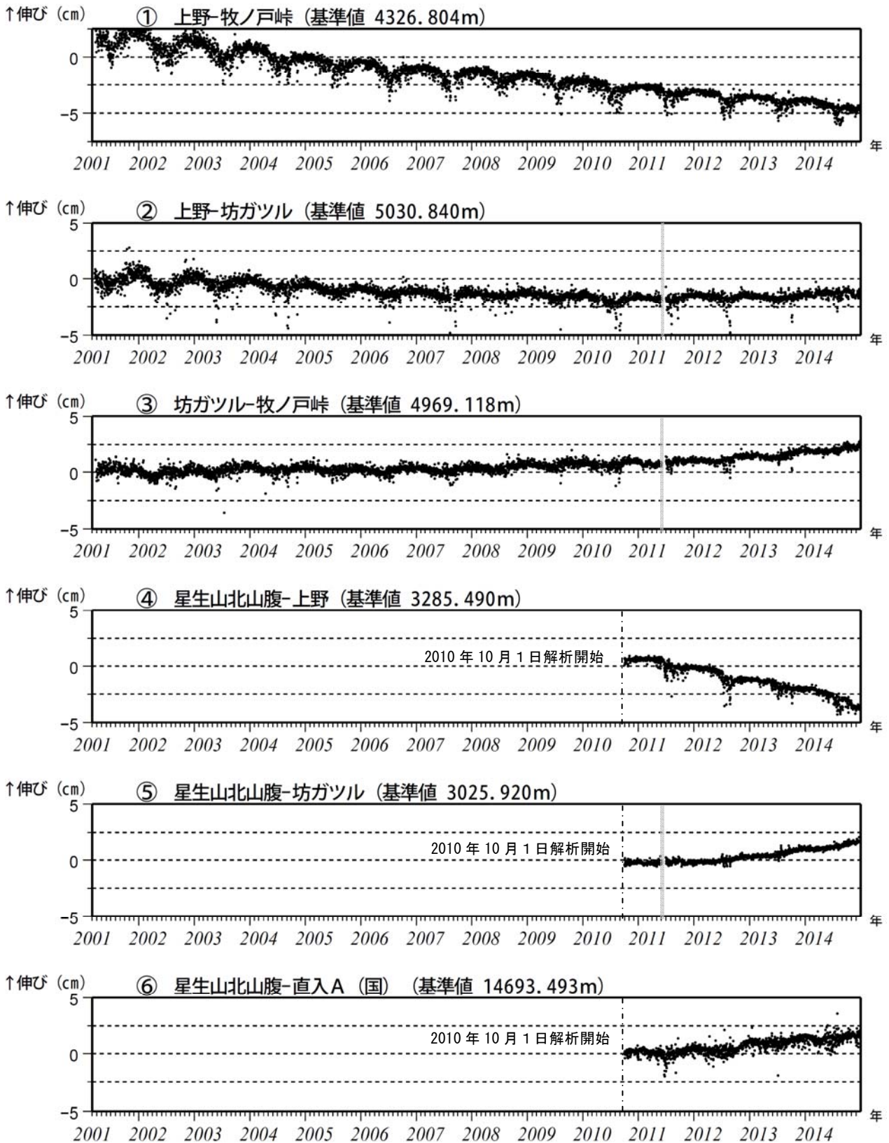
図5 九重山 GNSS 連続観測による基線長変化 (2001年3月~2014年12月)
