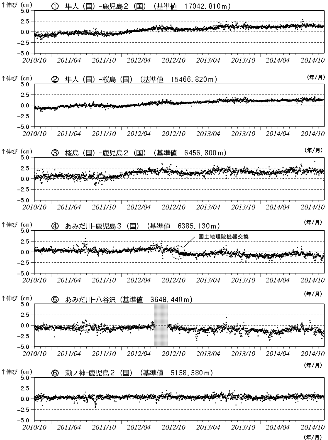
図 12-1 桜島 GNSS 連続観測による基線長変化 (2010 年 10 月～2014 年 11 月)
