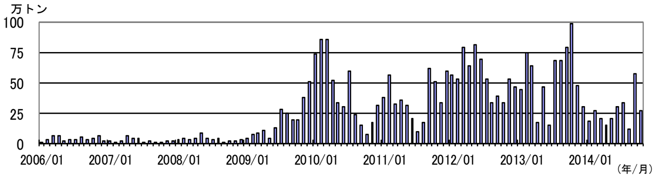
図5 桜島 鹿児島県が実施している降灰の観測データから推定した火山灰の月別総噴出量 （2006年1月～2014年10月）
