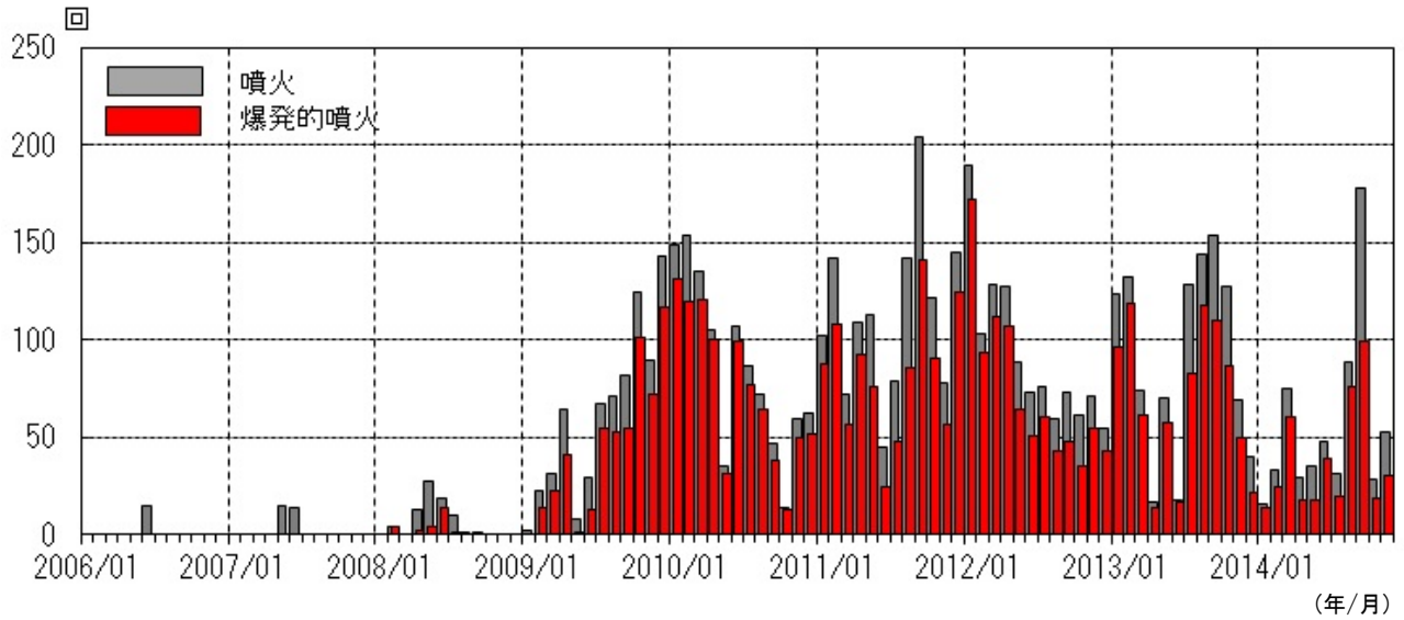
図4 桜島 昭和火口月別噴火回数（灰色）と昭和火口月別爆発回数（赤色） （2006年1月～2014年11月）
