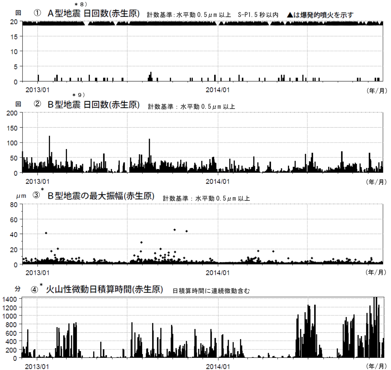
図 8 桜島 最近 2 年間の火山性地震、火山性微動（2012 年 12 月～2014 年 11 月）
