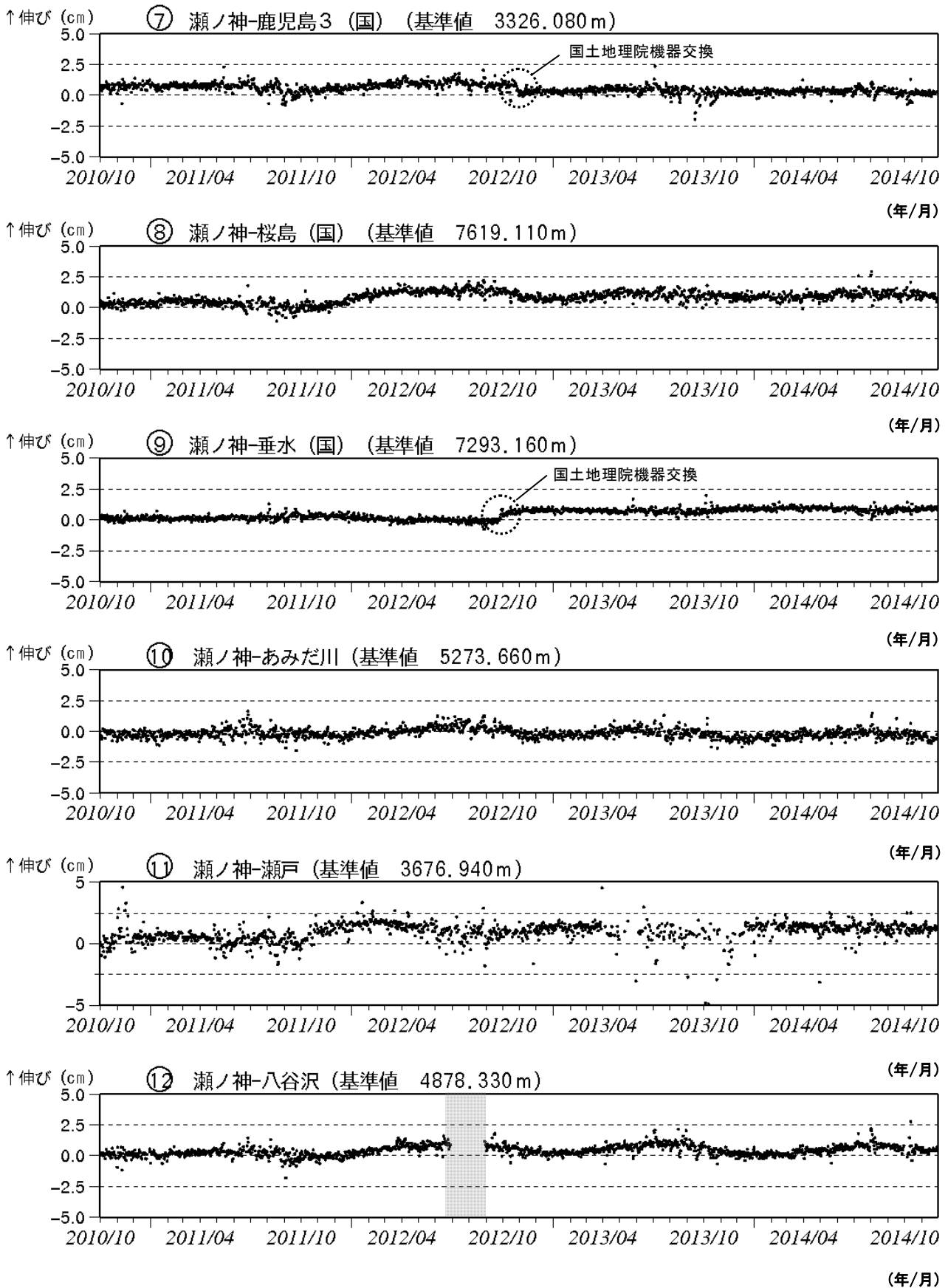
図 12-2 桜島 GNSS 連続観測による基線長変化 (2010 年 10 月～2014 年 11 月)
