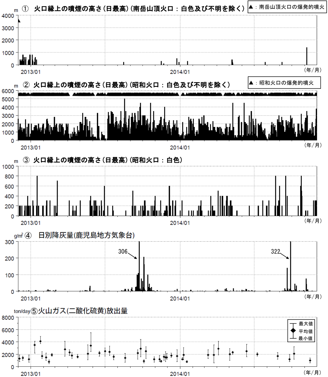
図7 桜島 最近2年間の噴煙、降灰、火山ガス（2012年12月～2014年11月）
