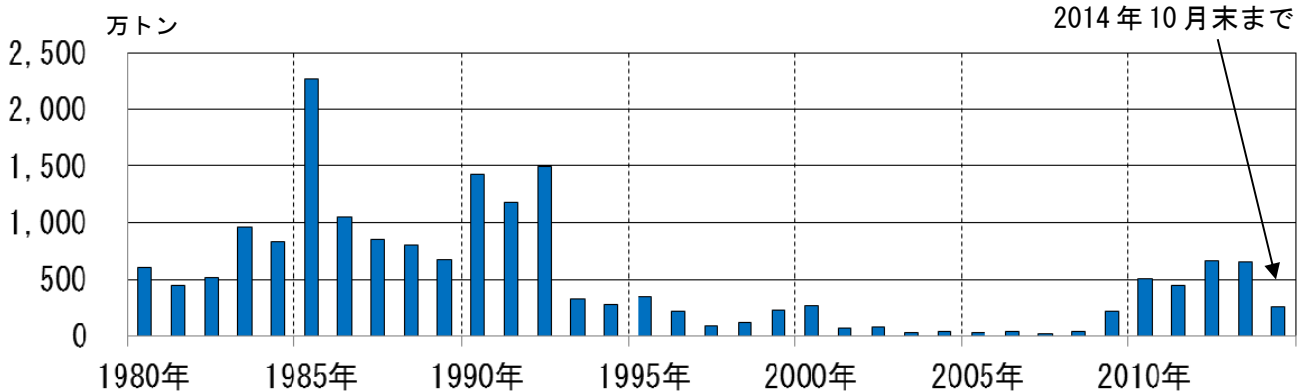
図6 桜島 鹿児島県が実施している降灰の観測データから推定した火山灰の年別総噴出量 （1980年～2014年10月）
