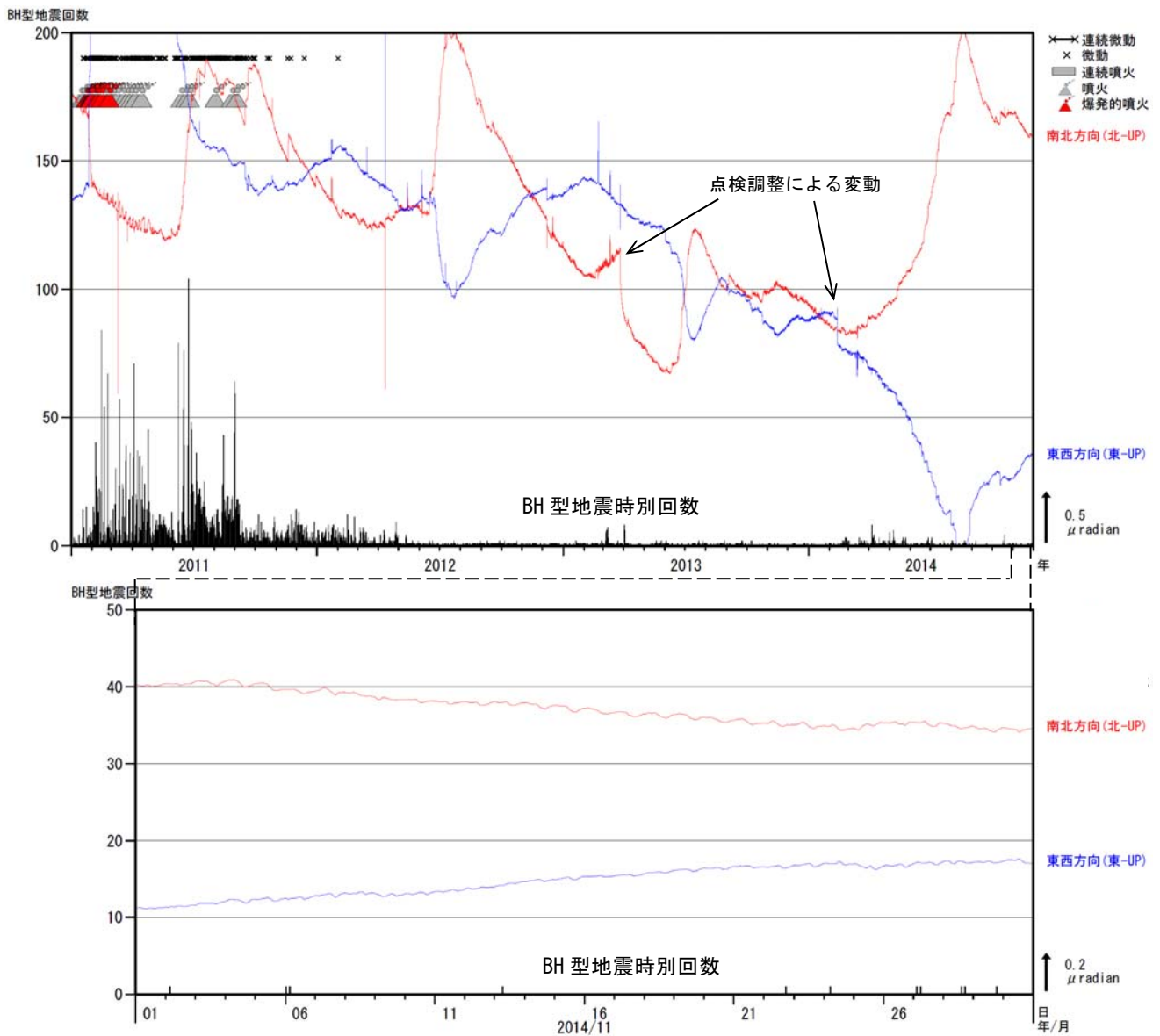
図4 霧島山（新燃岳） BH型地震の時間別回数と高千穂河原傾斜計の傾斜変動（2011年1月～2014年11月）
