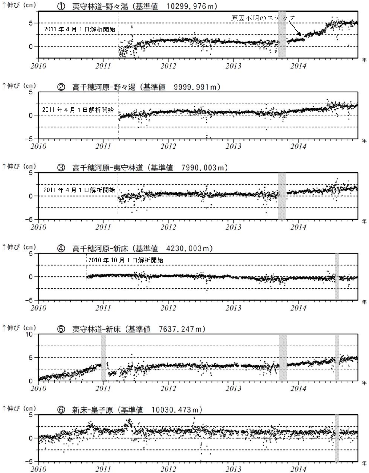
図 6-1 霧島山 GNSS 連続観測による基線長変化（2010 年 1 月～2014 年 11 月）
