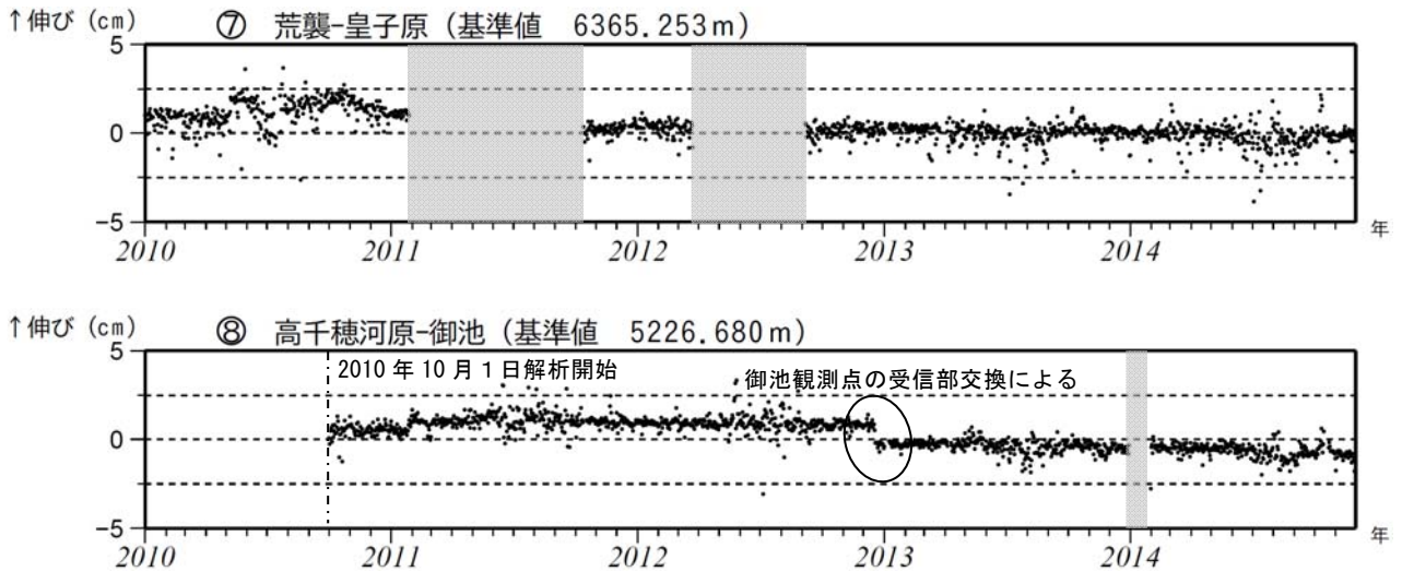
図 6-2 霧島山 GNSS 連続観測による基線長変化（2010 年 1 月～2014 年 11 月）
