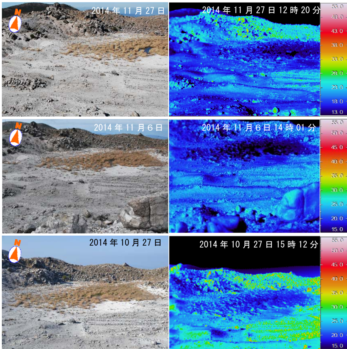
図 14-3 霧島山（えびの高原（硫黄山）周辺） 可視画像および赤外熱映像装置による地表面温度分布（硫黄山火口の南側から火口底及び北側火口壁を撮影）
