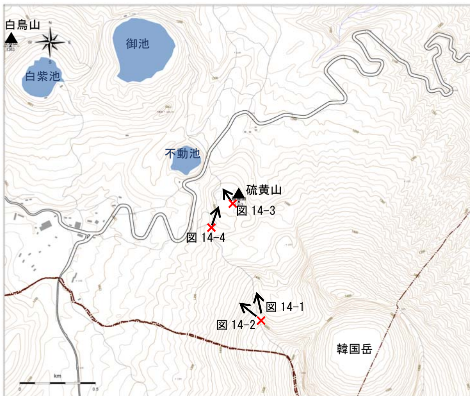
図 15 霧島山（えびの高原（硫黄山）付近） 図 14 の撮影位置図（×は撮影位置を、矢印は撮影方向を示します）
