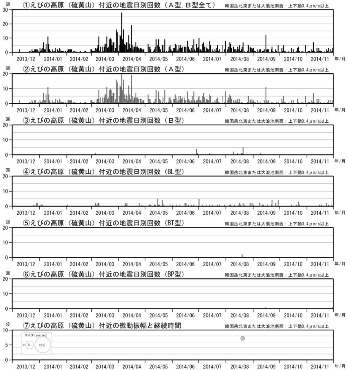
図 12 霧島山（えびの高原（硫黄山）周辺） 火山活動経過図（2013 年 12 月～2014 年 11 月）
