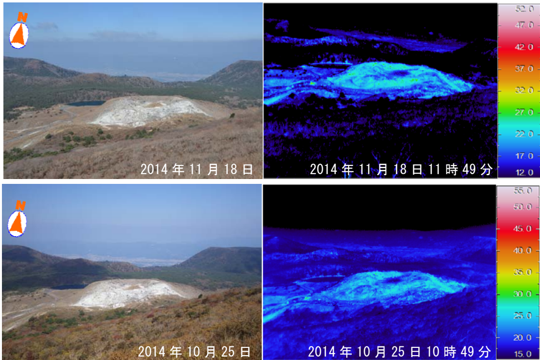
図 14-1 霧島山（えびの高原（硫黄山）周辺） 可視画像および赤外熱映像装置による地表面温度分布（韓国岳中腹から硫黄山の南側及び火口内を撮影）
