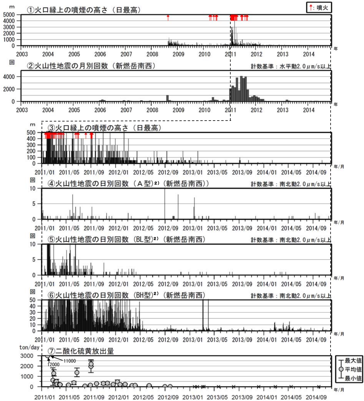
図3 霧島山（新燃岳） 火山活動経過図（2003年1月～2014年11月）
