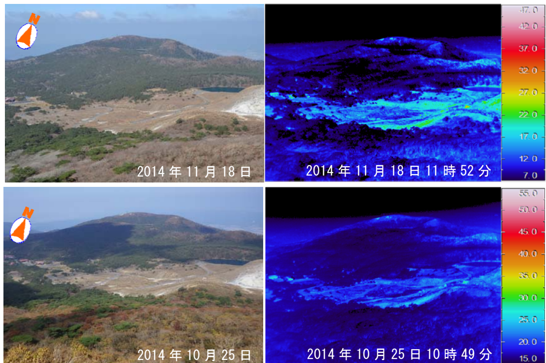
図 14-2 霧島山（えびの高原（硫黄山）周辺） 可視画像および赤外熱映像装置による地表面温度分布（韓国岳中腹からえびの高原方向を撮影）
