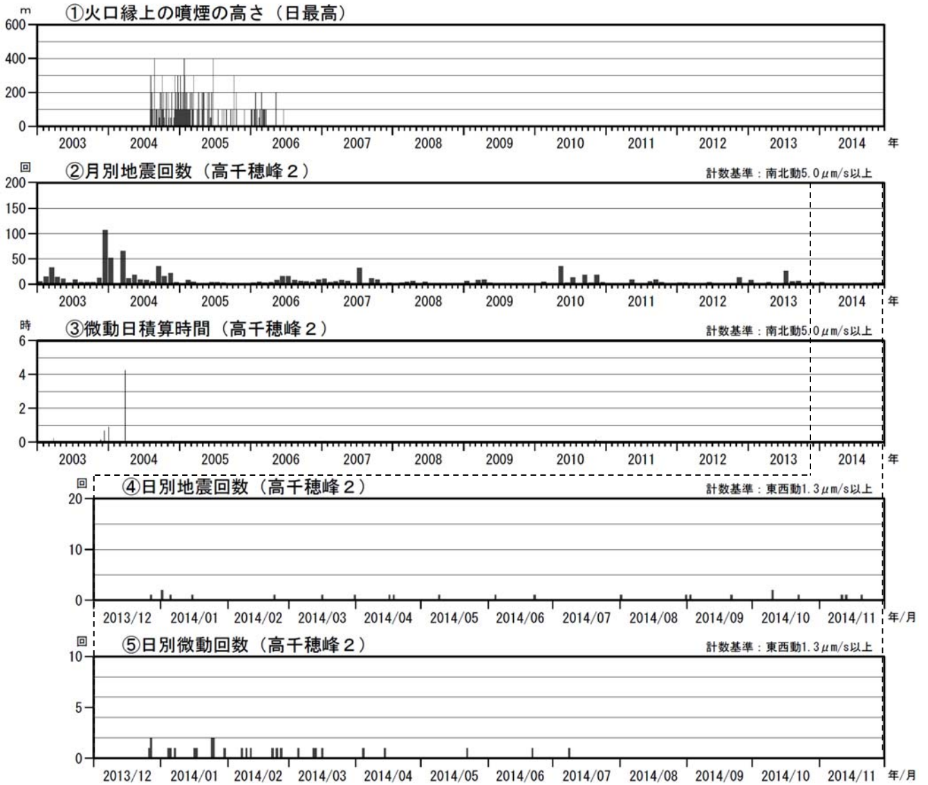
図 10 霧島山（御鉢） 火山活動経過図（2003 年 1 月～2014 年 11 月）
