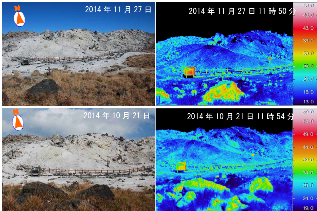
図 14-4 霧島山（えびの高原（硫黄山）周辺） 可視画像および赤外熱映像装置による地表面温度分布（韓国岳登山道入り口のベンチから硫黄山南側斜面を撮影）
