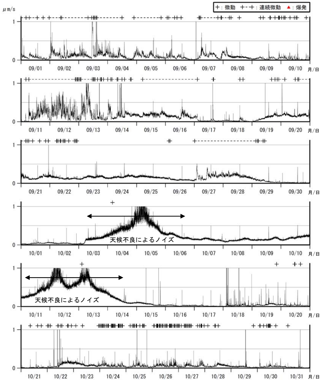
図4 諏訪之瀬島 1分間平均振幅の時間変化 （トンガマ南西観測点上下動成分）（2014年9～10月）
