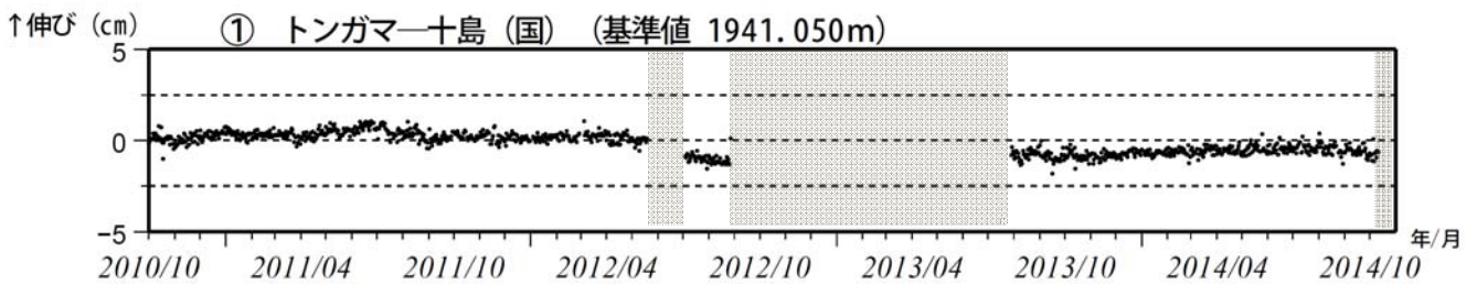
図5 諏訪之瀬島 GNSS連続観測による基線長変化（2010年10月～2014年10月）
