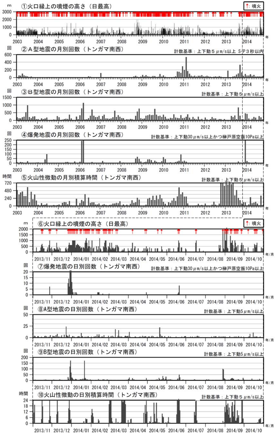
図3 諏訪之瀬島 火山活動経過図（2003年1月～2014年10月）
