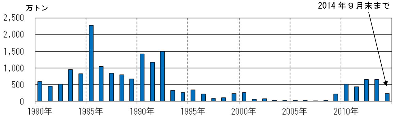
図5 桜島 鹿児島県が実施している降灰の観測データから推定した火山灰の年別総噴出量 （1980年～2014年9月）
