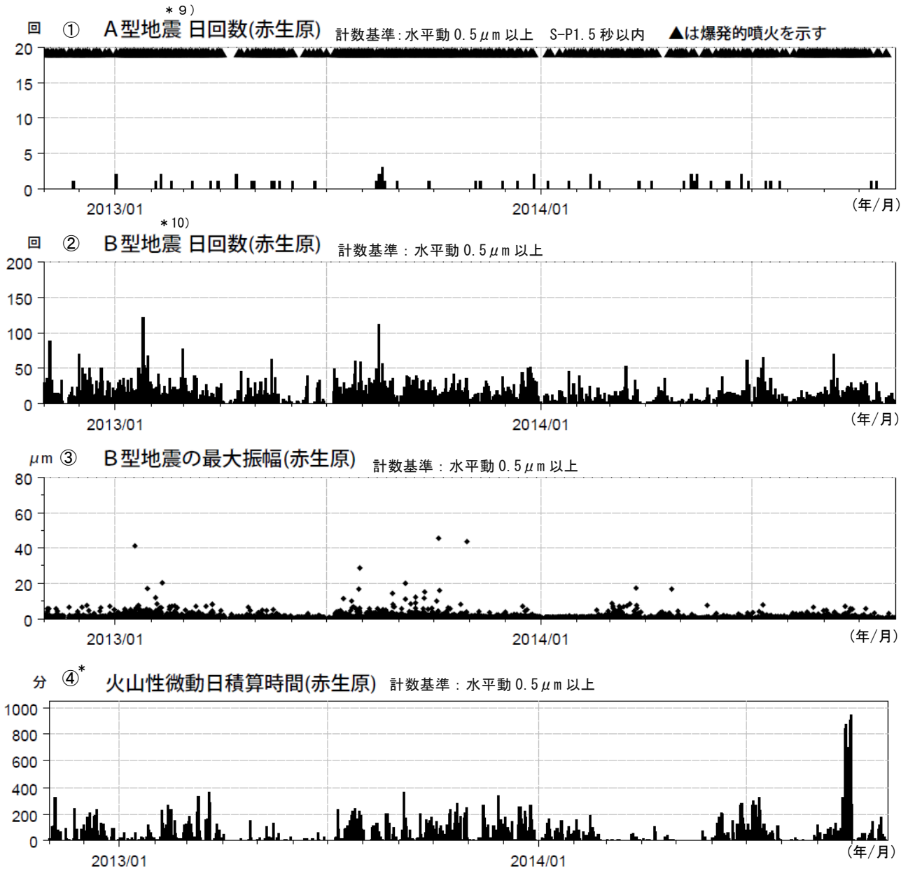
図 7 桜島 最近 2 年間の火山性地震、火山性微動（2012 年 11 月～2014 年 10 月）
