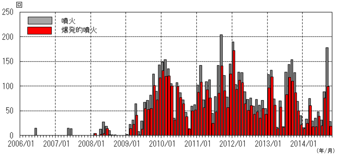
図3 桜島 昭和火口月別噴火回数（灰色）と昭和火口月別爆発回数（赤色） （2006年1月～2014年10月）
