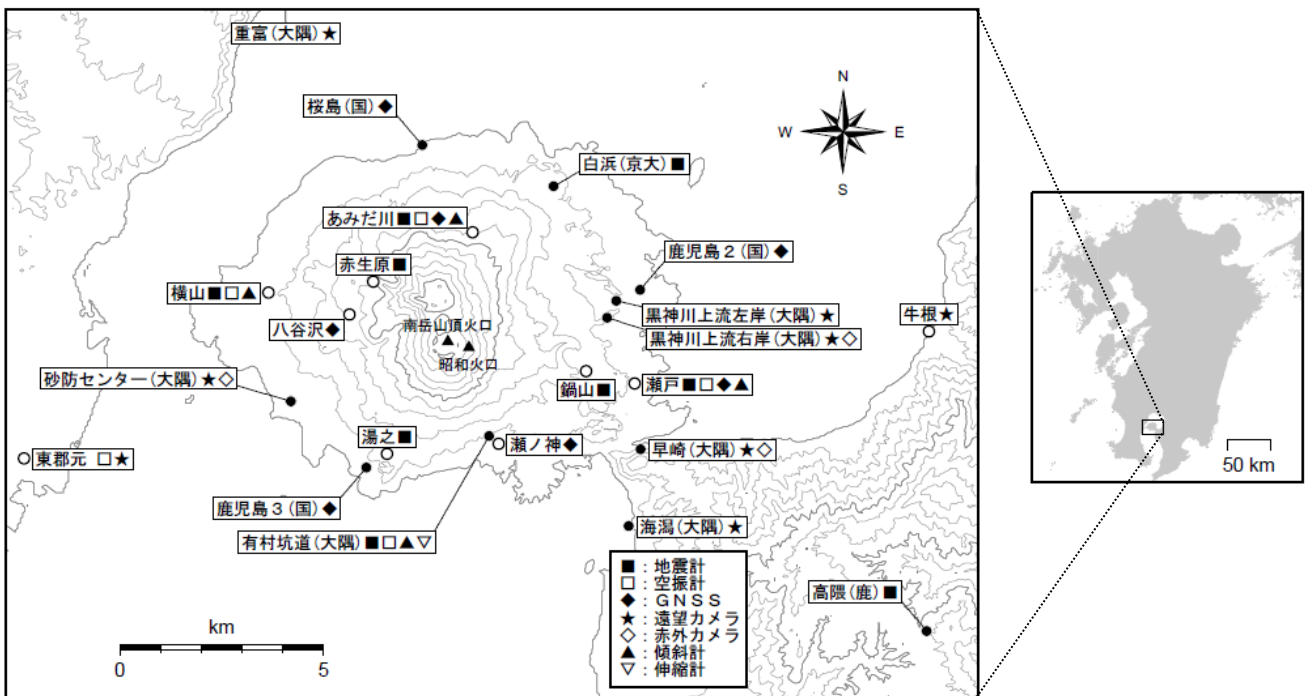
国土地理院 数値地図 50mメッシュ (標高) 使用 小さな白丸 (○) は気象庁、小さな黒丸 (●) は気象庁以外の機関の観測点位置を示しています。
