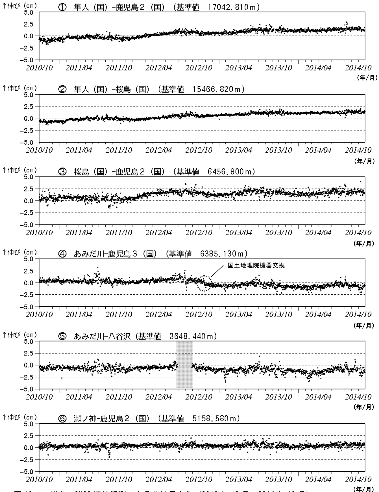
図 10-1 桜島 GNSS 連続観測による基線長変化 (2010 年 10 月～2014 年 10 月)
