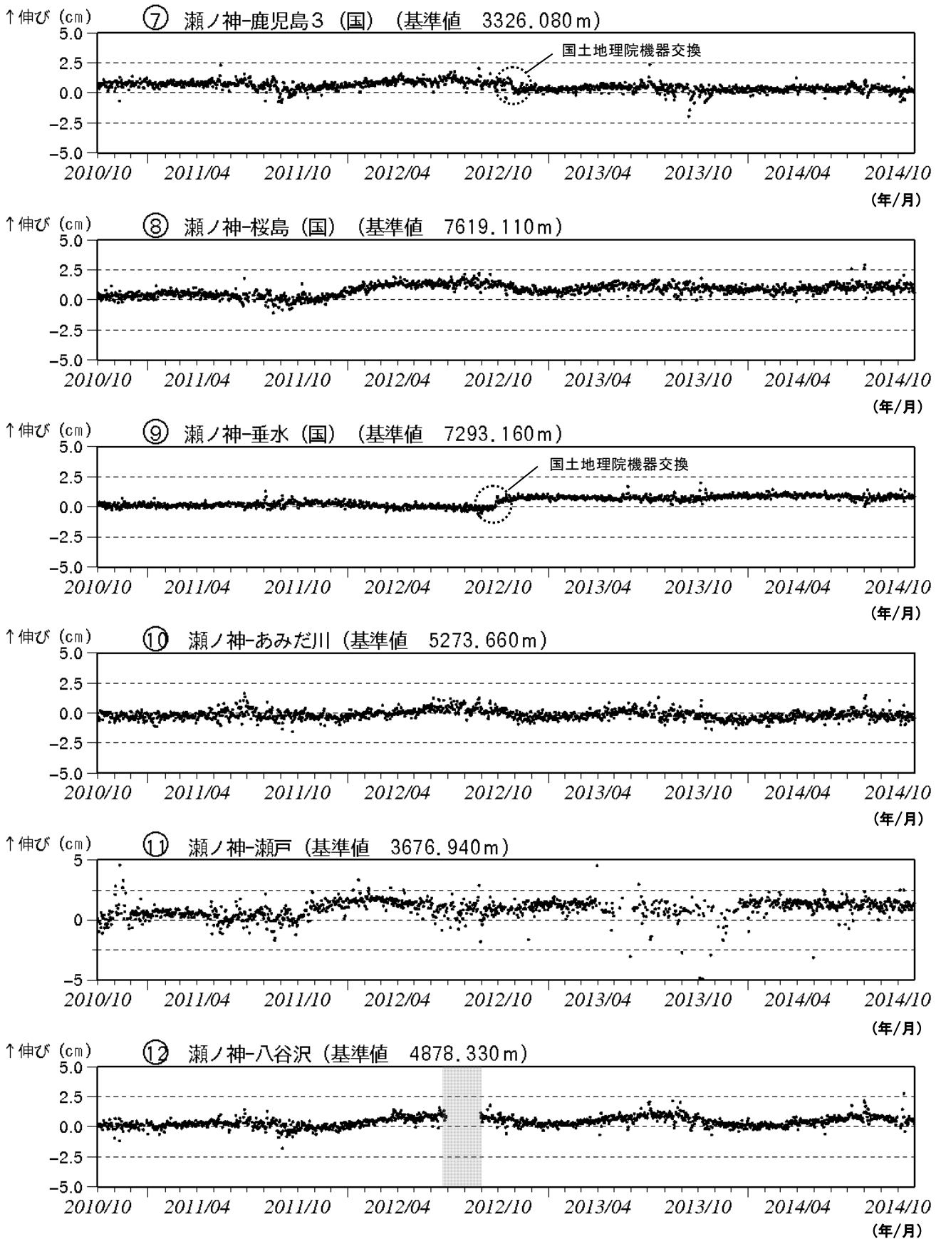
図 10-2 桜島 GNSS 連続観測による基線長変化（2010 年 10 月～2014 年 10 月）
