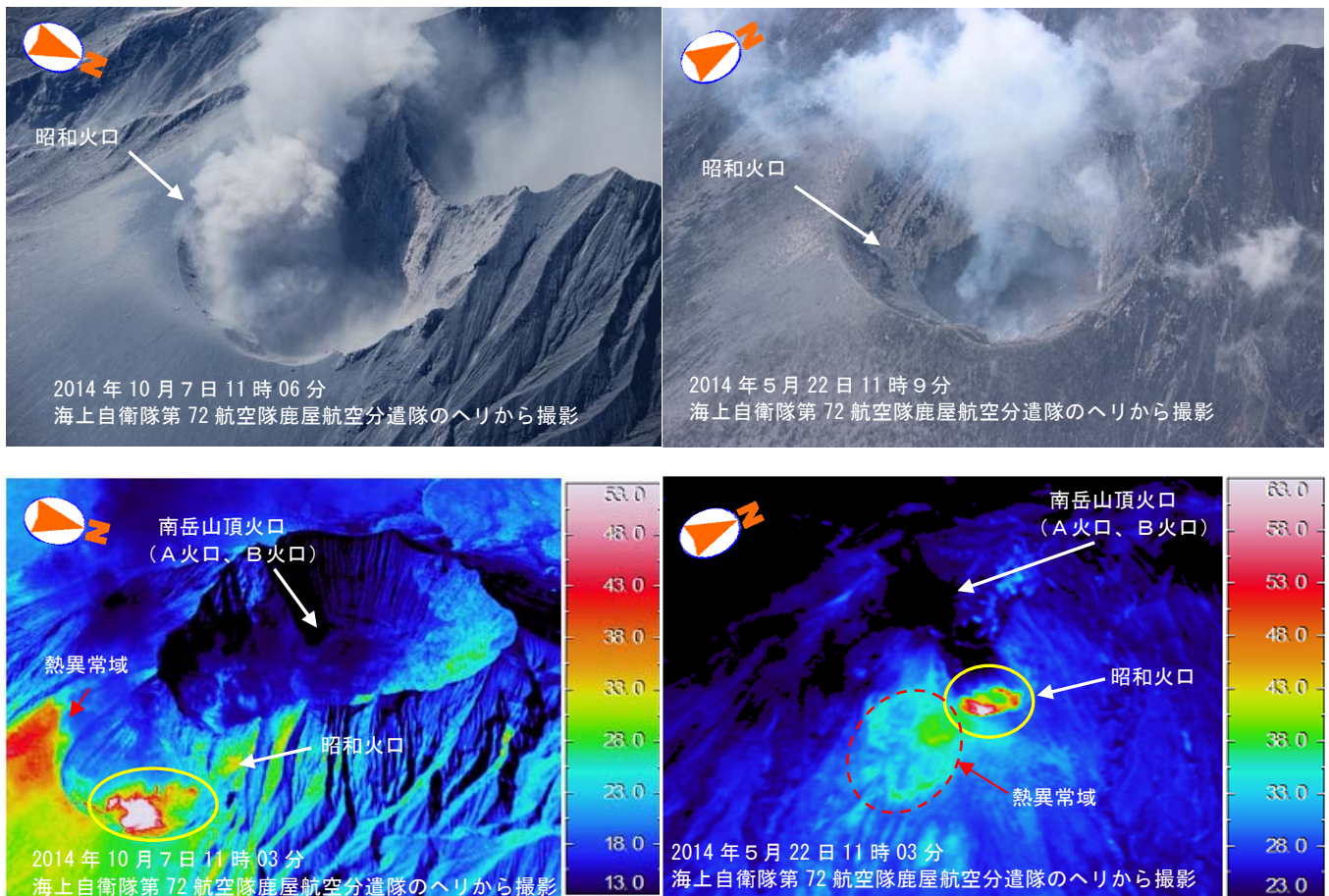
図 12 桜島 昭和火口の状況および赤外熱映像装置による地表面温度分布 (左：2014年10月7日、右：2014年5月22日)
