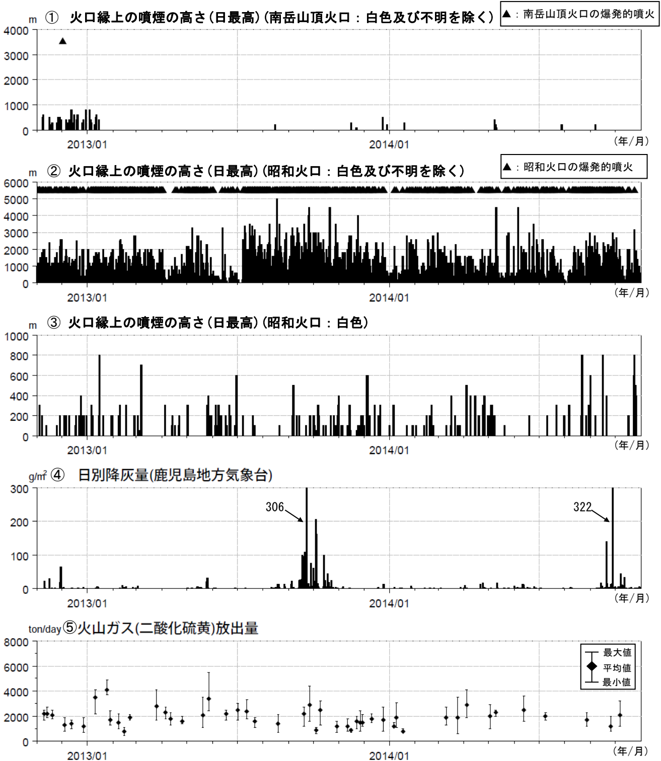
図6 桜島 最近2年間の噴煙、降灰、火山ガス（2012年11月～2014年10月）
