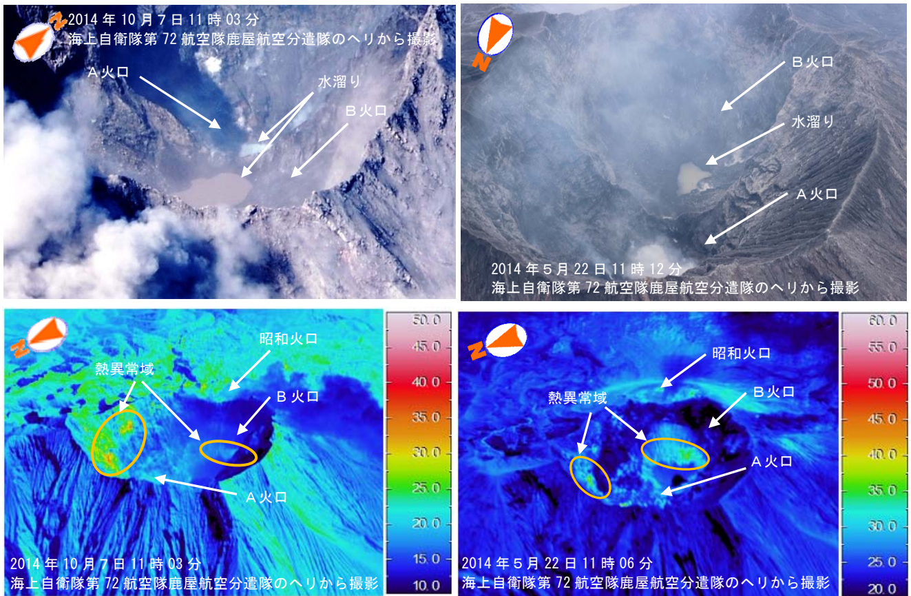
図 13 桜島 南岳山頂火口の状況および赤外熱映像装置による地表面温度分布 （左：2014 年 10 月 7 日、右：2014 年 5 月 22 日）
