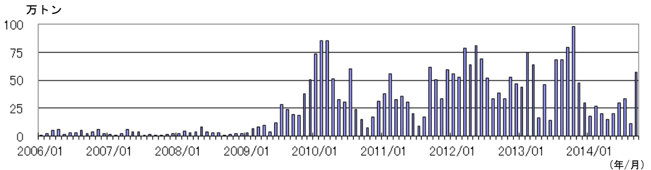
図4 桜島 鹿児島県が実施している降灰の観測データから推定した火山灰の月別総噴出量 （2006年1月～2014年9月）
