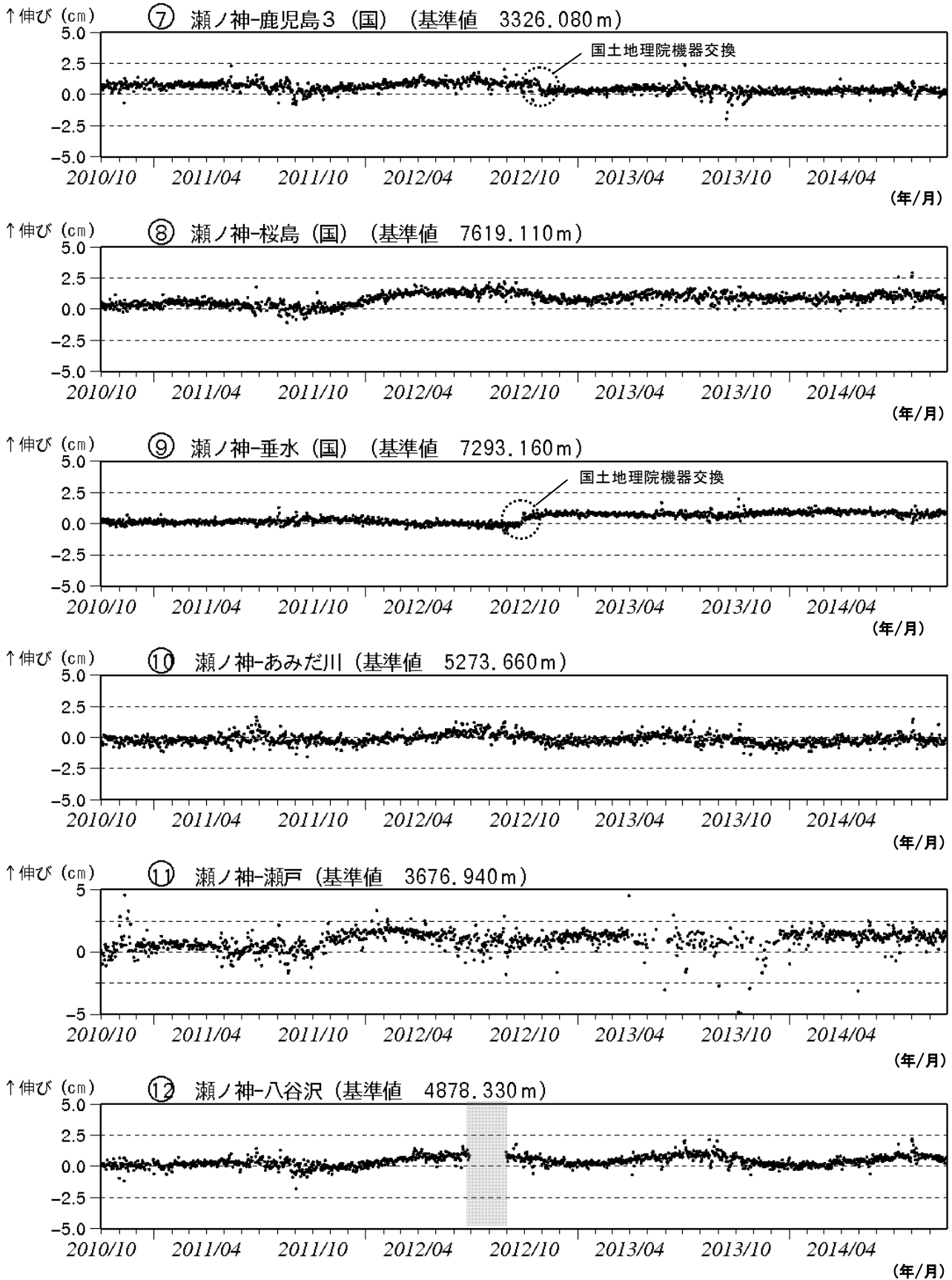
図 10-2 桜島 GNSS 連続観測による基線長変化 (2010 年 10 月～2014 年 9 月)
