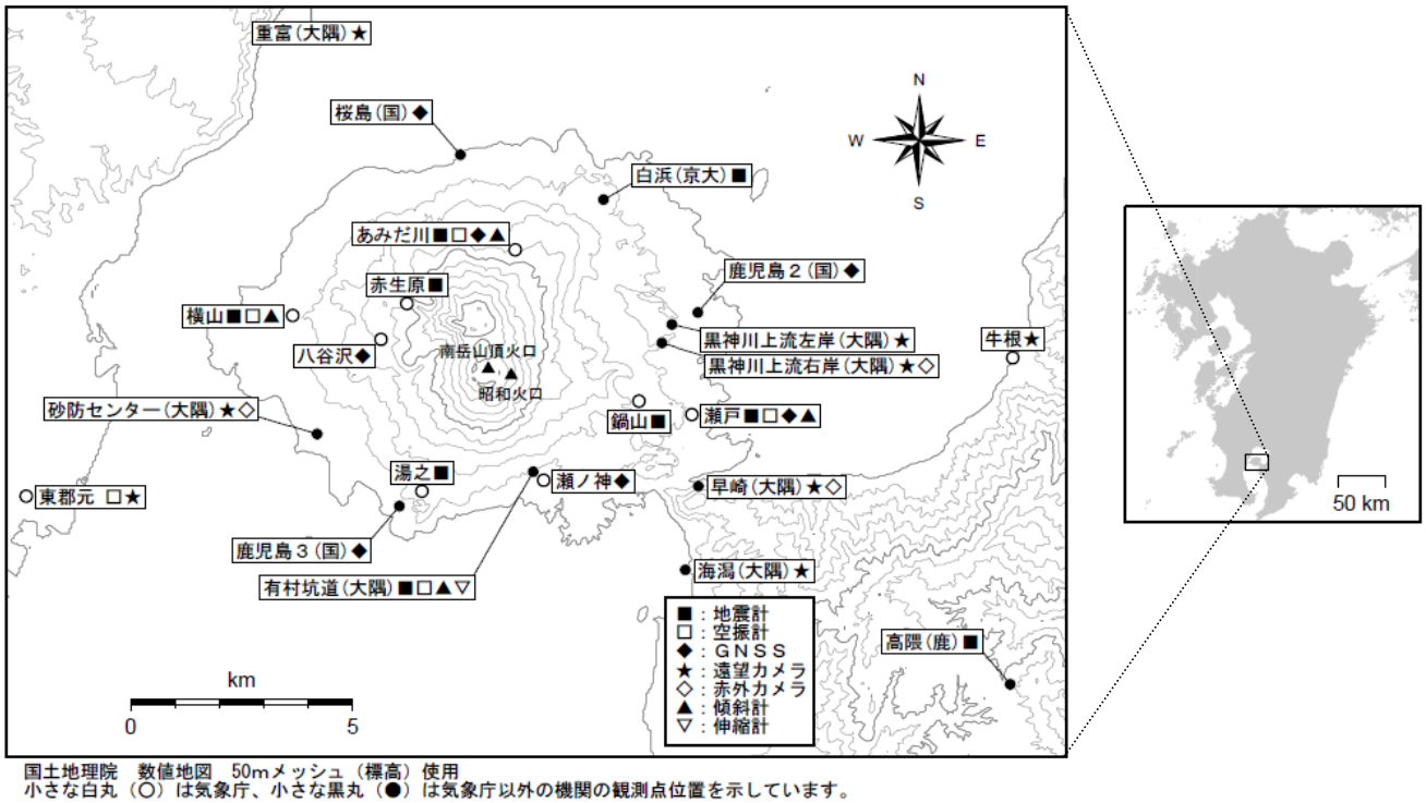
図12 桜島 観測点配置図
