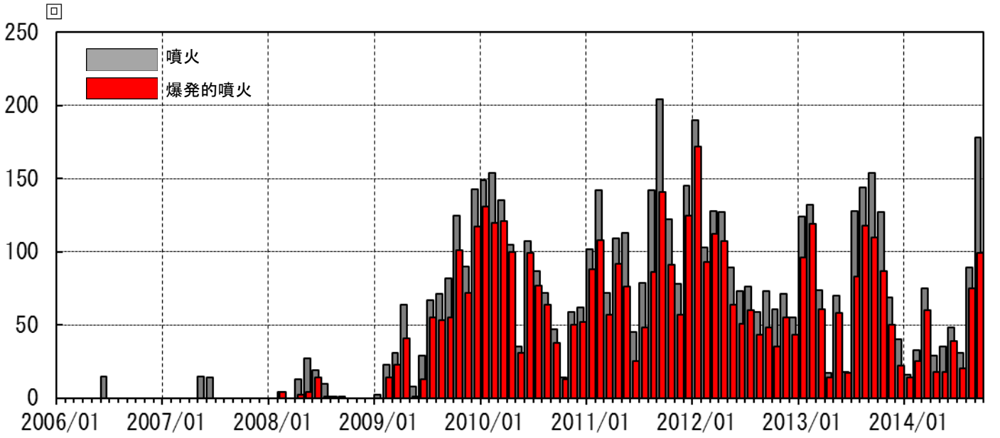
図3 桜島 昭和火口月別噴火回数（灰色）と昭和火口月別爆発回数（赤色） （年/月） （2006年1月～2014年9月）
