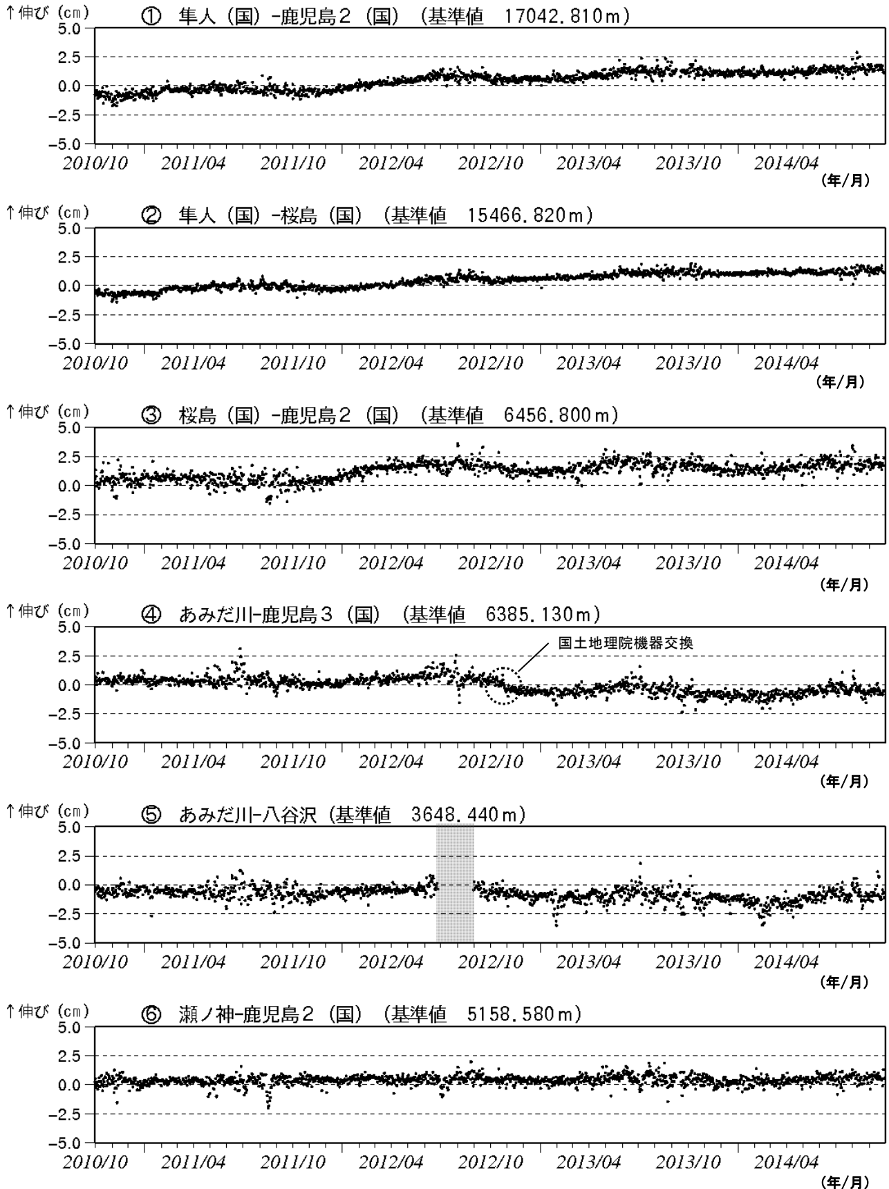
図 10-1 桜島 GNSS 連続観測による基線長変化（2010 年 10 月～2014 年 9 月）
