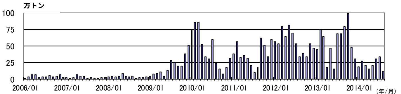
図4 桜島 鹿児島県が実施している降灰の観測データから推定した火山灰の月別総噴出量 （2006年1月～2014年8月）
