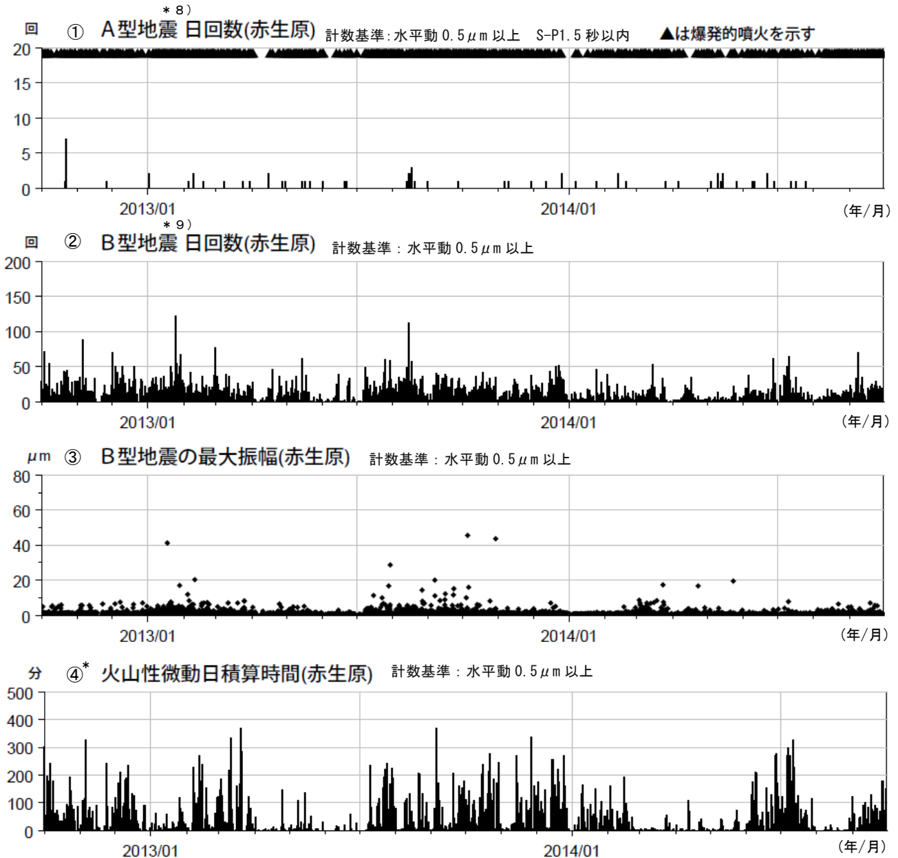
図7 桜島 最近2年間の火山性地震、火山性微動（2012年10月～2014年9月）
