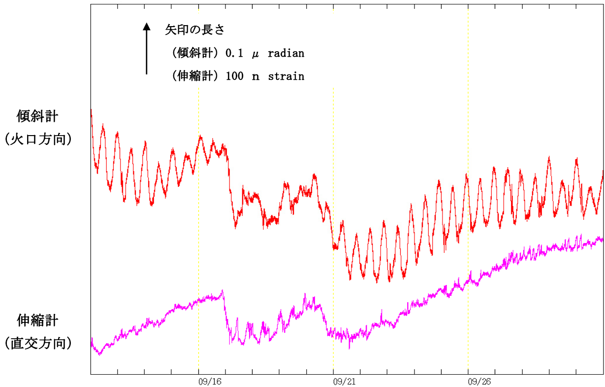
図 9 桜島 島内の傾斜計及び伸縮計の変化（2014 年 9 月 12 日～30 日） （有村観測坑道の水管傾斜計及び伸縮計（大隅河川国道事務所設置））
