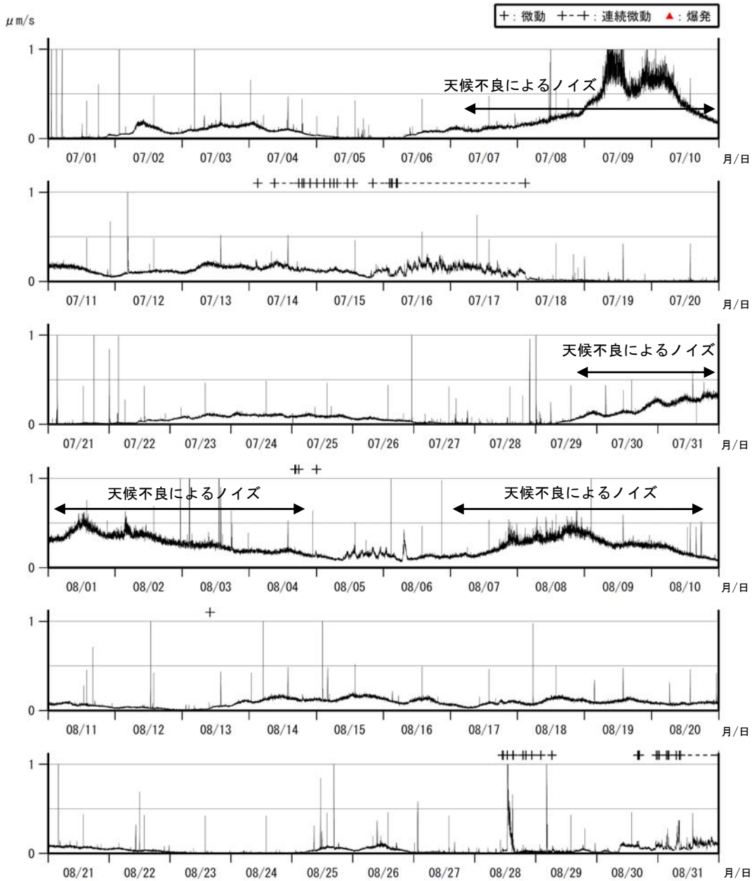
図 4 諏訪之瀬島 1 分間平均振幅の時間変化 （トンガマ南西観測点上下動成分）（2014 年 7～8 月）
