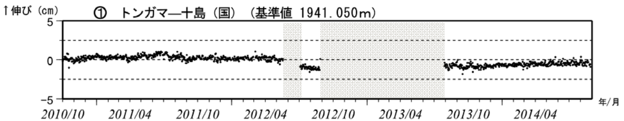
図 5 諏訪之瀬島 GNSS連続観測による基線長変化（2010 年 10 月～2014 年 8 月）
