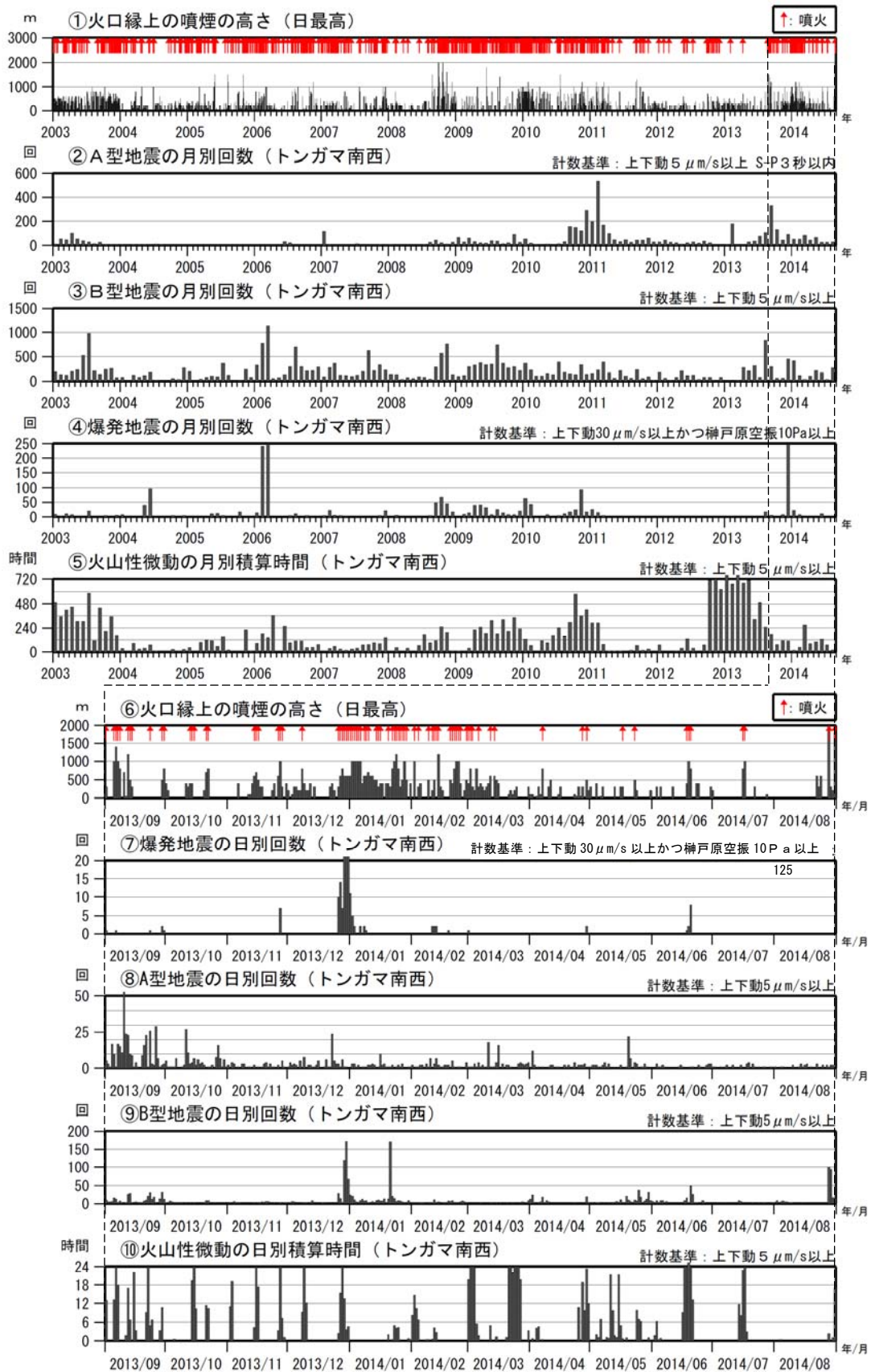
図 3 諏訪之瀬島 火山活動経過図（2003 年 1 月～2014 年 8 月）
