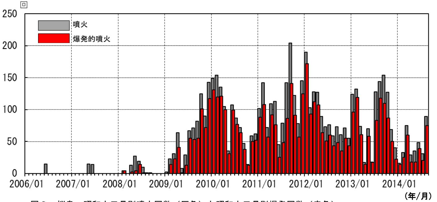
図3 桜島 昭和火口月別噴火回数（灰色）と昭和火口月別爆発回数（赤色） （2006年1月～2014年8月）
