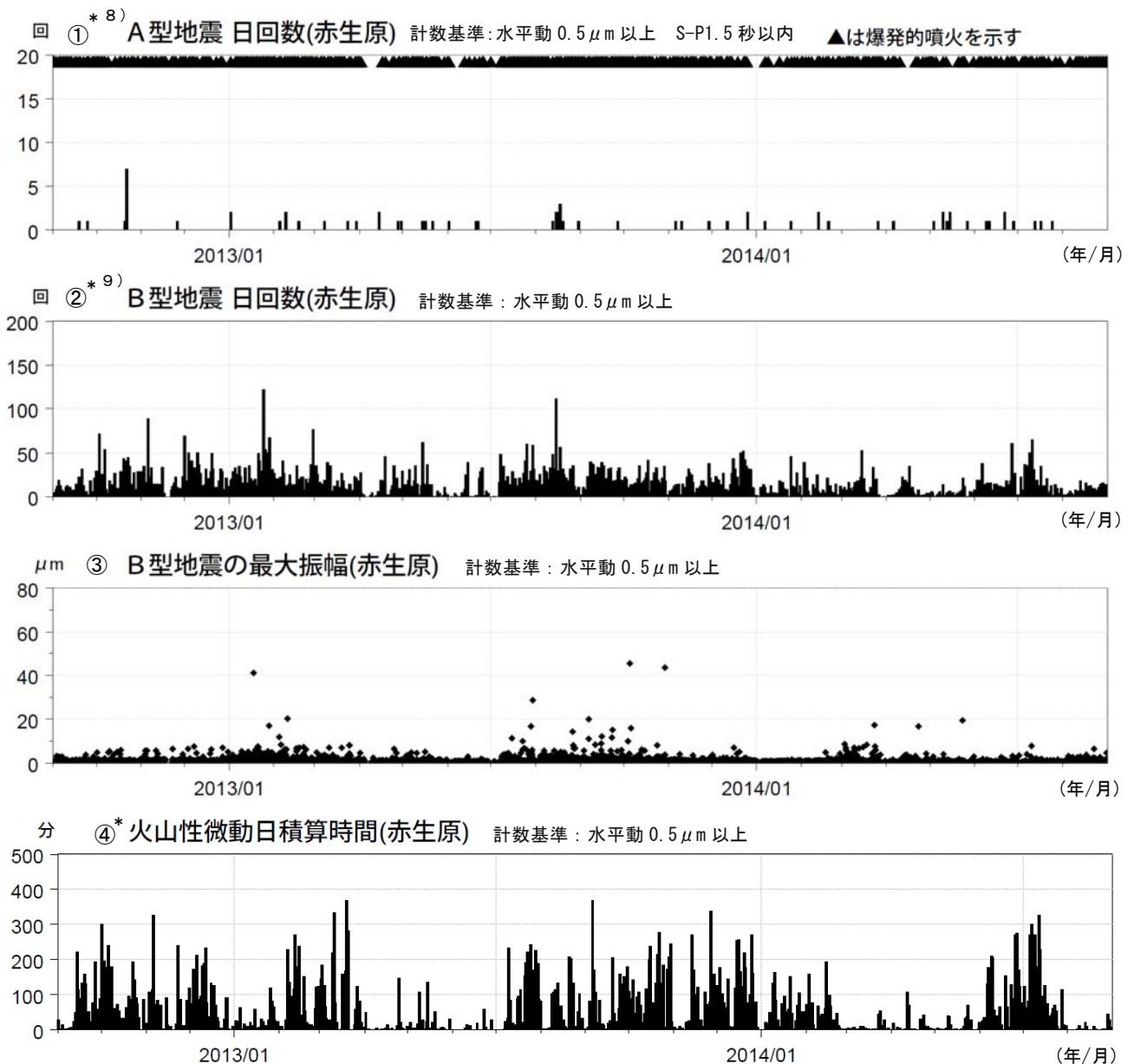
図6 桜島 最近2年間の火山性地震、火山性微動（2012年9月～2014年8月）
