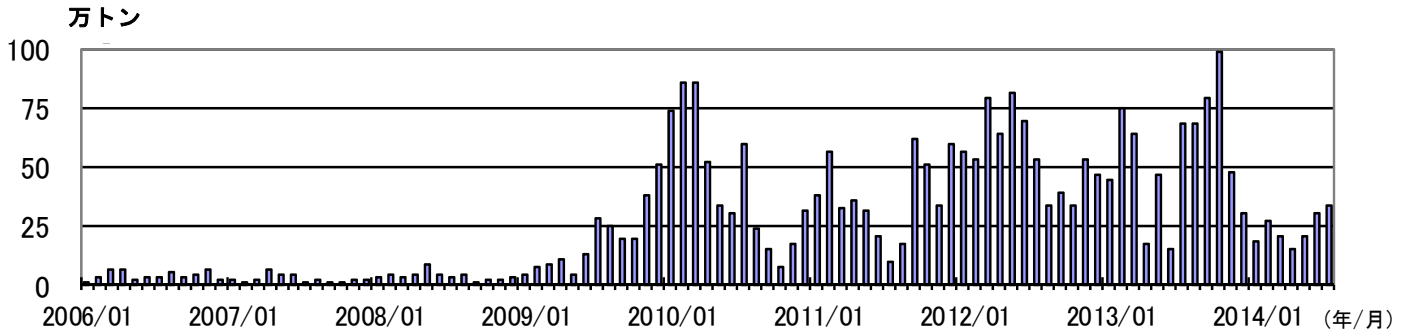
図7 桜島 鹿児島県が実施している降灰の観測データから推定した火山灰の月別総噴出量 （2006年1月～2014年7月）
