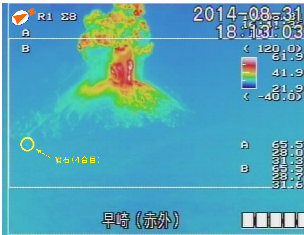
図 2 桜島 31 日 18 時 12 分の昭和火口の爆発的噴火の状況 (早崎熱カメラ：大隅河川国道事務所設置)
