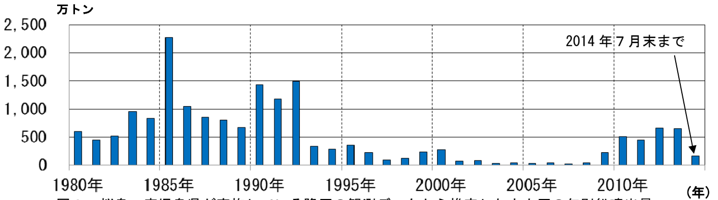
図8 桜島 鹿児島県が実施している降灰の観測データから推定した火山灰の年別総噴出量 （1980年～2014年7月）
