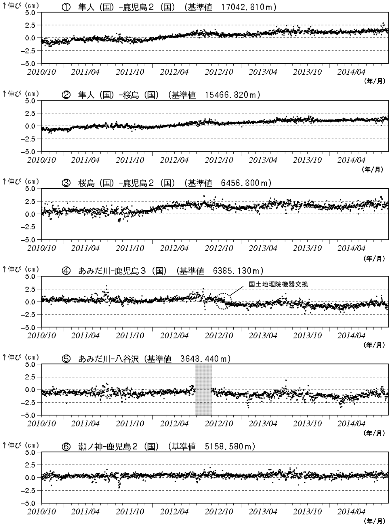
図 10-1 桜島 GNSS 連続観測による基線長変化 (2010 年 10 月～2014 年 8 月)
