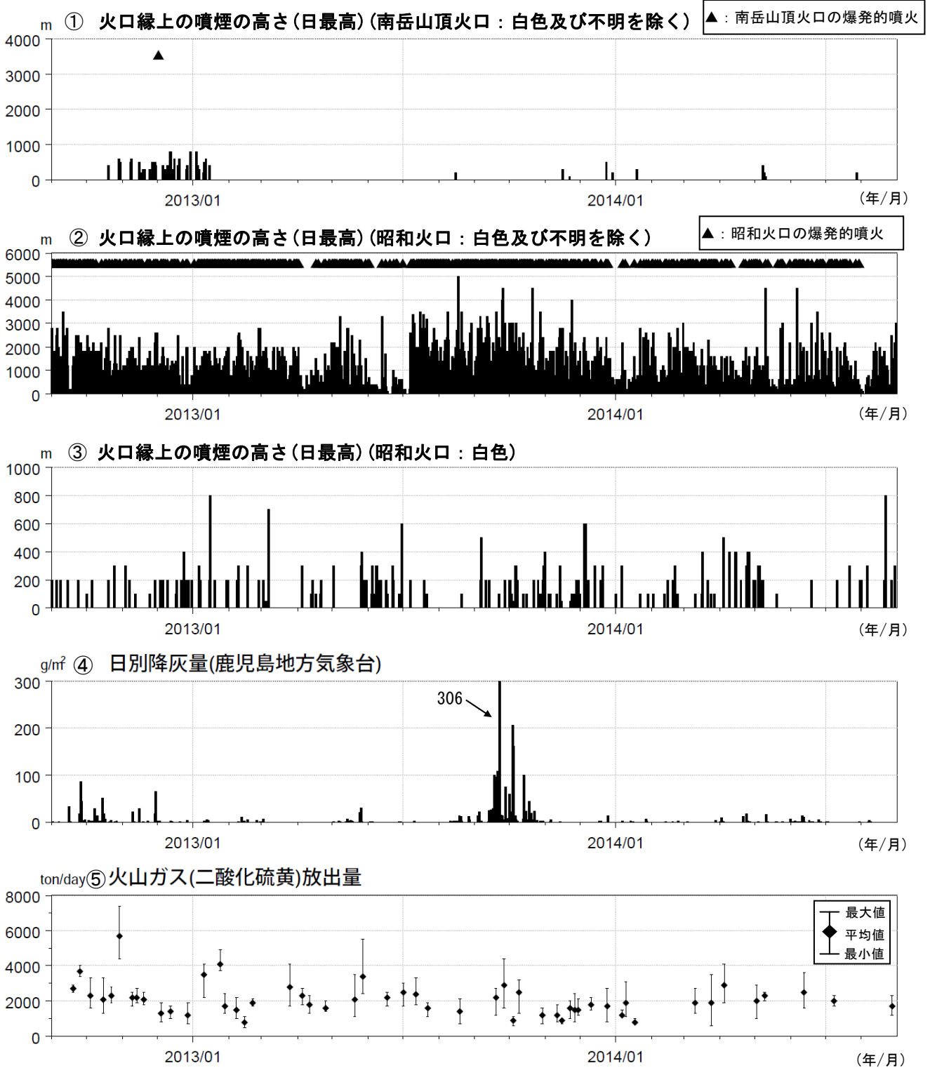
図5 桜島 最近2年間の噴煙、降灰、火山ガス（2012年9月～2014年8月）
