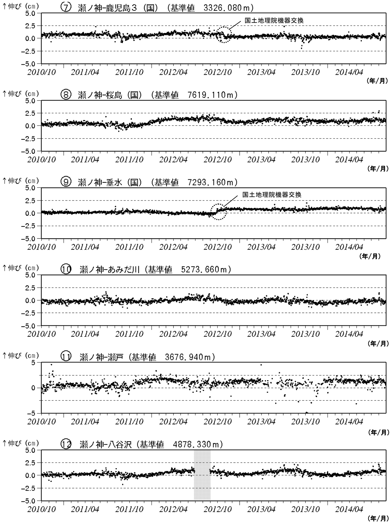
図 10-2 桜島 GNSS 連続観測による基線長変化 (2010 年 10 月～2014 年 8 月)
