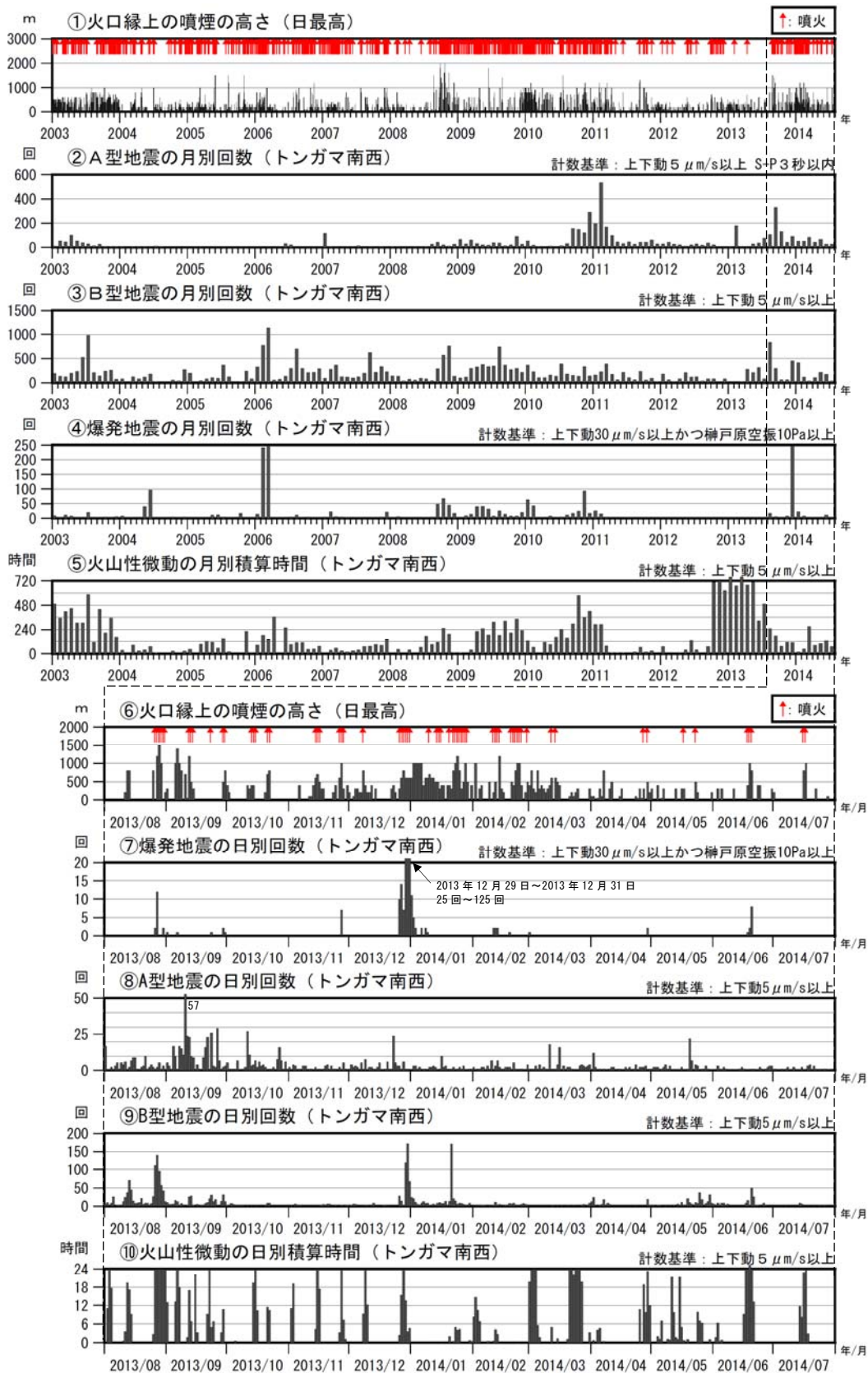
図3 諏訪之瀬島 火山活動経過図（2003年1月～2014年7月）
