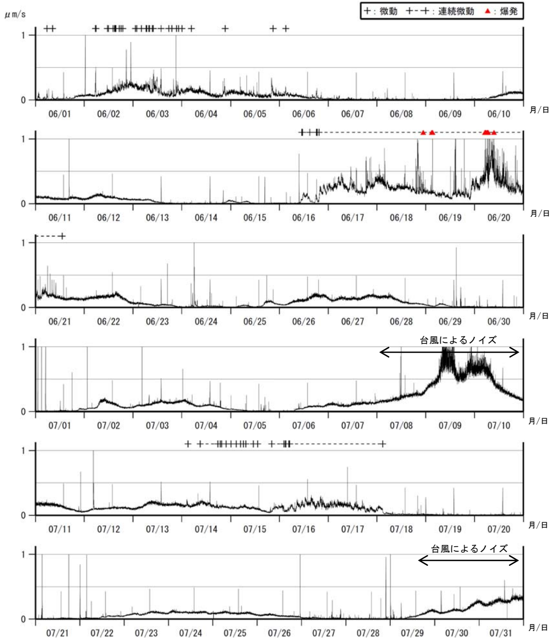
図4 諏訪之瀬島 1分間平均振幅の時間変化 （ナベタオ観測点上下動成分）（2014年6～7月）
