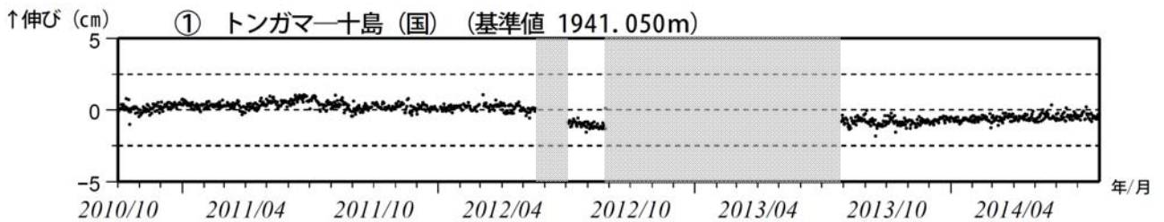
図5 諏訪之瀬島 GNSS連続観測による基線長変化（2010年10月～2014年7月）
