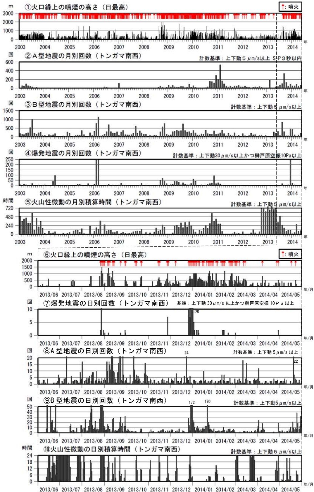
図3 諏訪之瀬島 火山活動経過図（2003年1月～2014年5月）
