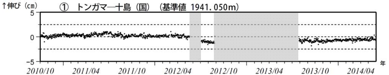
図5 諏訪之瀬島 GNSS連続観測による基線長変化（2010年10月～2014年5月）
