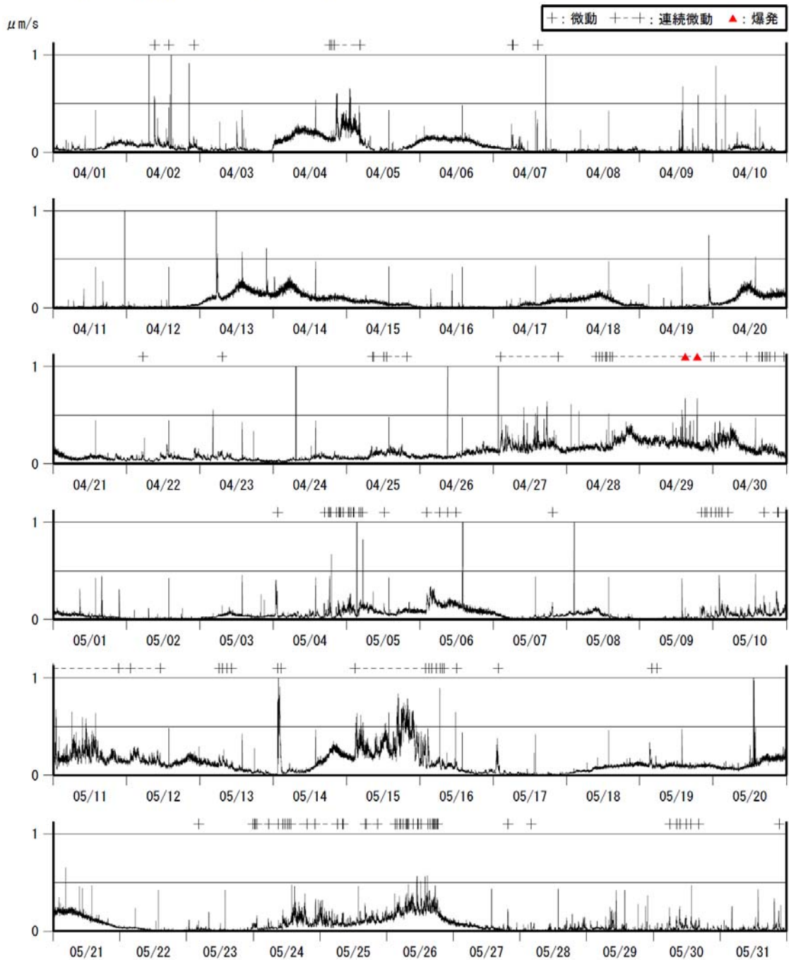
図4 諏訪之瀬島 1分間平均振幅の時間変化 (ナベタオ観測点上下動成分) (2014年4月～5月)
