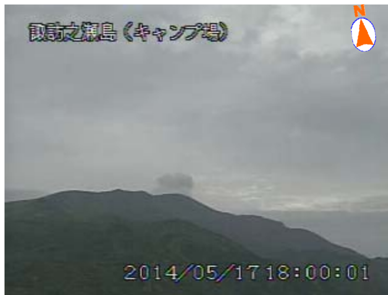
図 1 諏訪之瀬島 噴煙の状況 （5 月 17 日、諏訪之瀬島キャンプ場遠望カメラによる）
