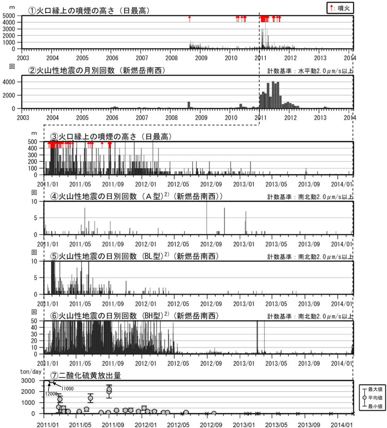
図 4 霧島山（新燃岳） 火山活動経過図（2003 年 1 月～2014 年 2 月）
