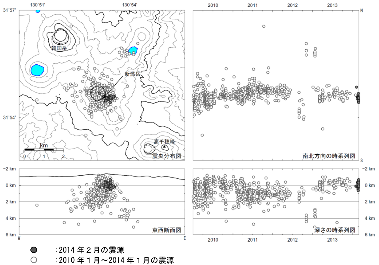
図 2 霧島山（新燃岳） 震源分布図（2010 年 1 月～2014 年 2 月）
