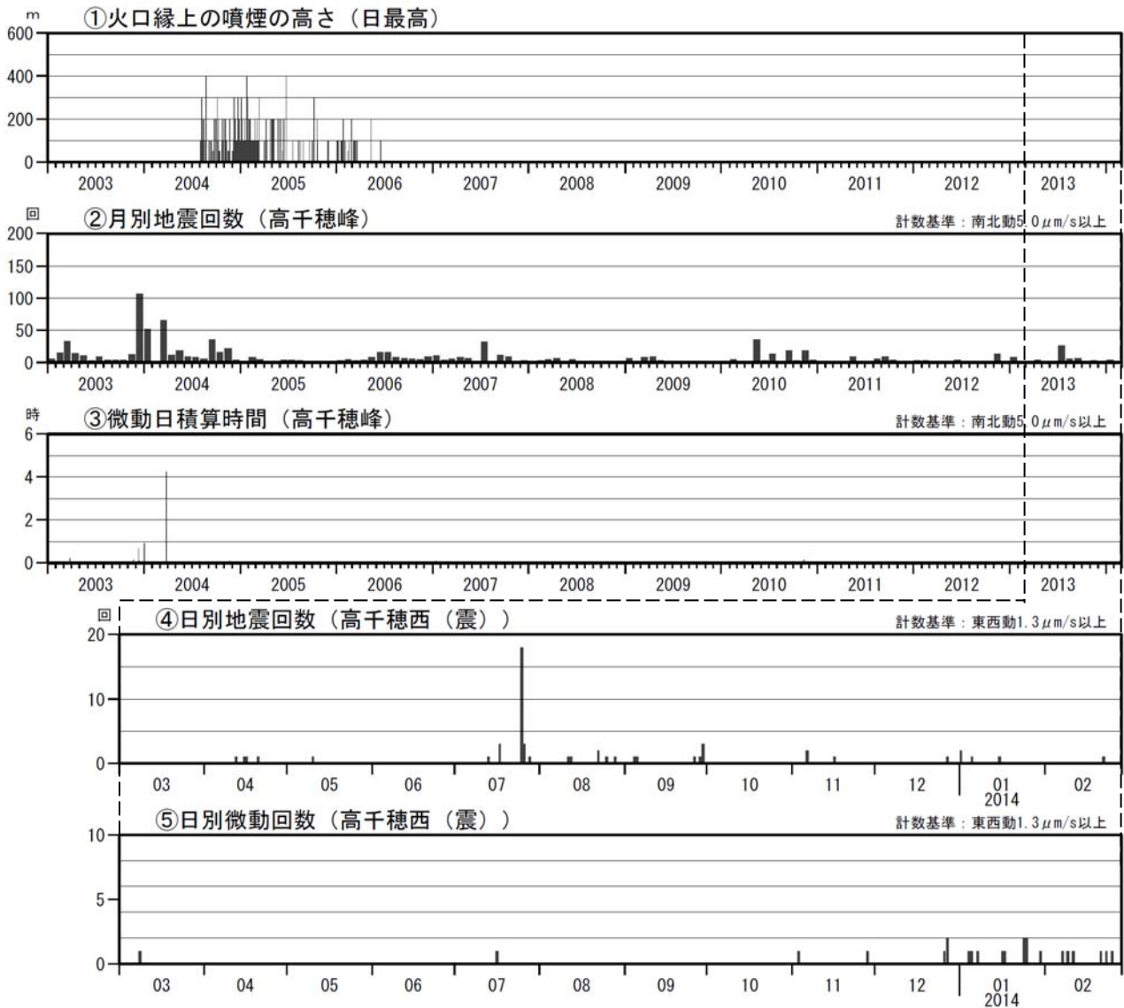
図 12 霧島山（御鉢） 火山活動経過図（2003 年 1 月～2014 年 2 月）
