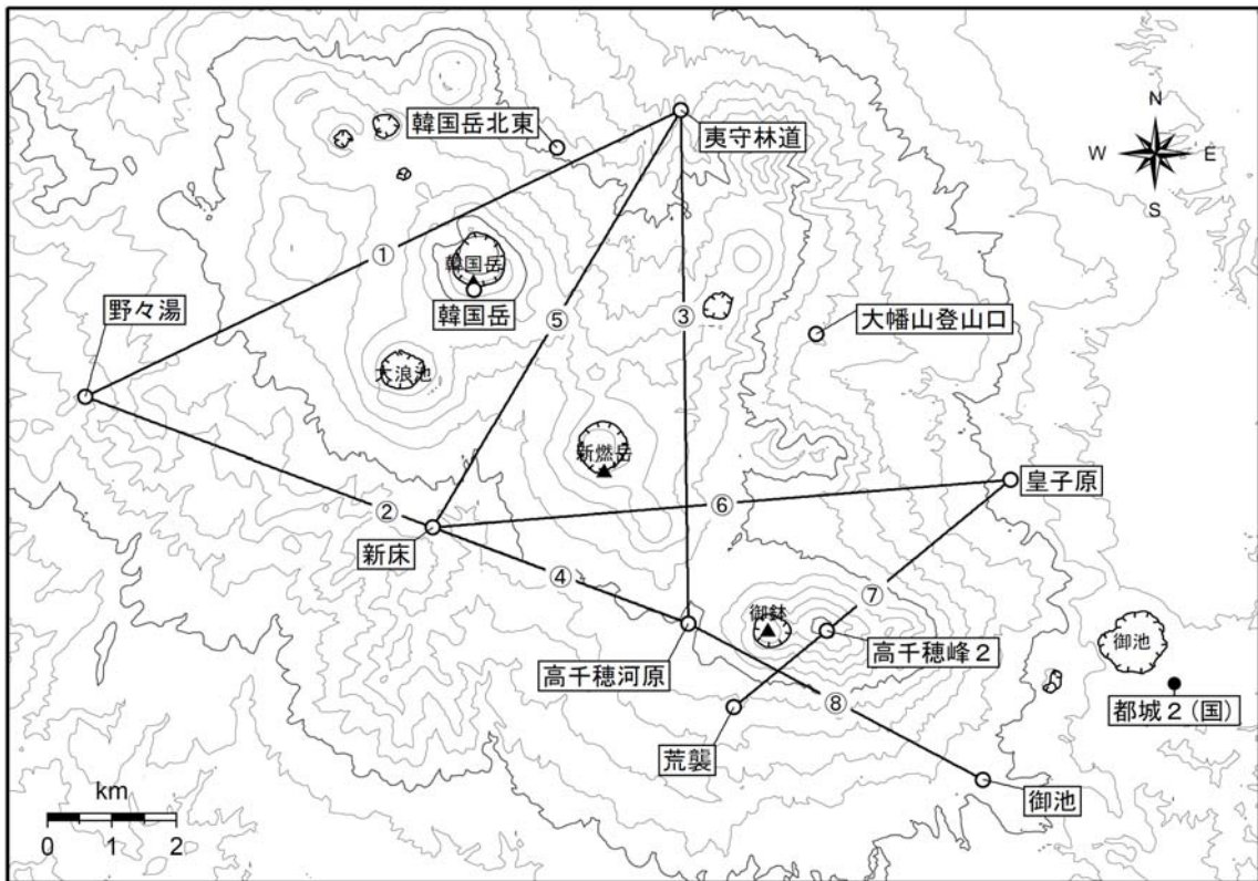
図 8 霧島山 GNSS 連続観測点と基線番号
