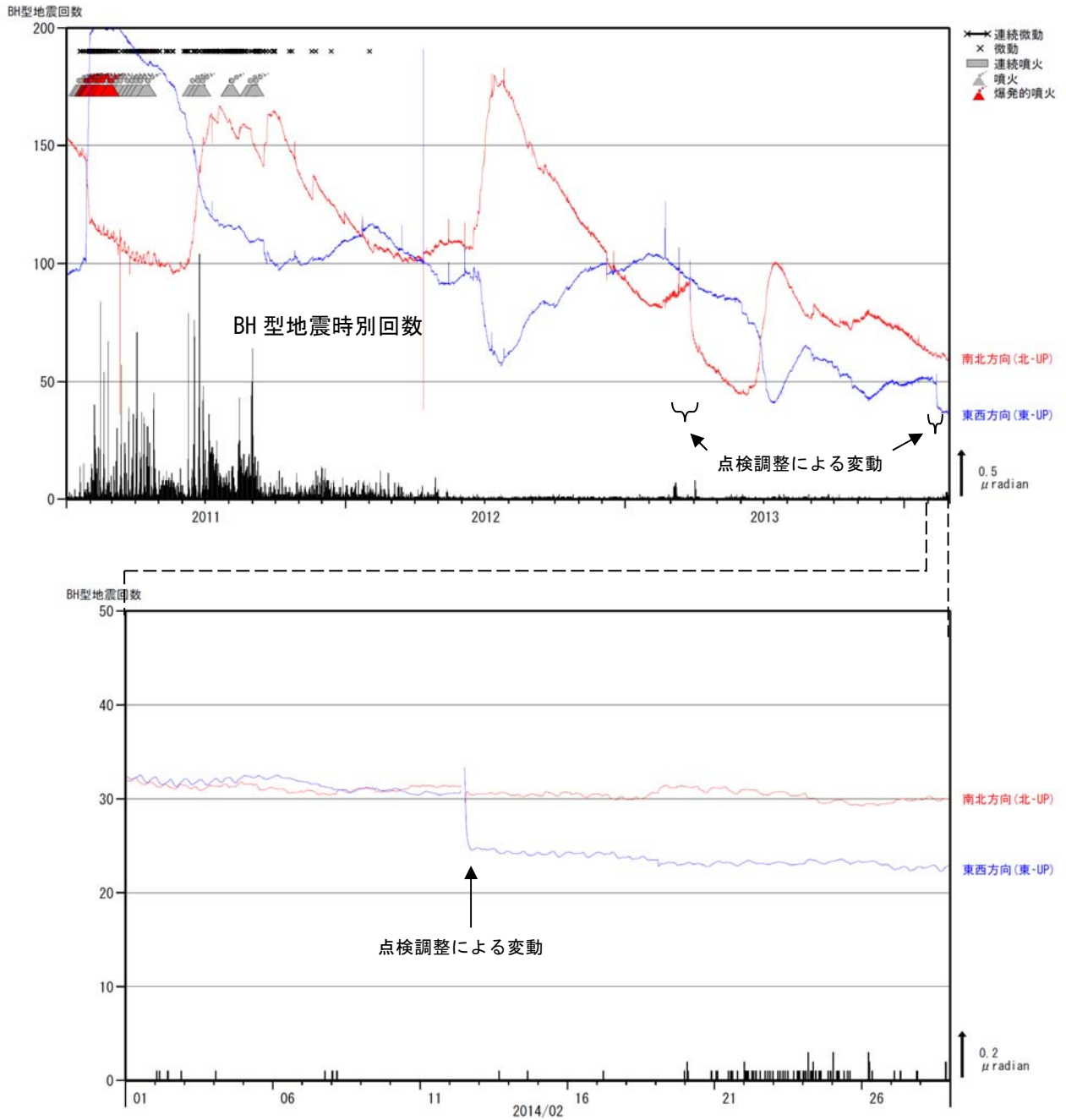
図5 霧島山（新燃岳） BH型地震の時間別回数と高千穂河原傾斜計の傾斜変動（2011年1月～2014年2月）
