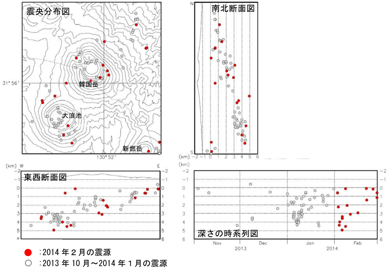
図 10 霧島山（韓国岳、大浪池付近） 震源分布図（2013 年 10 月～2014 年 2 月）
