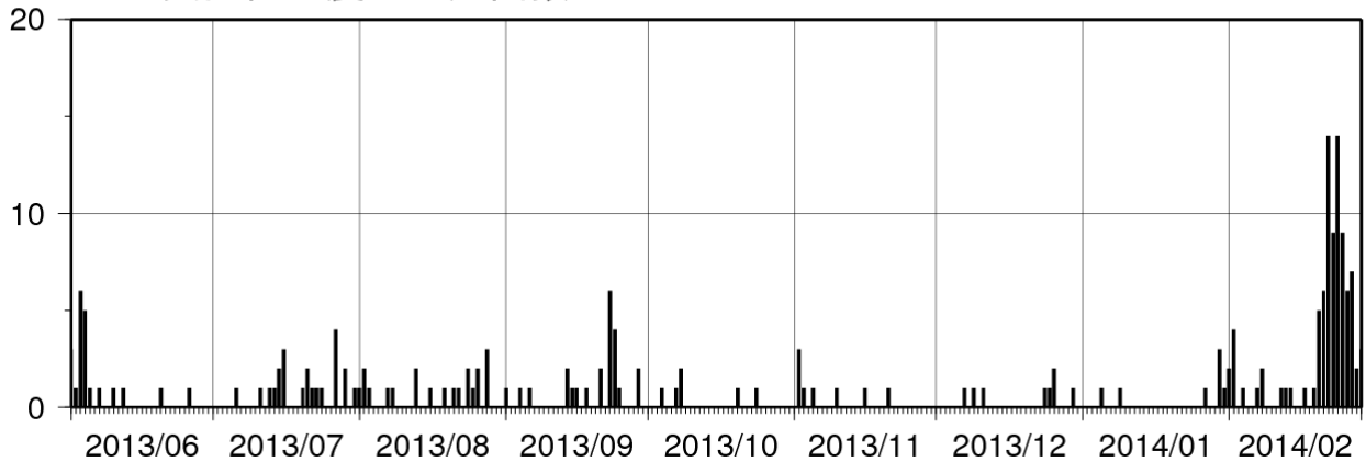
図 3 霧島山（新燃岳） 火山性地震の日別回数（2013 年 6 月～2014 年 2 月）
