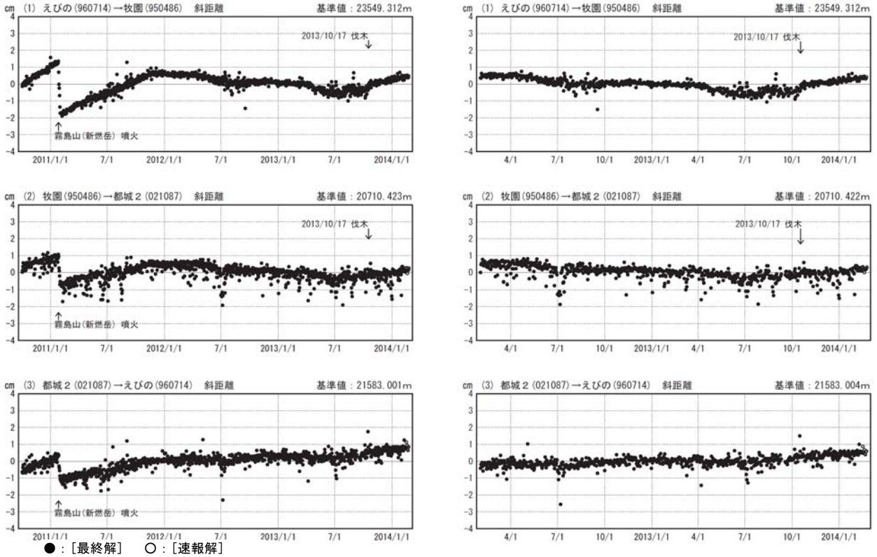
図 6 霧島山（新燃岳） 国土地理院による広域的な地殻変動観測結果* (2010 年 10 月 1 日～2014 年 2 月 23 日)
