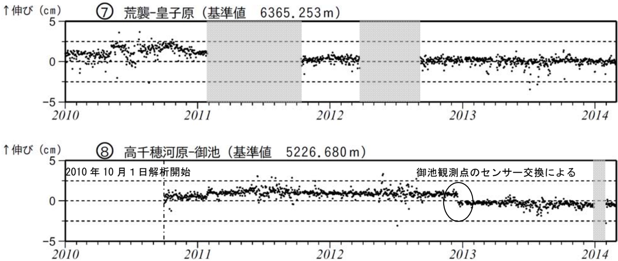
図 7-2 霧島山 GNSS 連続観測による長期の基線長変化（2010 年 1 月～2014 年 2 月）
