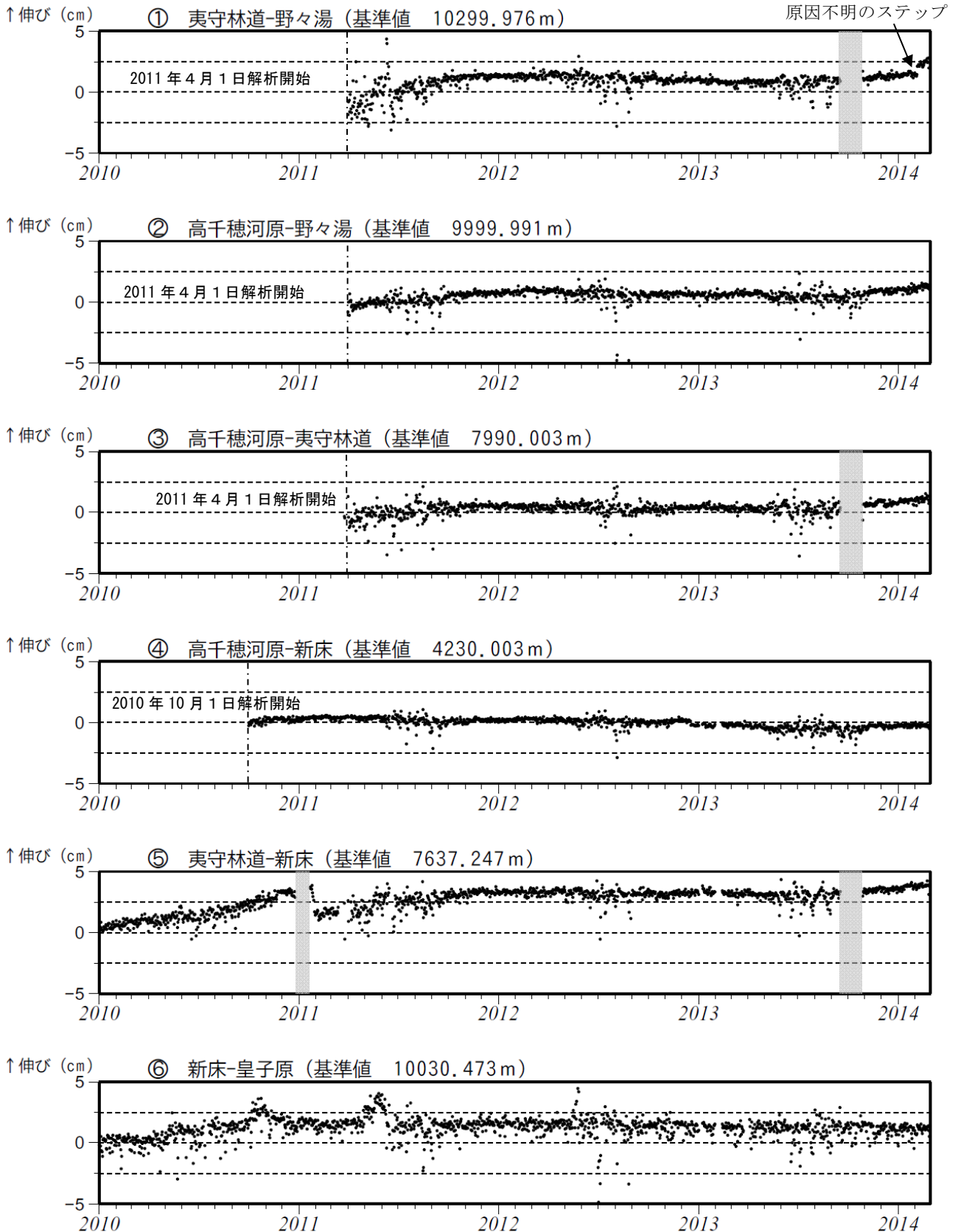
図 7-1 霧島山 GNSS 連続観測による長期の基線長変化（2010 年 1 月～2014 年 2 月）
