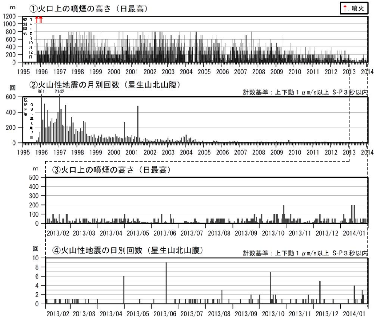
図2 九重山 火山活動経過図（1995年10月～2014年1月）
