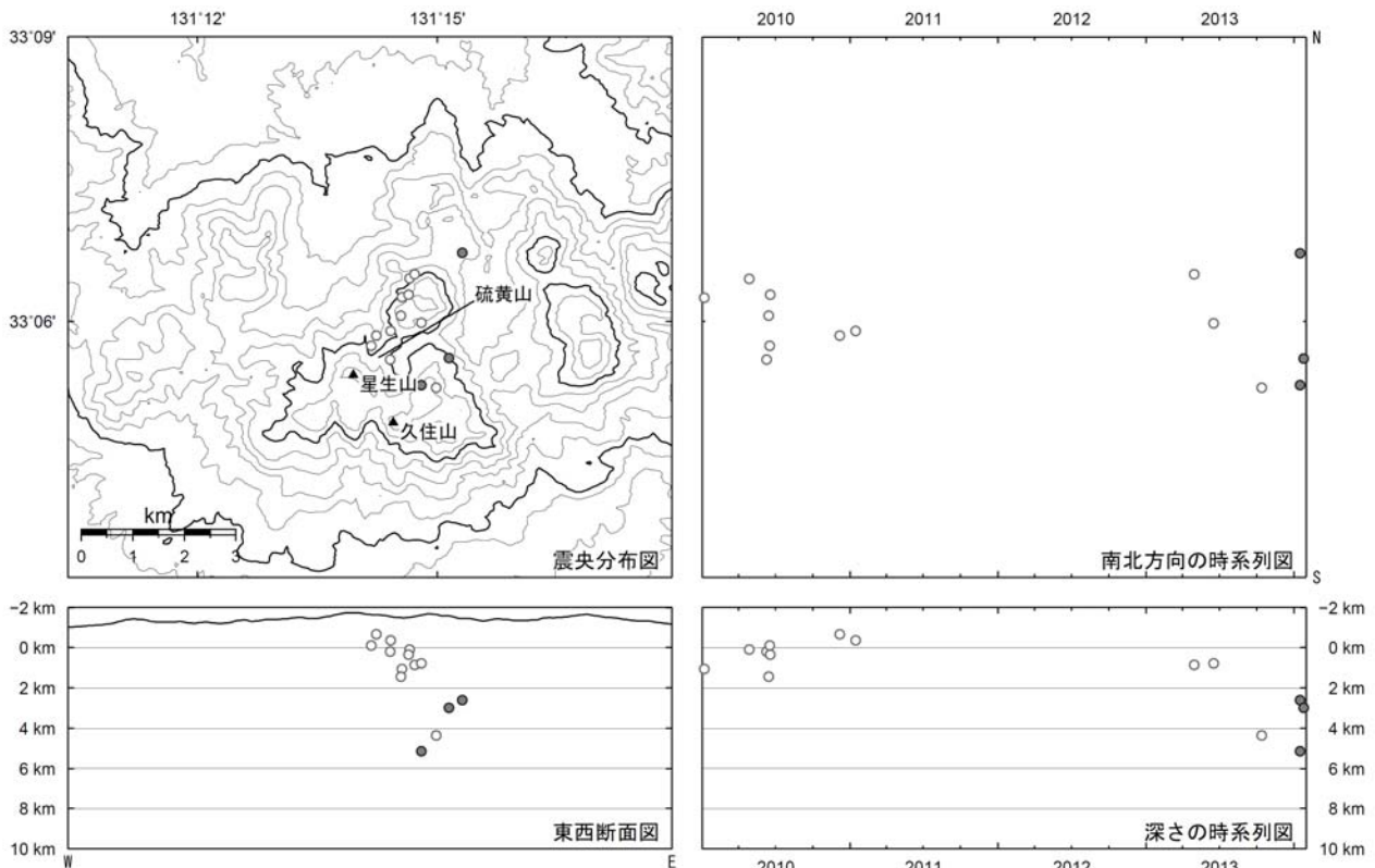
図3 九重山 震源分布図（2010 年 1 月～2014 年 1 月）
