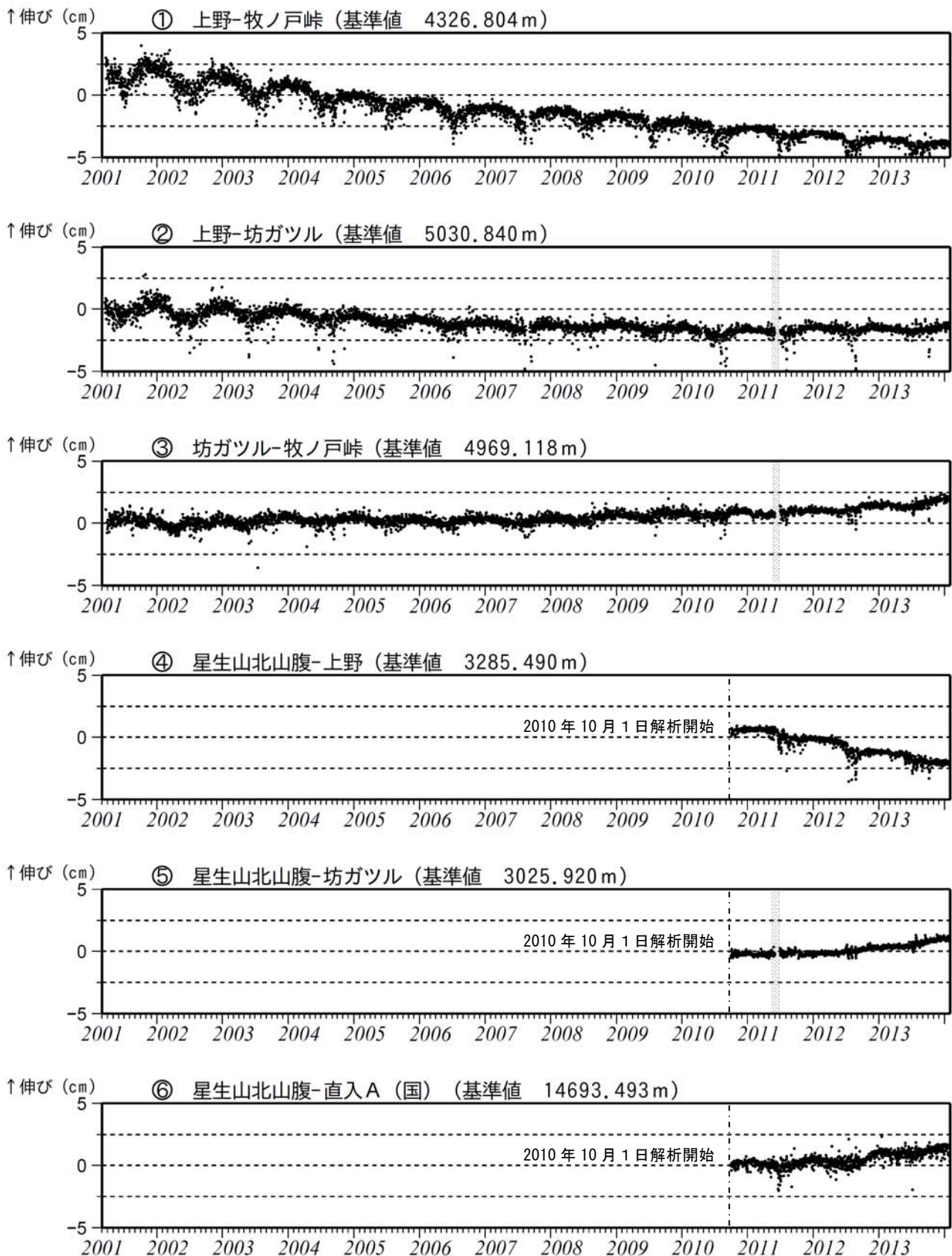
図 5 九重山 GPS 連続観測による基線長変化 (2001 年 3 月～2014 年 1 月)
