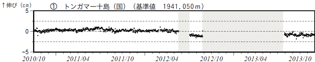
図 5 諏訪之瀬島 GPS連続観測による基線長変化（2010 年 10 月～2013 年 11 月） 火山活動によると考えられる変化は認められませんでした。
