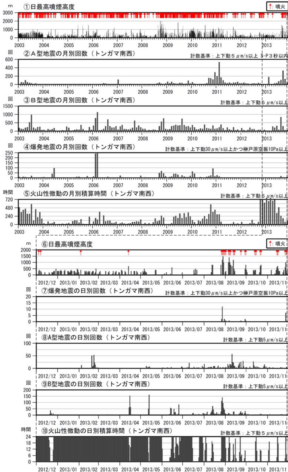
図3 諏訪之瀬島 火山活動経過図（2003年1月～2013年11月）
