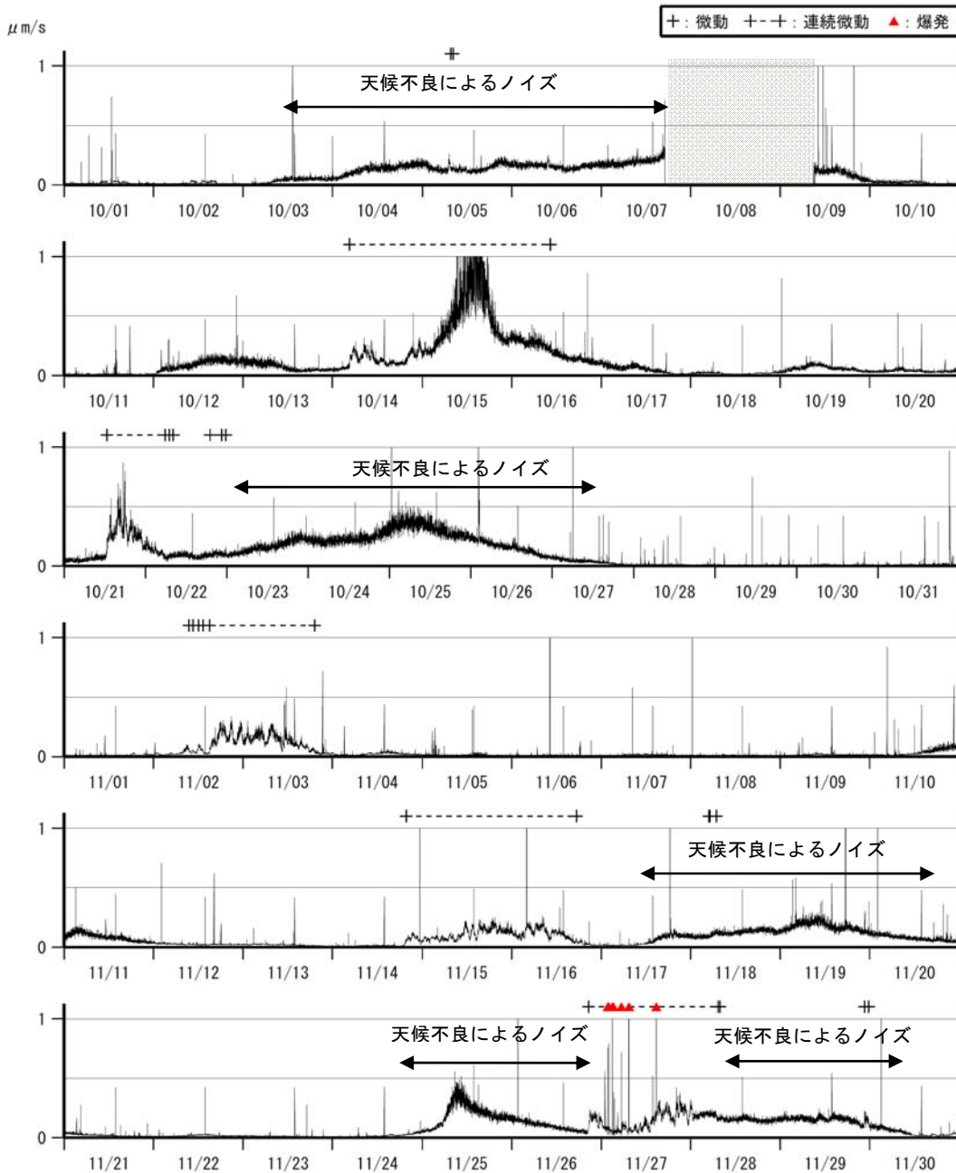
図 4 諏訪之瀬島 1 分間平均振幅の時間変化（ナベタオ観測点上下動成分）（2013 年 10～11 月） <11 月の状況>
