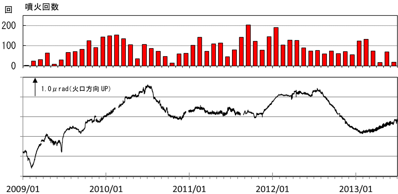
図 7 桜島 有村観測坑道の水管傾斜計（大隅河川国道事務所設置）の変化 (2009 年 1 月～2013 年 6 月)
