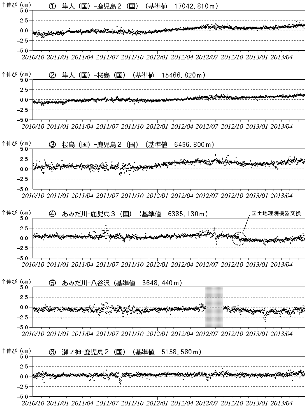
図 8-1 桜島 GPS 連続観測による長期の基線長変化（2010 年 10 月～2013 年 6 月）
