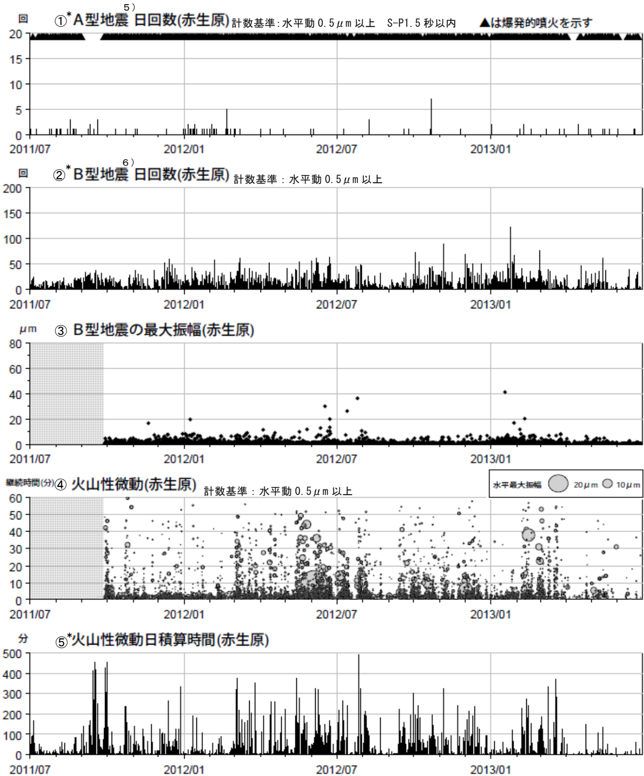
図5 桜島 最近2年間の火山性地震、火山性微動 (2011年7月~2013年6月)
