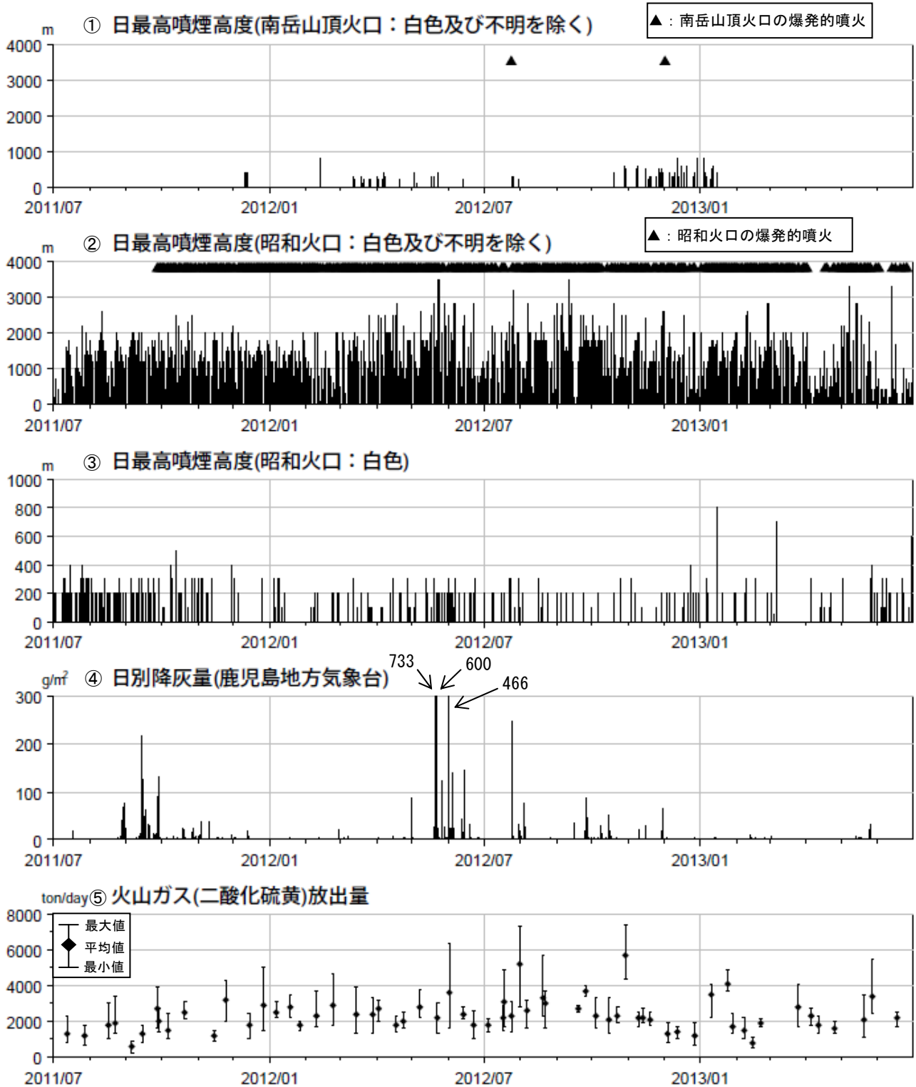
図 4 桜島 最近 2 年間の噴煙、降灰、火山ガス（2011 年 7 月～2013 年 6 月）
