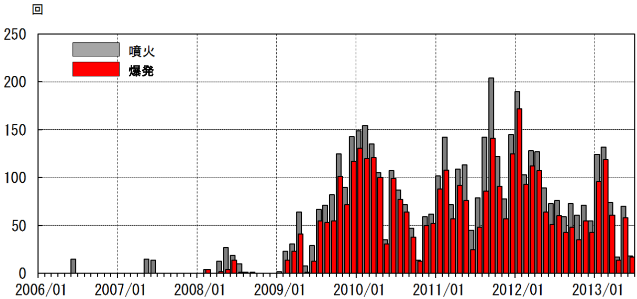
図2 桜島 昭和火口月別噴火回数（灰色）と昭和火口月別爆発回数（赤色） (2006年1月～2013年6月)
