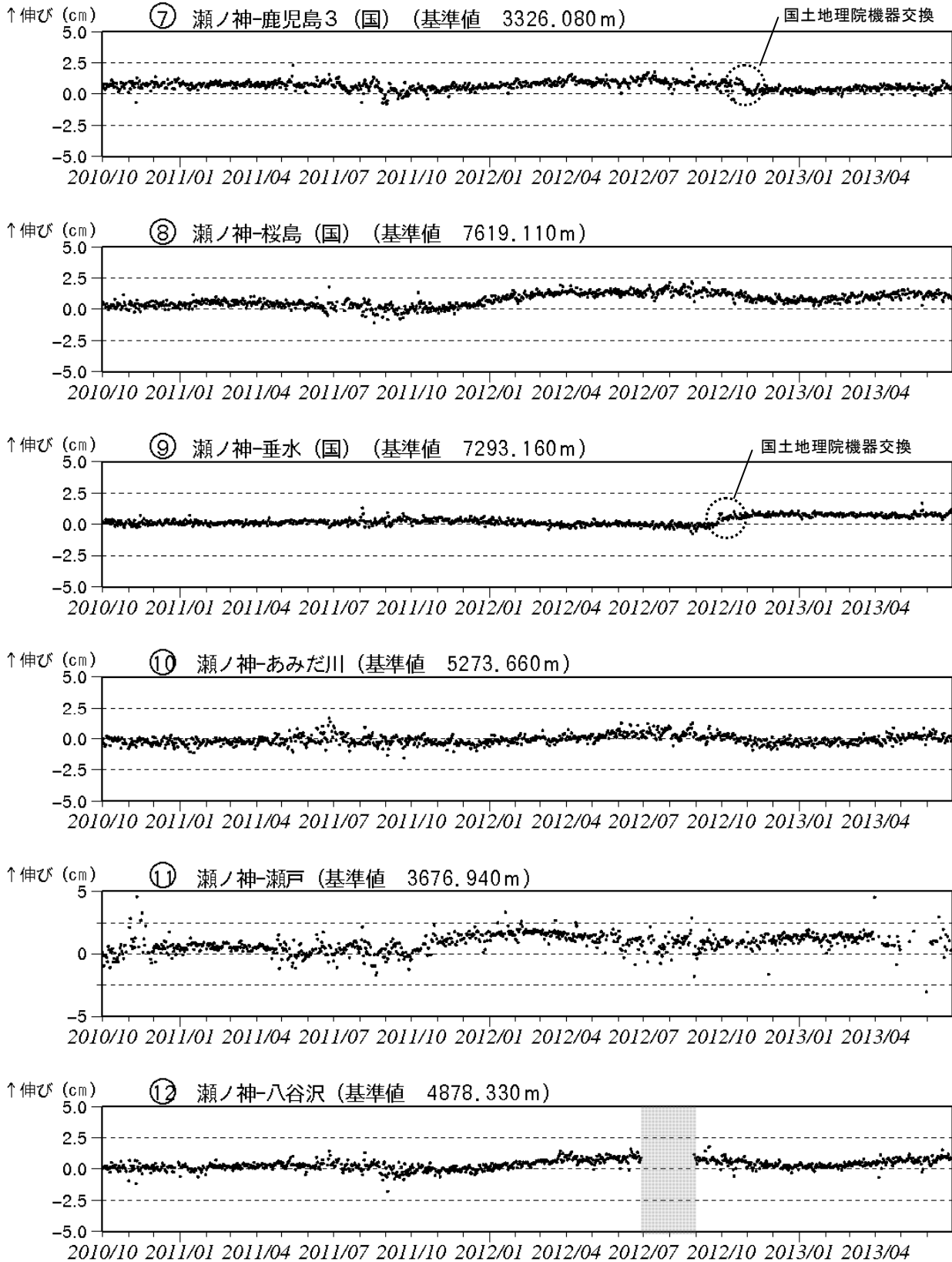
図 8-2 桜島 GPS 連続観測による長期の基線長変化（2010 年 10 月～2013 年 6 月）
