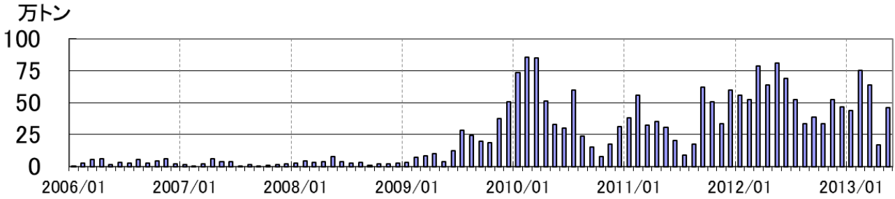
図 10 桜島 鹿児島県が実施している降灰の観測データから推定した火山灰の月別総噴出量 (2006 年 1 月～2013 年 5 月)
