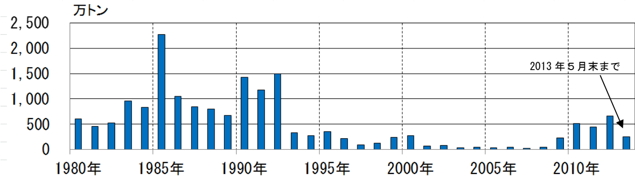
図 11 桜島 鹿児島県が実施している降灰の観測データから推定した火山灰の年別総噴出量 (1980 年～2013 年)
