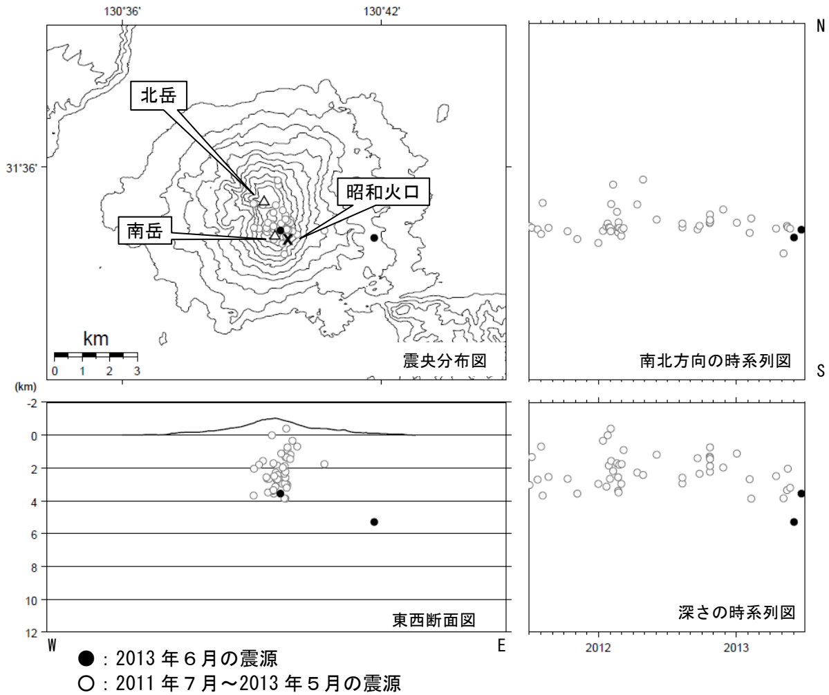
● : 2013 年 6 月の震源 ○ : 2011 年 7 月～2013 年 5 月の震源 図 6 桜島 震源分布図 (2011 年 7 月～2013 年 6 月) < 6 月の状況 >
