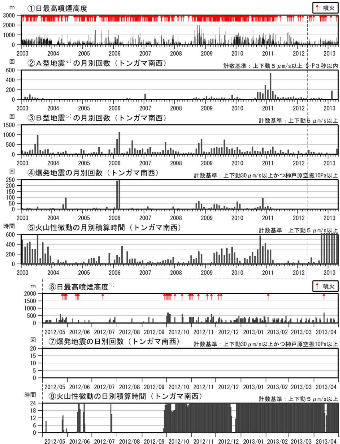
図3 諏訪之瀬島 火山活動経過図（2003年1月～2013年4月）
