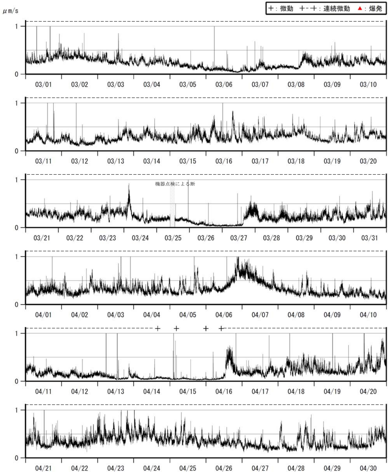
図 4 諏訪之瀬島 1 分間平均振幅の時間変化（ナベタオ上下成分）（2013 年 3 月～2013 年 4 月） < 4 月の状況 >
