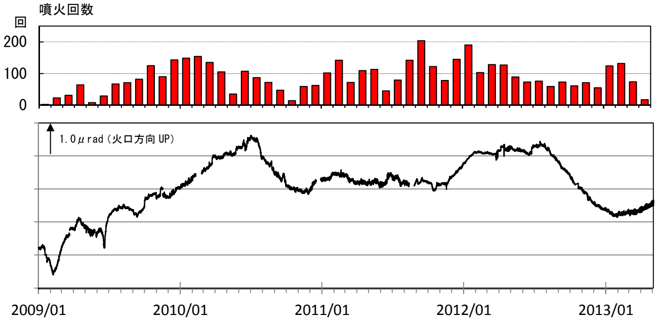
図 8※ 桜島 有村観測坑道の水管傾斜計（大隅河川国道事務所設置）の変化 （2009 年 1 月～2013 年 4 月）
