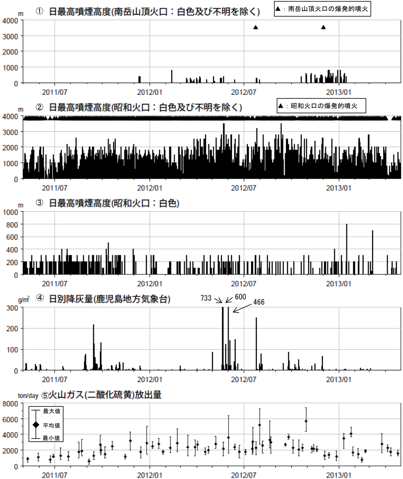
図3 桜島 最近2年間の噴煙、降灰、火山ガス（2011年5月～2013年4月）
