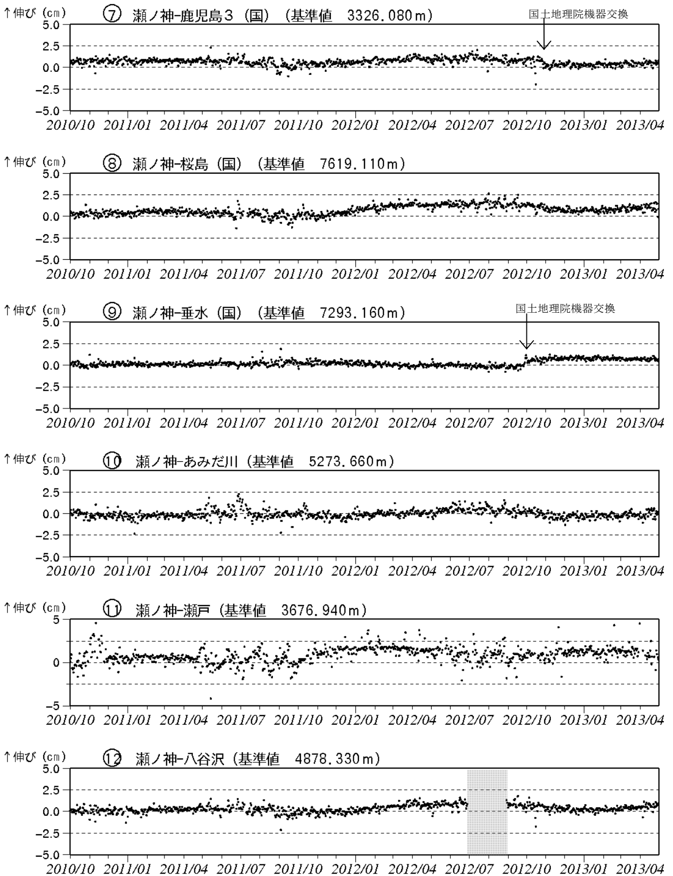
図 6-2* 桜島 GPS 連続観測による長期の基線長変化（2010 年 10 月～2013 年 4 月）
