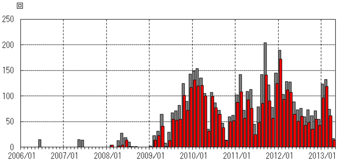
図 2 桜島 昭和火口月別噴火回数（灰色）と昭和火口月別爆発回数（赤色）
