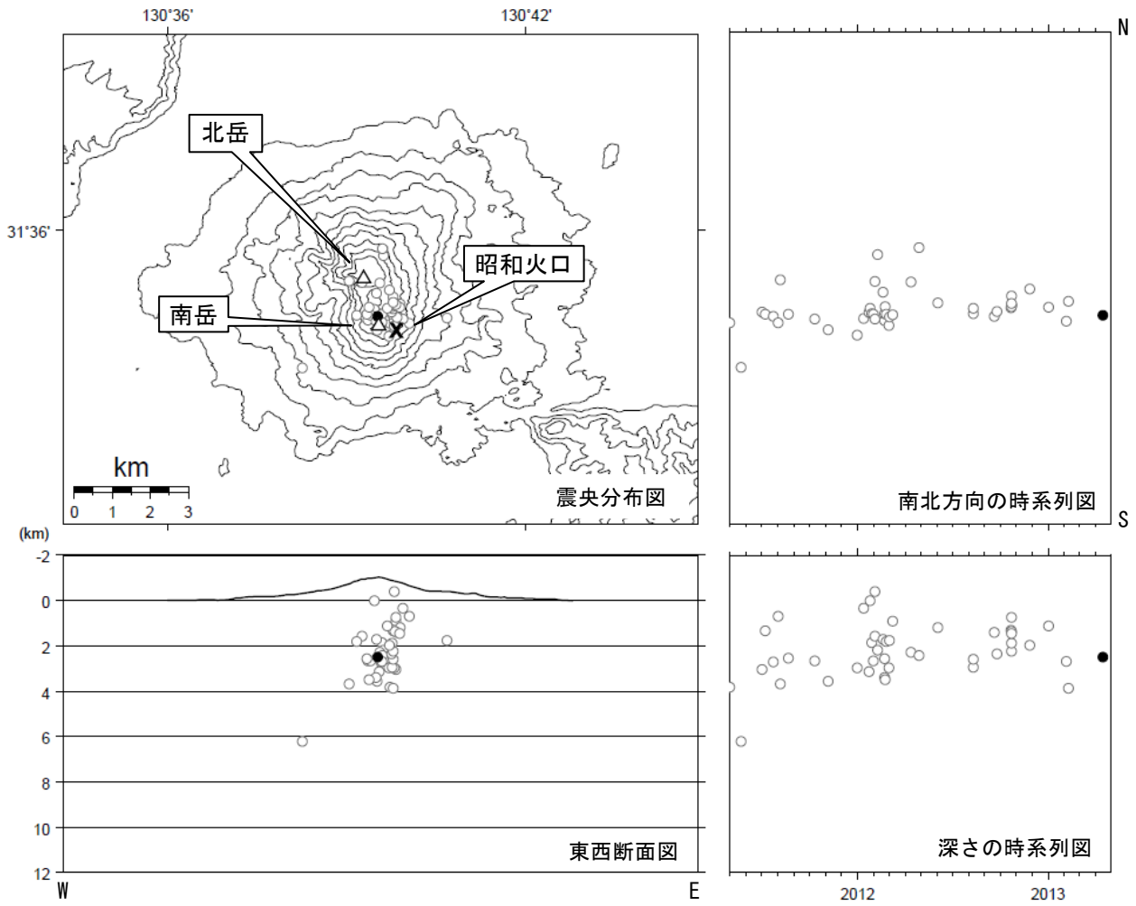
● : 2013 年 4 月の震源 ○ : 2011 年 5 月～2013 年 3 月の震源 図 5※ 桜島 震源分布図 (2011 年 5 月～2013 年 4 月) < 4 月の状況 > 震源は、南岳直下の海拔下 2 km 付近でした。
