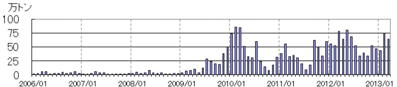
図 9※ 桜島 鹿児島県が実施している降灰の観測データから推定した火山灰の月別総噴出量 （2006 年 1 月～2013 年 3 月）
