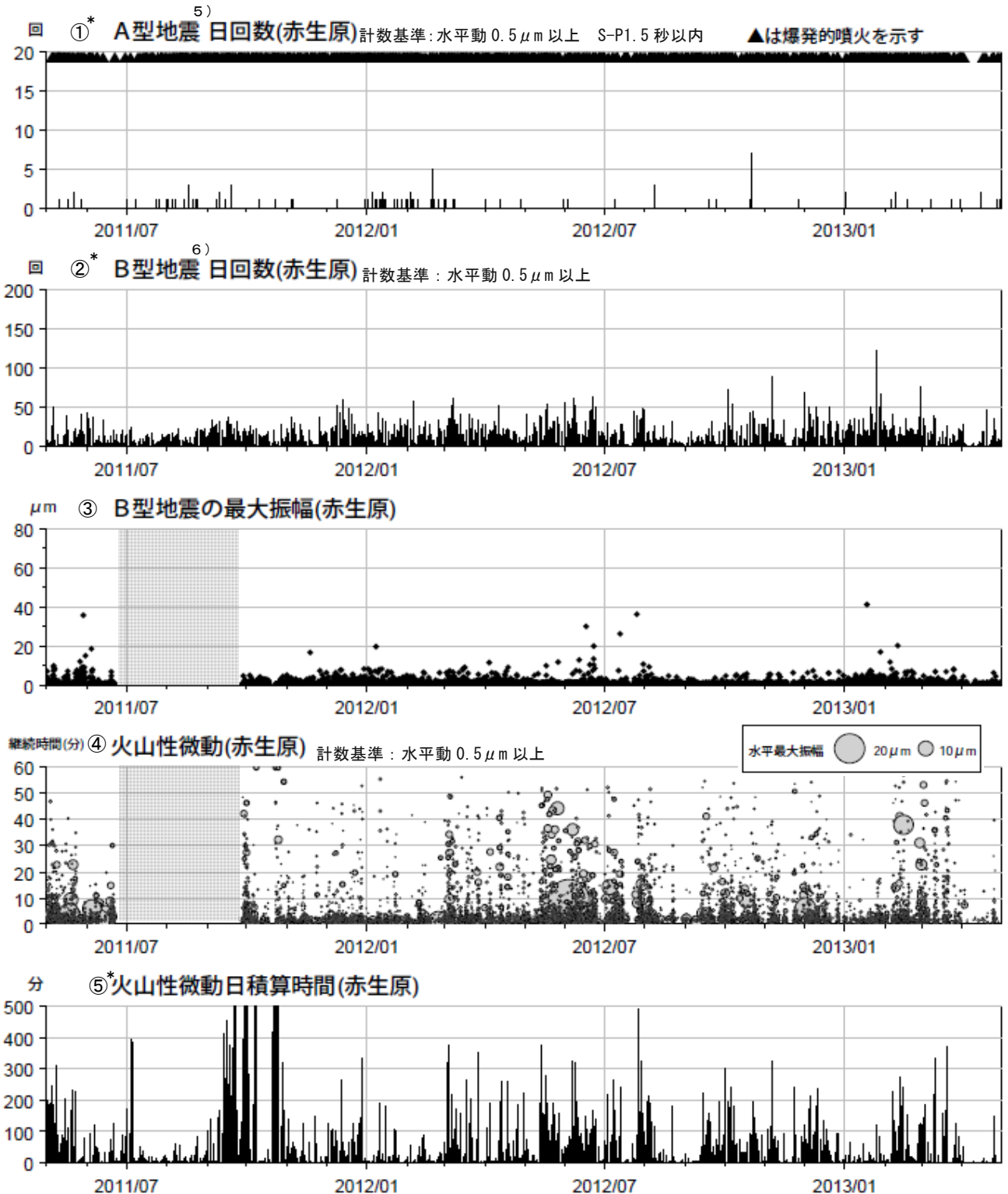
図4 桜島 最近2年間の火山性地震、火山性微動（2011年5月～2013年4月）
