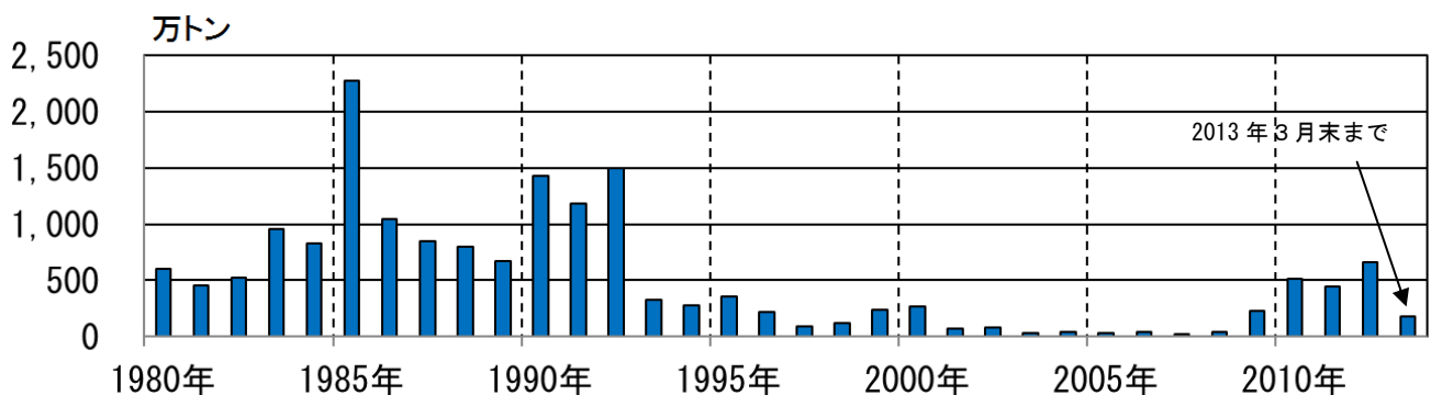
図 10※ 桜島 鹿児島県が実施している降灰の観測データから推定した火山灰の年別総噴出量 （1980 年～2013 年）
