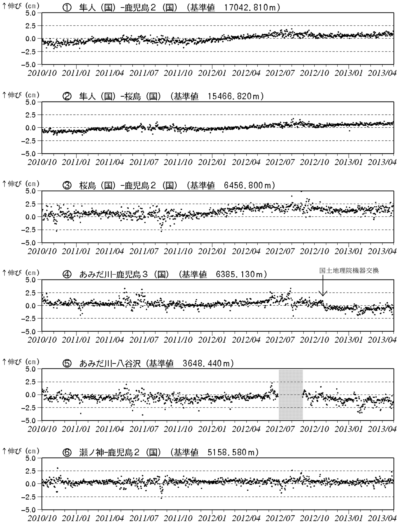
図 6-1※ 桜島 GPS 連続観測による長期の基線長変化 (2010 年 10 月～2013 年 4 月)
