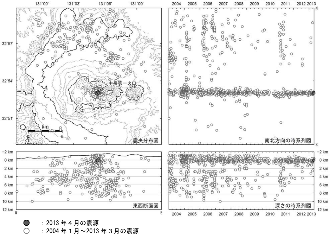
図5※ 阿蘇山 震源分布図（2004年1月～2013年4月） < 4月の状況 > 震源は、中岳第一火口付近のごく浅いところに分布しました。
