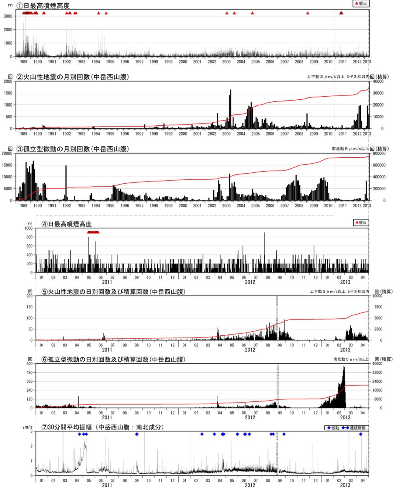
図3 阿蘇山 火山活動経過図（1989年1月～2013年4月、赤線は積算回数）
