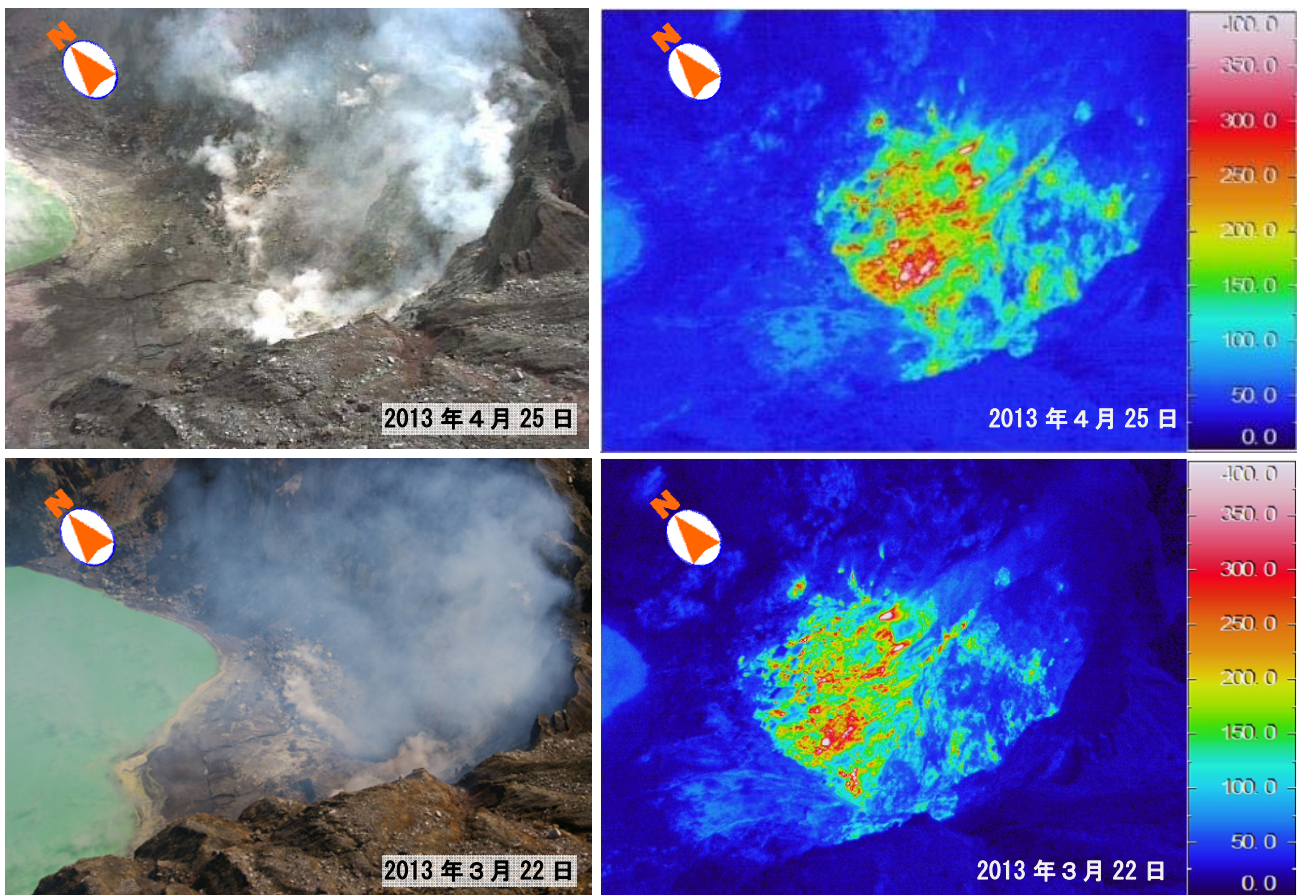
図 9 阿蘇山 赤外熱映像装置による中岳第一火口南側火口壁の地表面温度分布 （左：可視画像 右：赤外画像） （上段：4月25日撮影 下段：3月22日撮影） 温度分布に、特段の変化はありませんでした。
