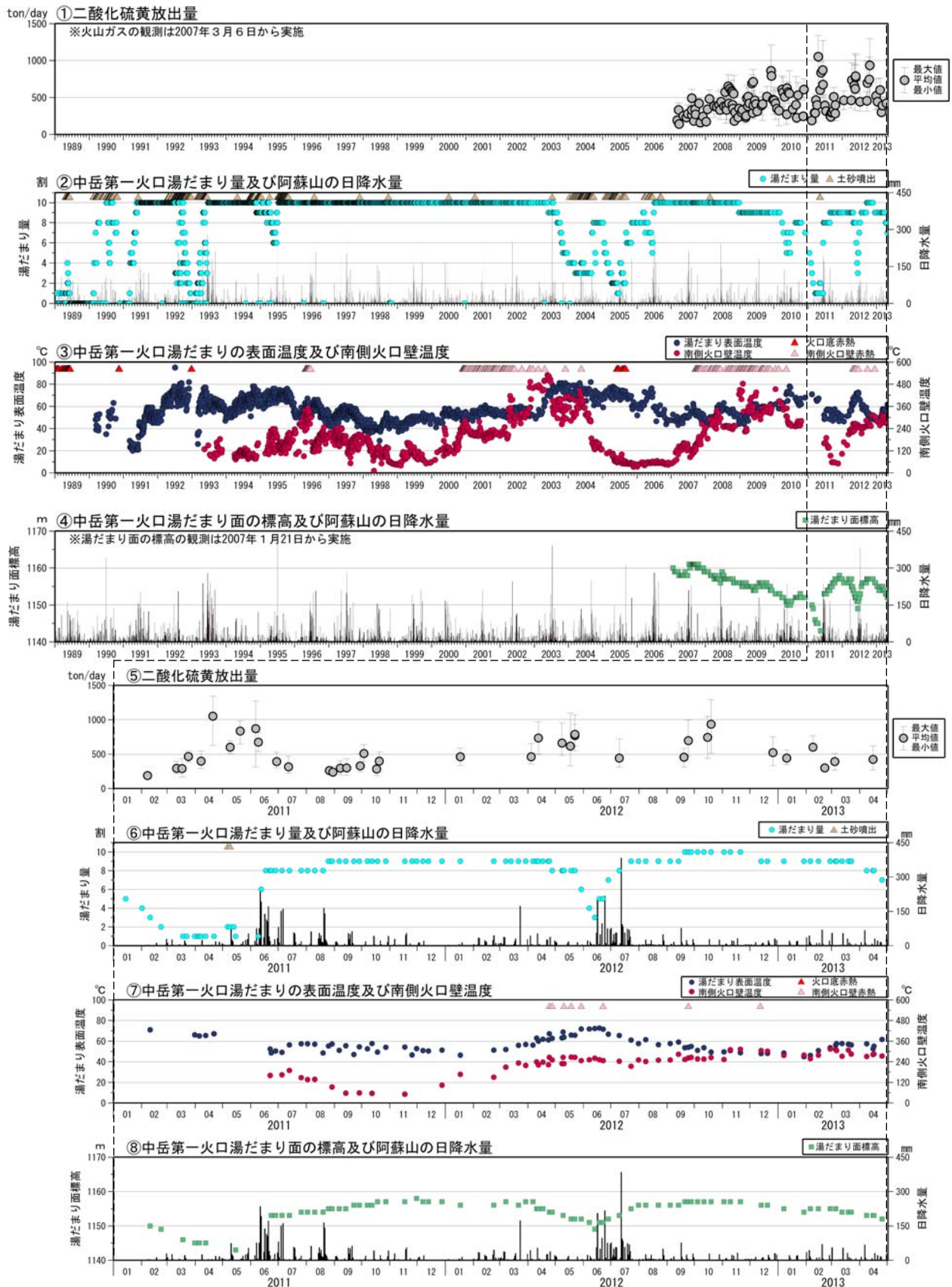
図 4 ※ 阿蘇山 湯だまり、火口壁、二酸化硫黄放出量の状況（1989 年 1 月～2013 年 4 月） < 4 月の状況 >
