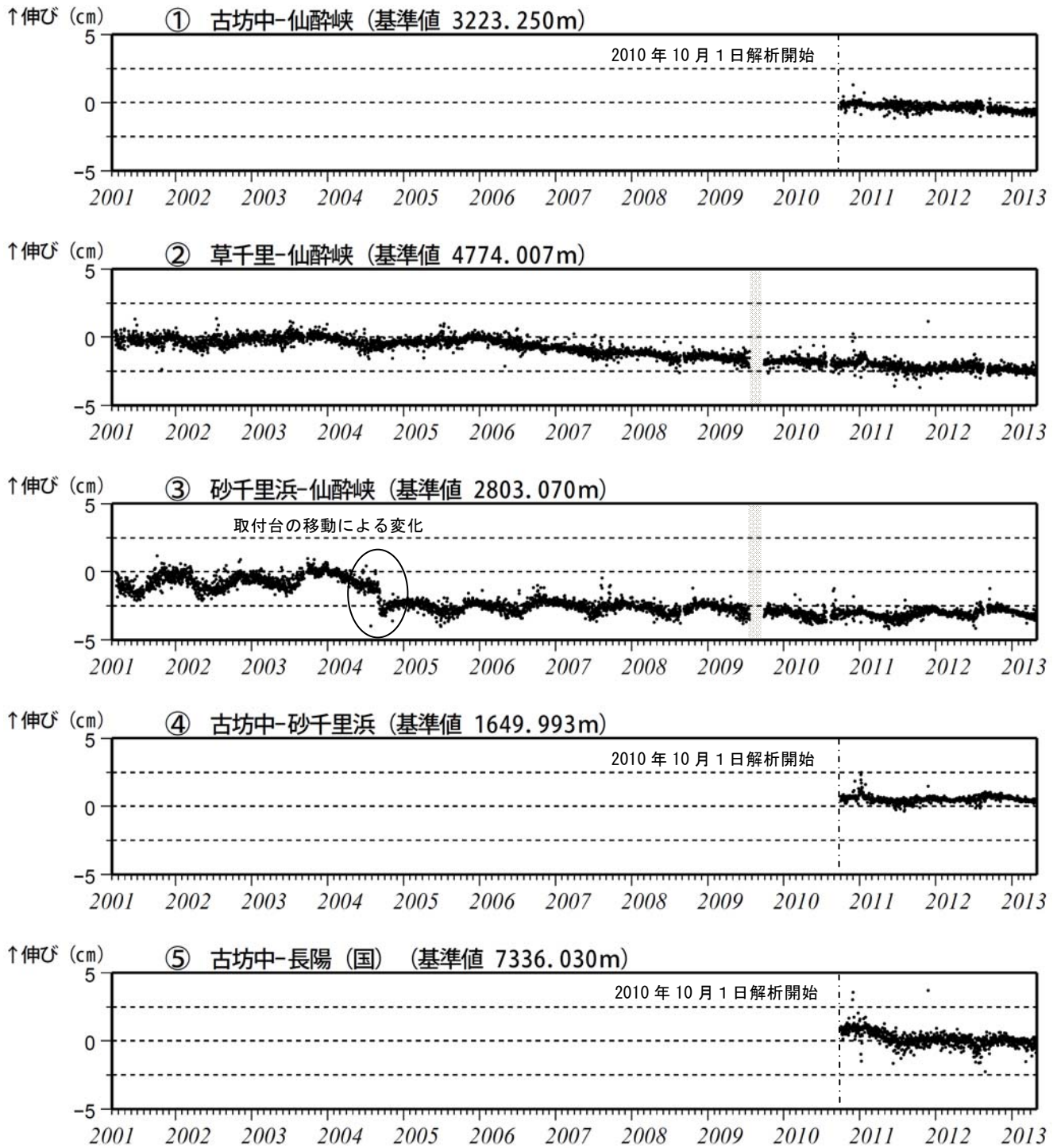
図 7※ 阿蘇山 GPS連続観測による基線長変化（2001 年 3 月～2013 年 4 月） GPS 連続観測では、火山活動によると考えられる変化は認められませんでした。
