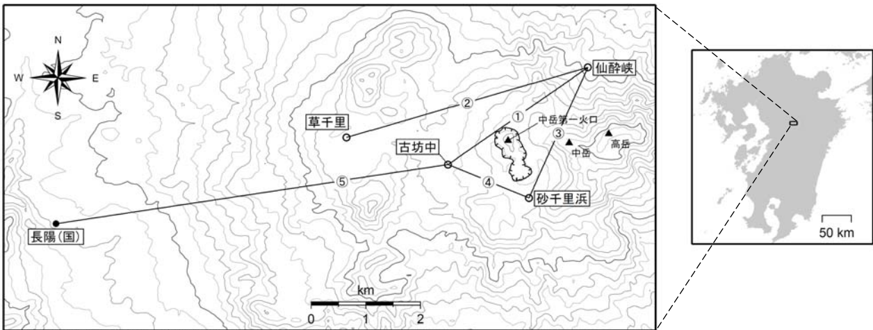
図6 阿蘇山 GPS 連続観測点と基線番号 小さな白丸（○）は気象庁、小さな黒丸（●）は気象庁以外の機関の観測点位置を示しています。 (国)：国土地理院
