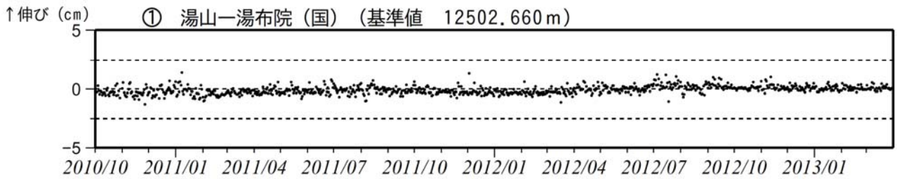
図 2※ 鶴見岳・伽藍岳 GPS連続観測による基線長変化（2010 年 10 月～2013 年 3 月） 火山活動によると考えられる変化は認められませんでした。
