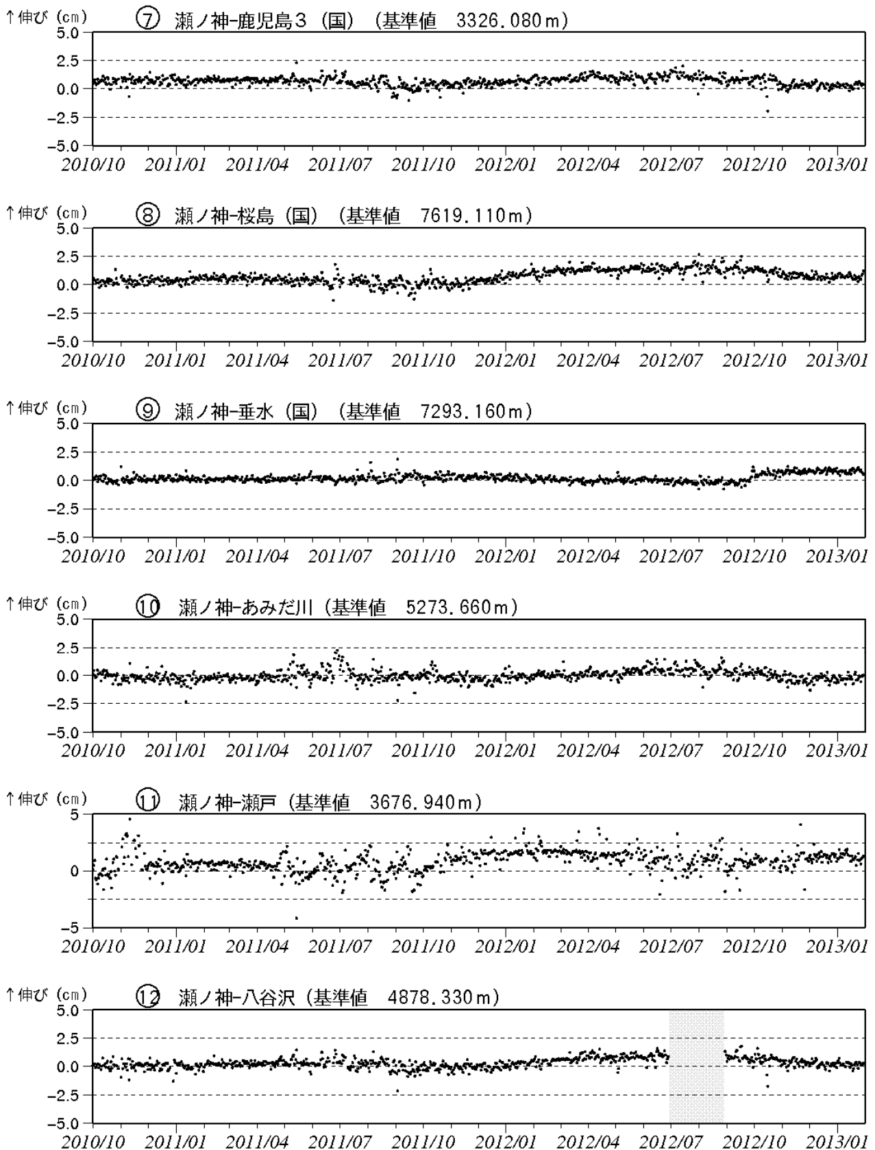
図 6-2※ 桜島 GPS 連続観測による長期の基線長変化 (2010 年 10 月～2013 年 1 月)
