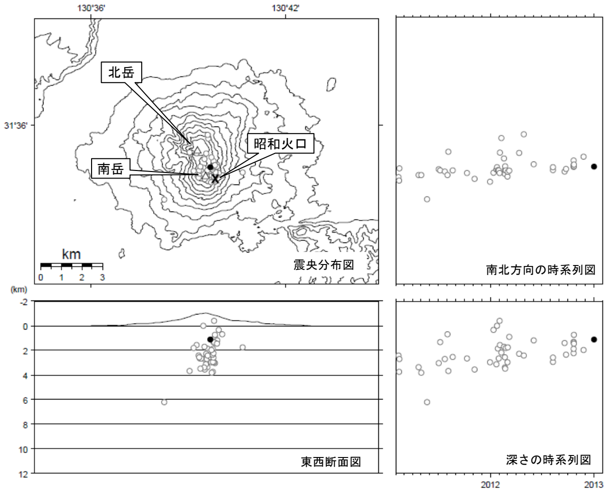
図 5※ 桜島 震源分布図（2011 年 2 月～2013 年 1 月）
