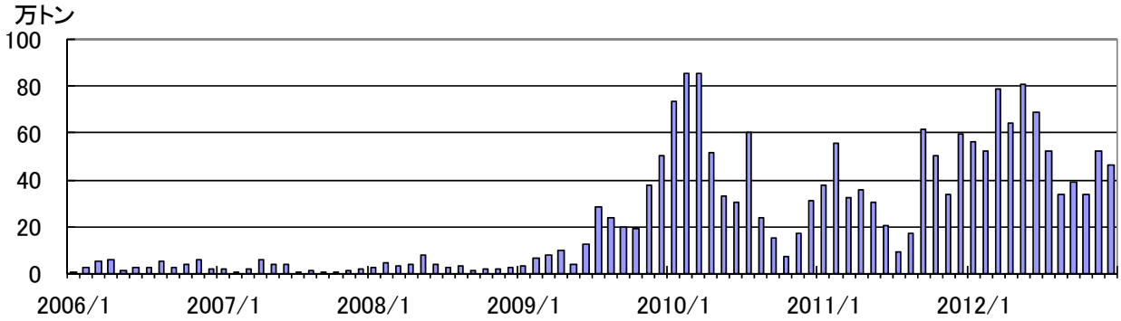
図 10※ 桜島 鹿児島県が実施している降灰の観測データから推定した火山灰の月別総噴出量（2006 年 1 月～2012 年 12 月）
