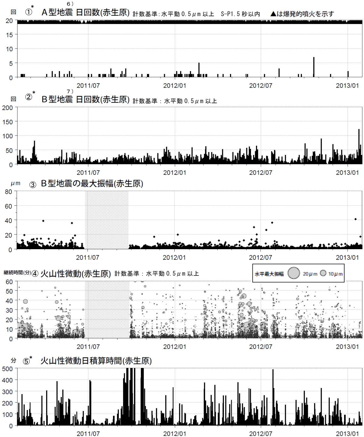
図 4 桜島 最近 2 年間の火山性地震、火山性微動（2011 年 2 月～2013 年 1 月） < 1 月の状況 >
