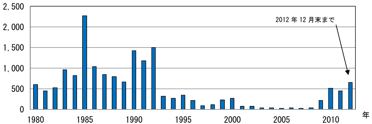
図 11※ 桜島 鹿児島県が実施している降灰の観測データから推定した火山灰の年別総噴出量（1980 年～2012 年）
