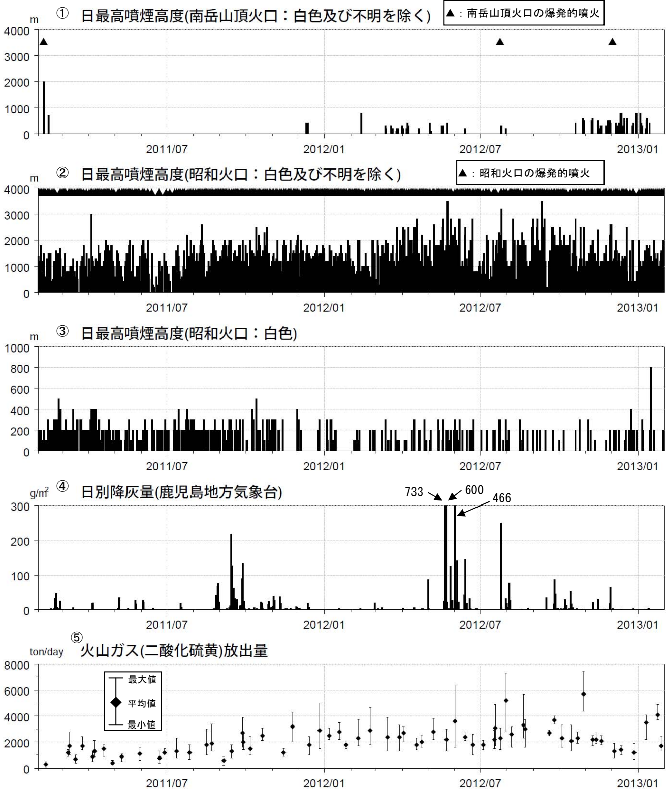
図3 桜島 最近2年間の噴煙、降灰、火山ガス（2011年2月～2013年1月） < 1月の状況 >
