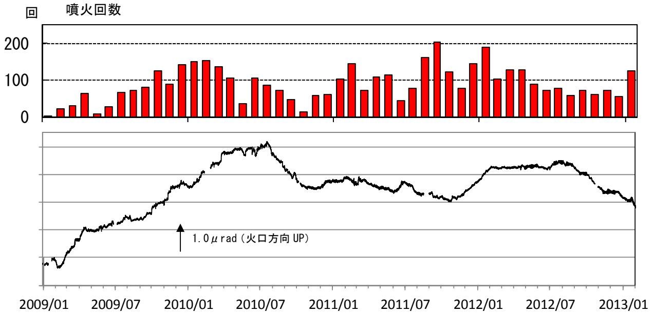
図 8※ 桜島 有村観測坑道の水管傾斜計（大隅河川国道事務所設置）の変化 （2009 年 1 月～2013 年 1 月）
