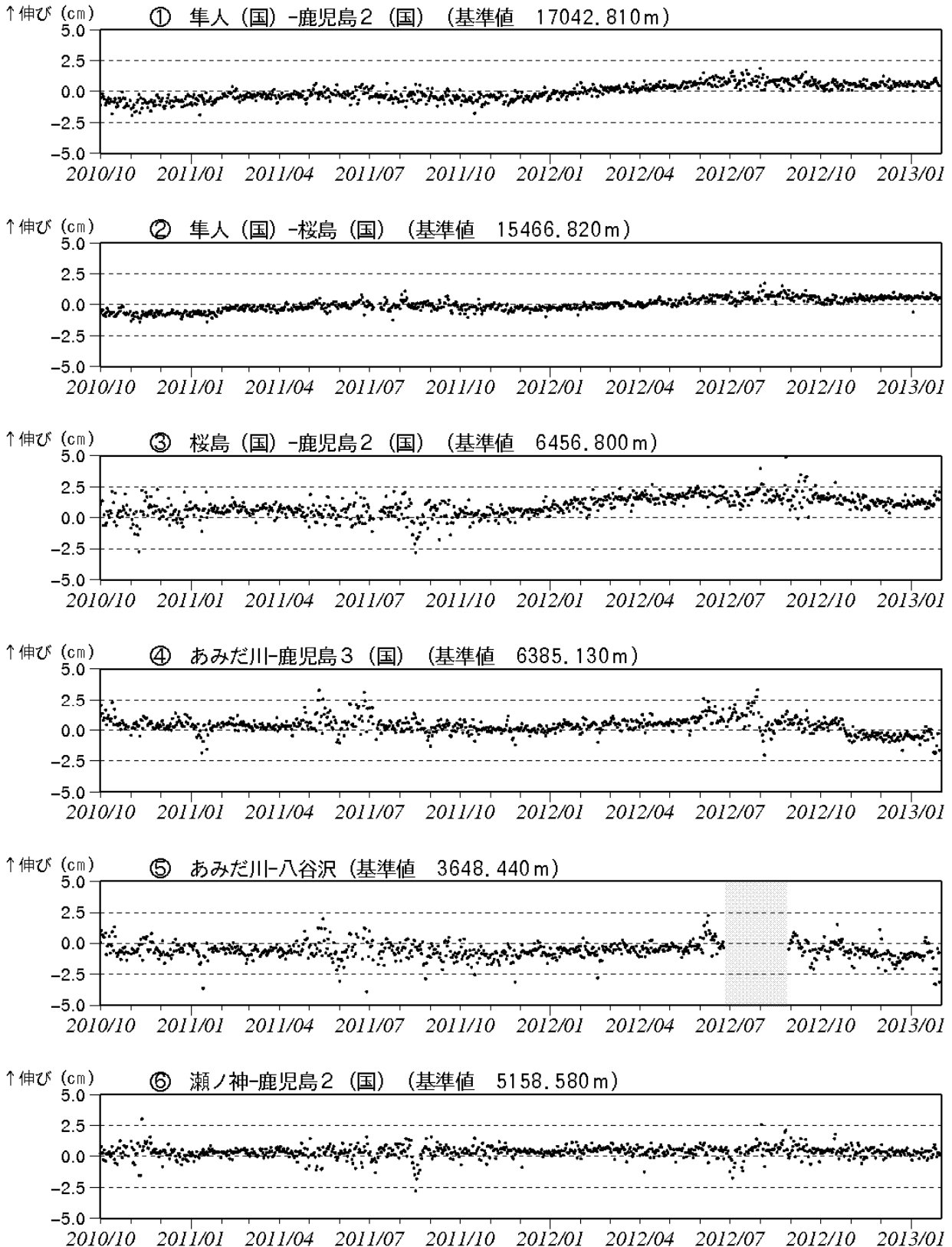
図 6-1※ 桜島 GPS 連続観測による長期の基線長変化（2010 年 10 月～2013 年 1 月）
