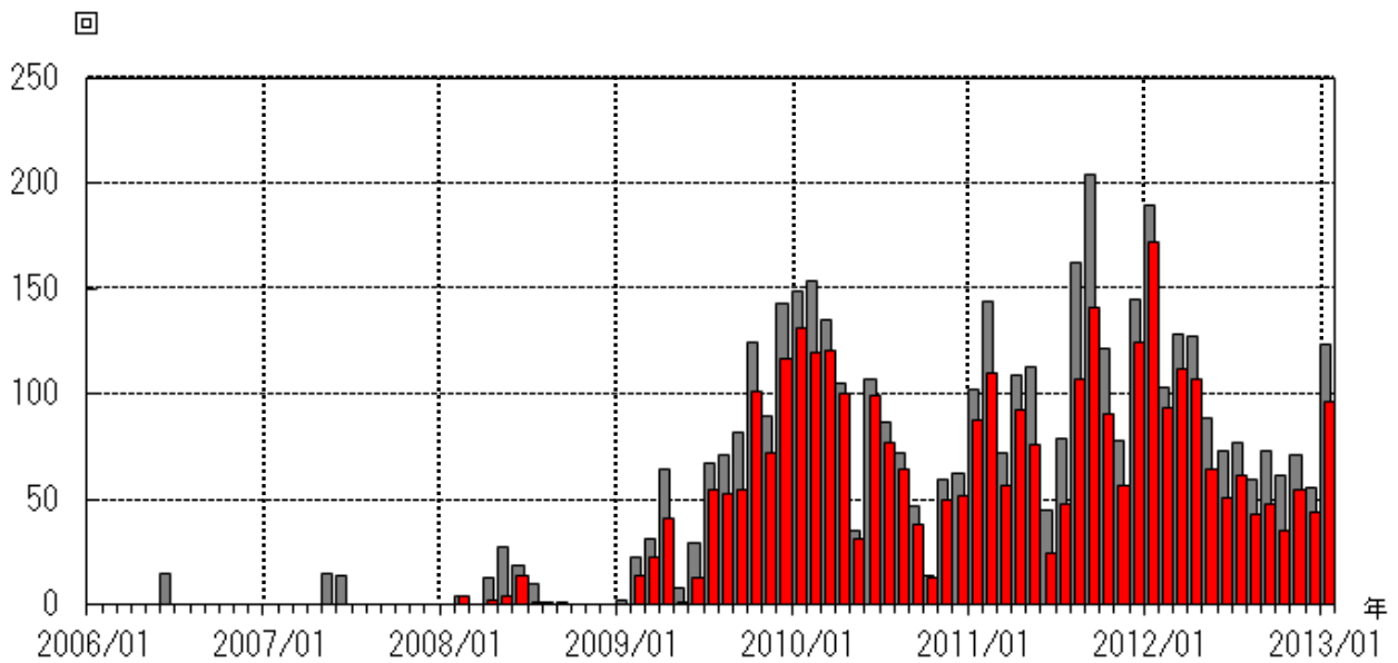
図2 桜島 昭和火口月別噴火回数（灰色）と昭和火口月別爆発回数（赤色） （2006年1月～2013年1月）
