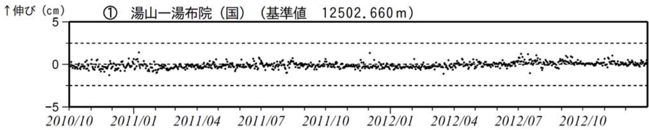
図 2※ 鶴見岳・伽藍岳 GPS連続観測による基線長変化（2010 年 10 月～2012 年 12 月）
