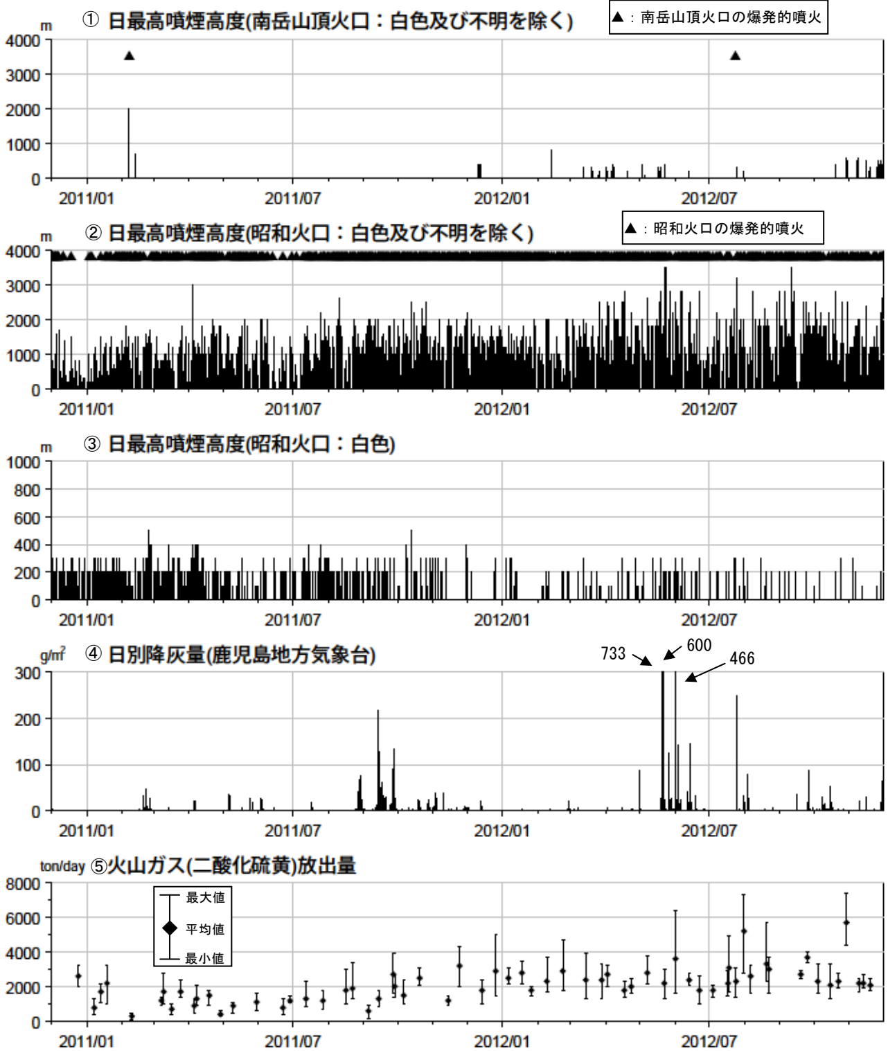
図 4 桜島 最近 2 年間の噴煙、降灰、火山ガス（2010 年 12 月～2012 年 11 月） <11 月の状況>
