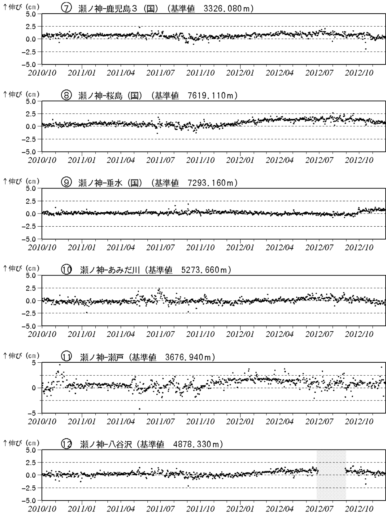
図 8-2* 桜島 GPS 連続観測による長期の基線長変化 (2010 年 10 月～2012 年 11 月)
