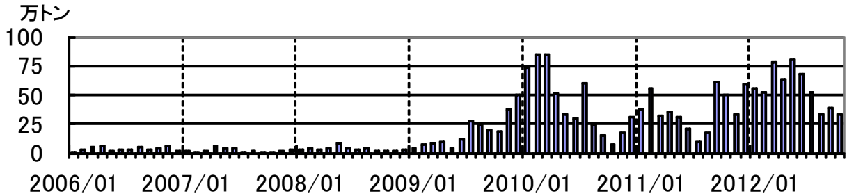
図 10※ 桜島 鹿児島県が実施している降灰の観測データから推定した火山灰の月別総噴出量（2006 年 1 月～2012 年 10 月）
