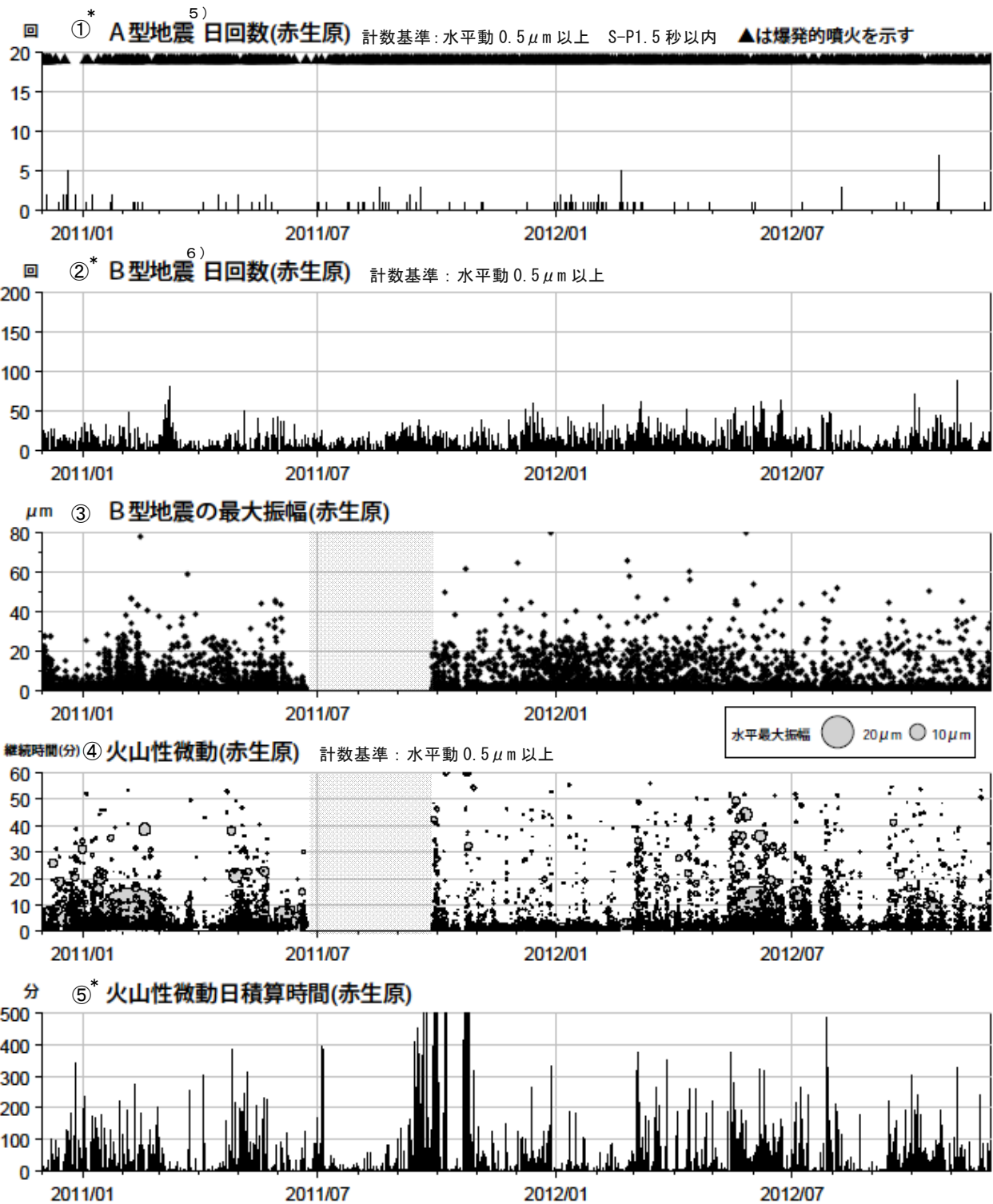
図5 桜島 最近2年間の火山性地震、火山性微動 (2010年12月～2012年11月)
