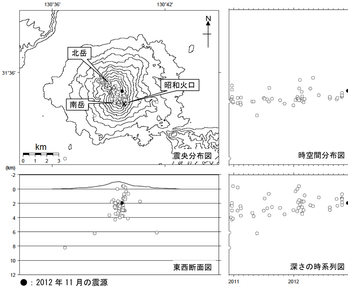
● : 2012 年 11 月の震源 ○ : 2010 年 12 月～2012 年 10 月の震源 図 6※ 桜島 震源分布図（2010 年 12 月～2012 年 11 月） <11 月の状況> 震源は、南岳直下の海拔下 2 km 付近でした。
