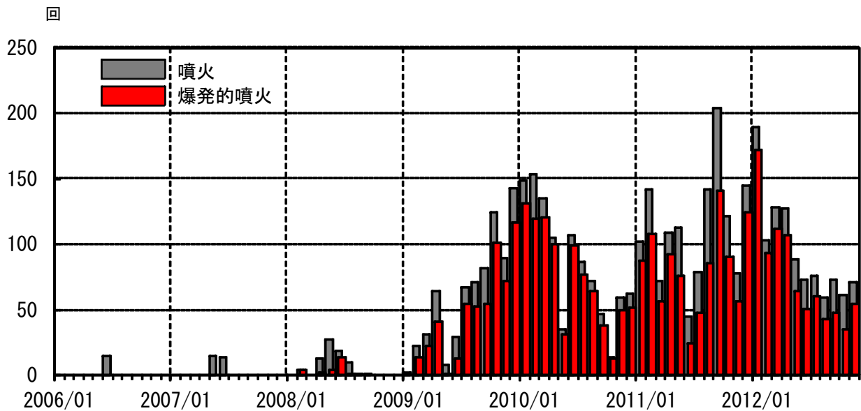
図3 桜島 昭和火口月別噴火回数（灰色）と昭和火口月別爆発回数（赤色） （2006年1月～2012年11月）
