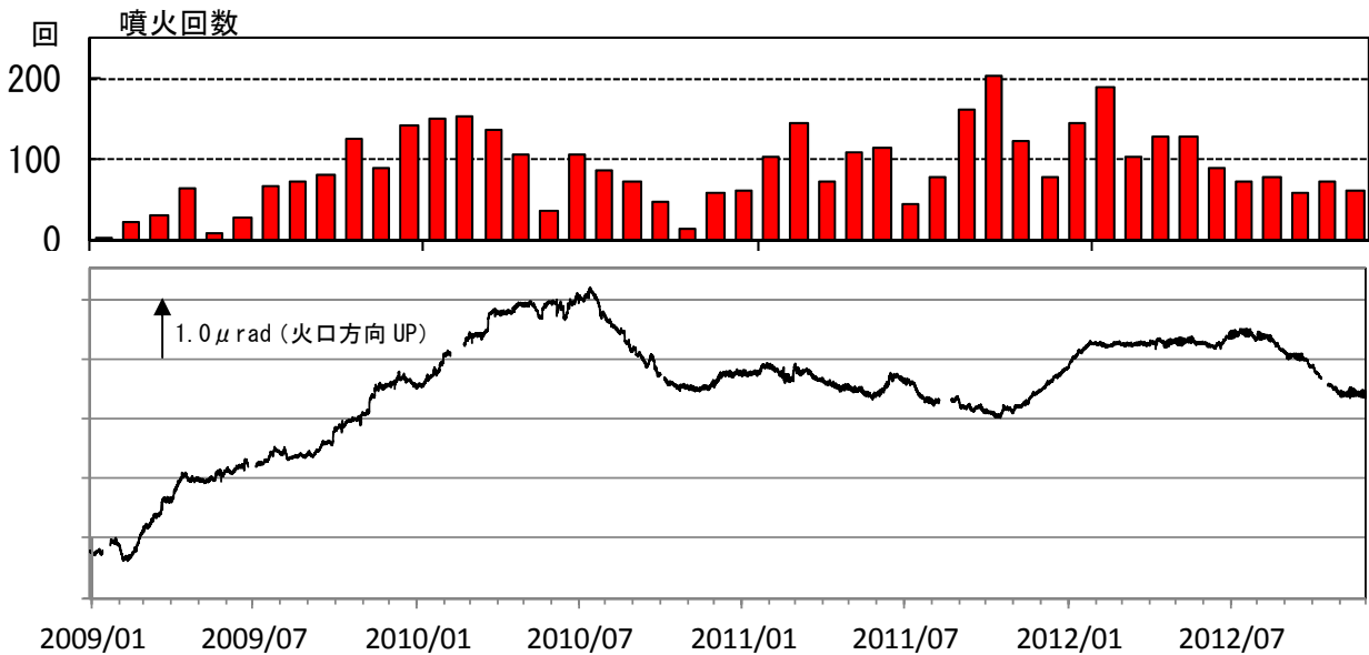
図 7※ 桜島 有村観測坑道の水管傾斜計（大隅河川国道事務所設置）の変化 （2009 年 1 月～2012 年 11 月）
