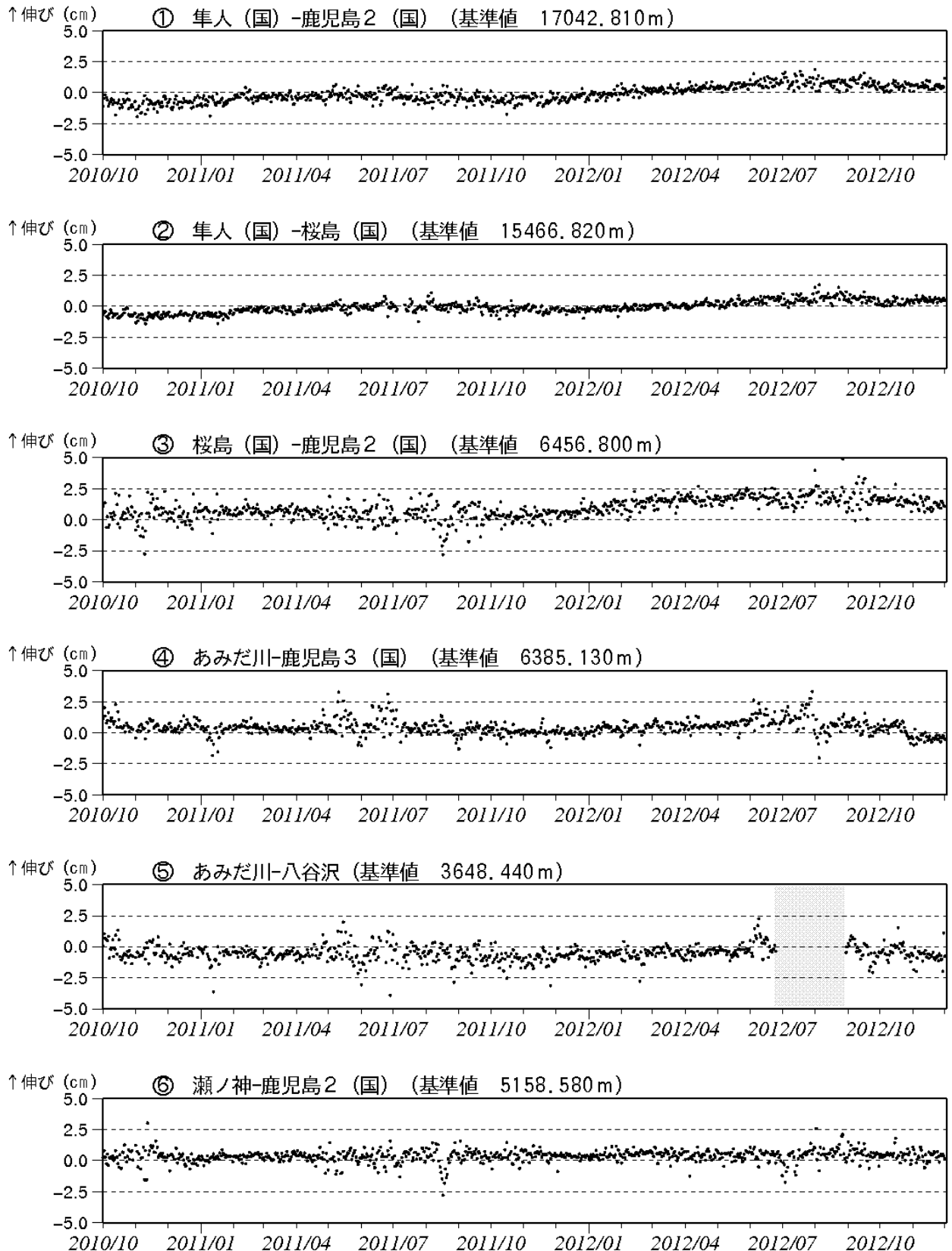
図 8-1※ 桜島 GPS 連続観測による長期の基線長変化 (2010 年 10 月～2012 年 11 月)
