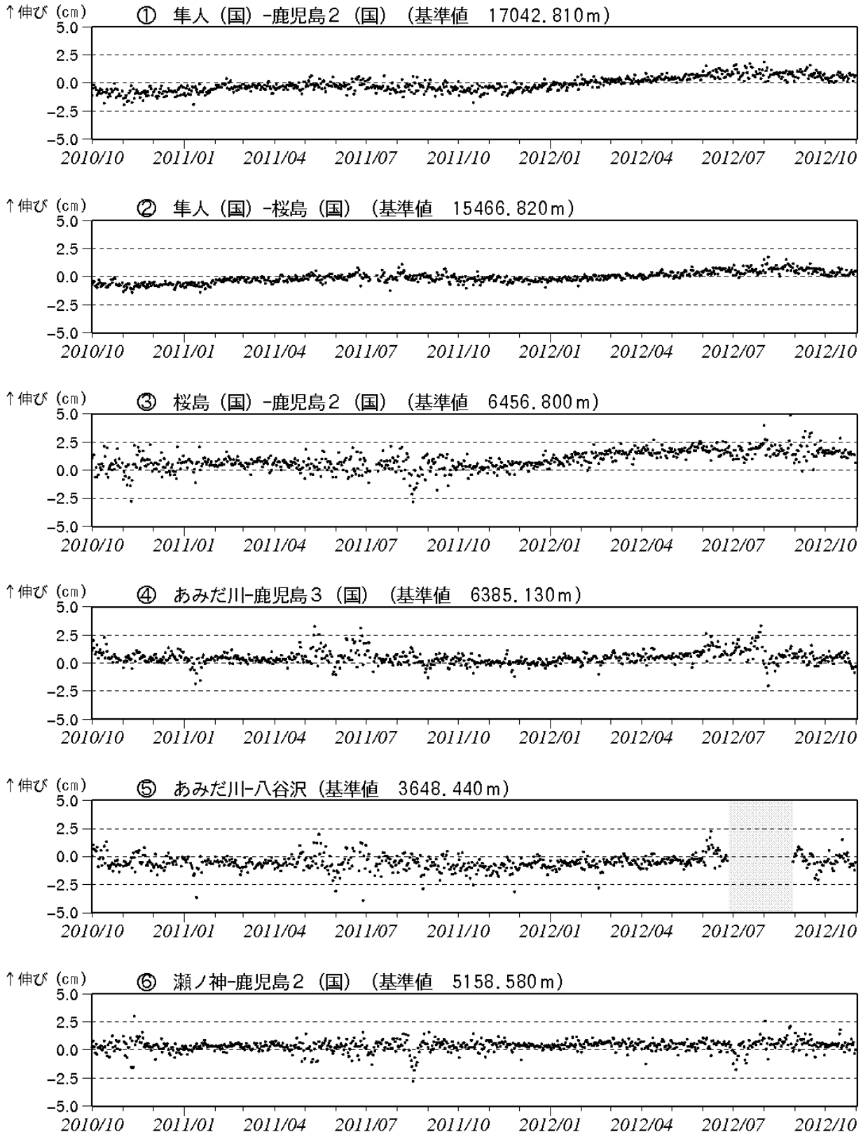
図 8-1※ 桜島 GPS 連続観測による長期の基線長変化（2010 年 10 月～2012 年 10 月）
