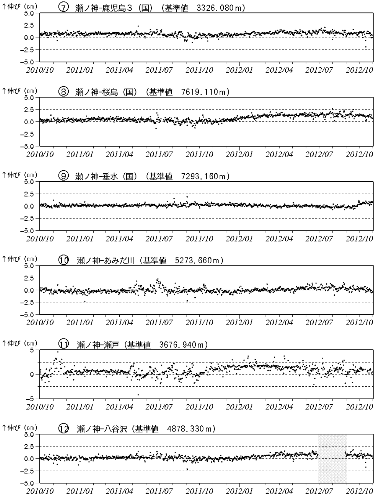
図 8-2* 桜島 GPS 連続観測による長期の基線長変化（2010 年 10 月～2012 年 10 月） 桜島島内及び始良カルデラ周辺の気象庁・国土地理院の 9 観測点の基線による観測を行っています。 この基線は図 9 の⑦～⑫に対応しています。 灰色の部分は機器障害のため欠測を示しています。
