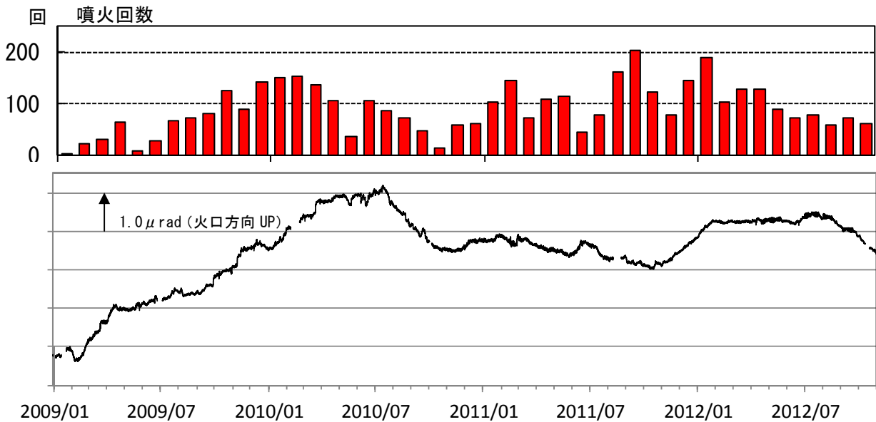
図 7※ 桜島 有村観測坑道の水管傾斜計（大隅河川国道事務所設置）の変化 （2009 年 1 月～2012 年 10 月） 2012 年 2 月頃から山体の変動は停滞していましたが、8 月頃からわずかに沈降しています。 ※有村観測坑道の傾斜変動は 0.48 \times 10^{-8} rad/day のトレンド補正を行っています。
