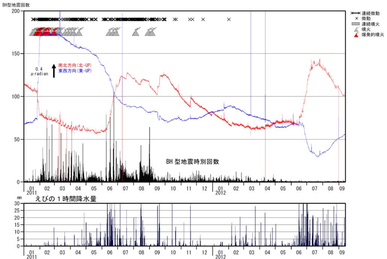
図3 霧島山（新燃岳） BH型地震 2) の時間別回数と高千穂河原傾斜計（新燃岳の南東約3km）の変化（2011年1月～2012年9月13日）
