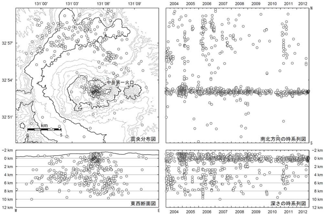
図 6※ 阿蘇山 震源分布図（2004 年 1 月～2012 年 9 月）
