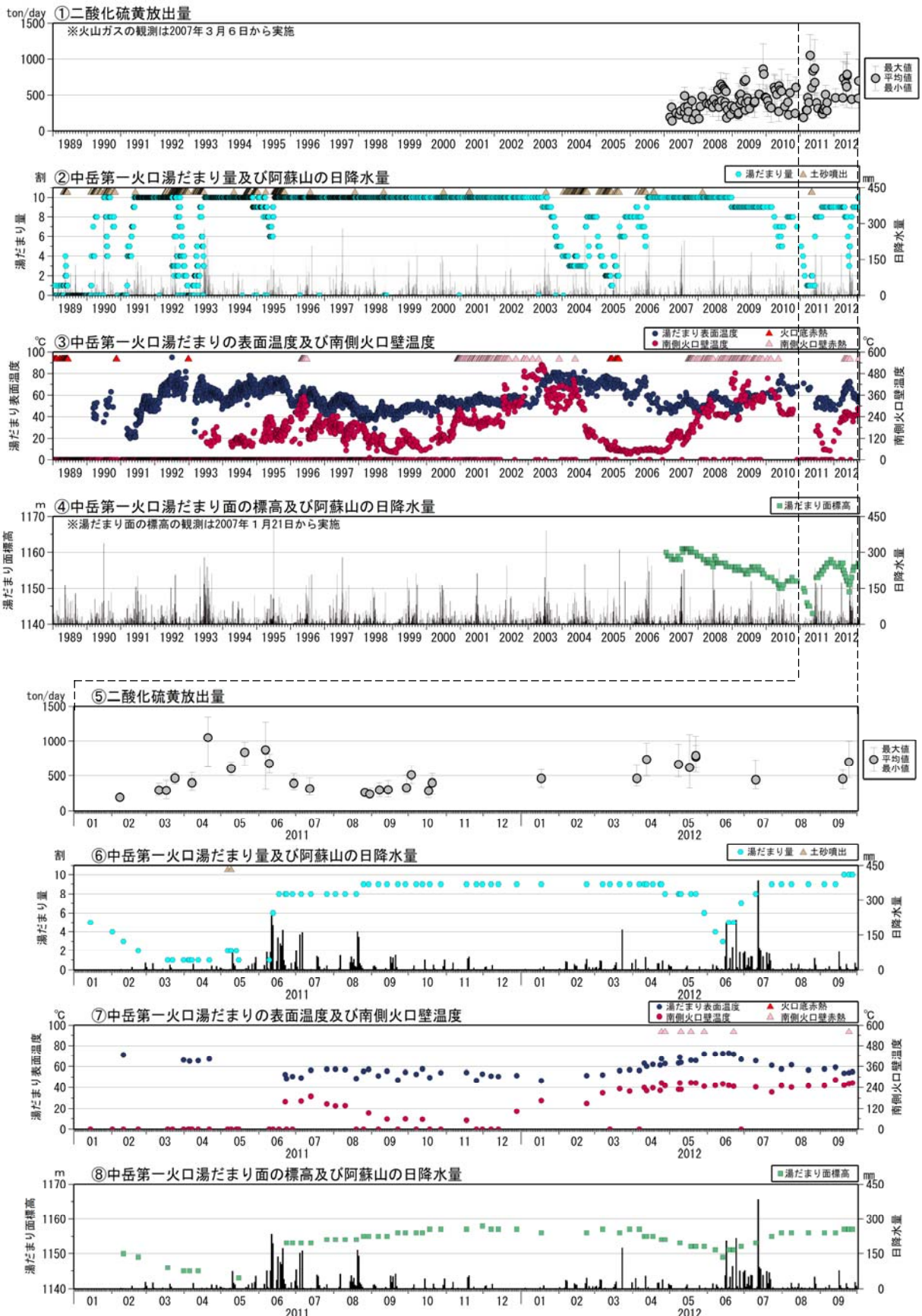
図5※ 阿蘇山 湯だまり、火口壁、二酸化硫黄放出量の状況（1989年1月～2012年9月） <9月の状況>
