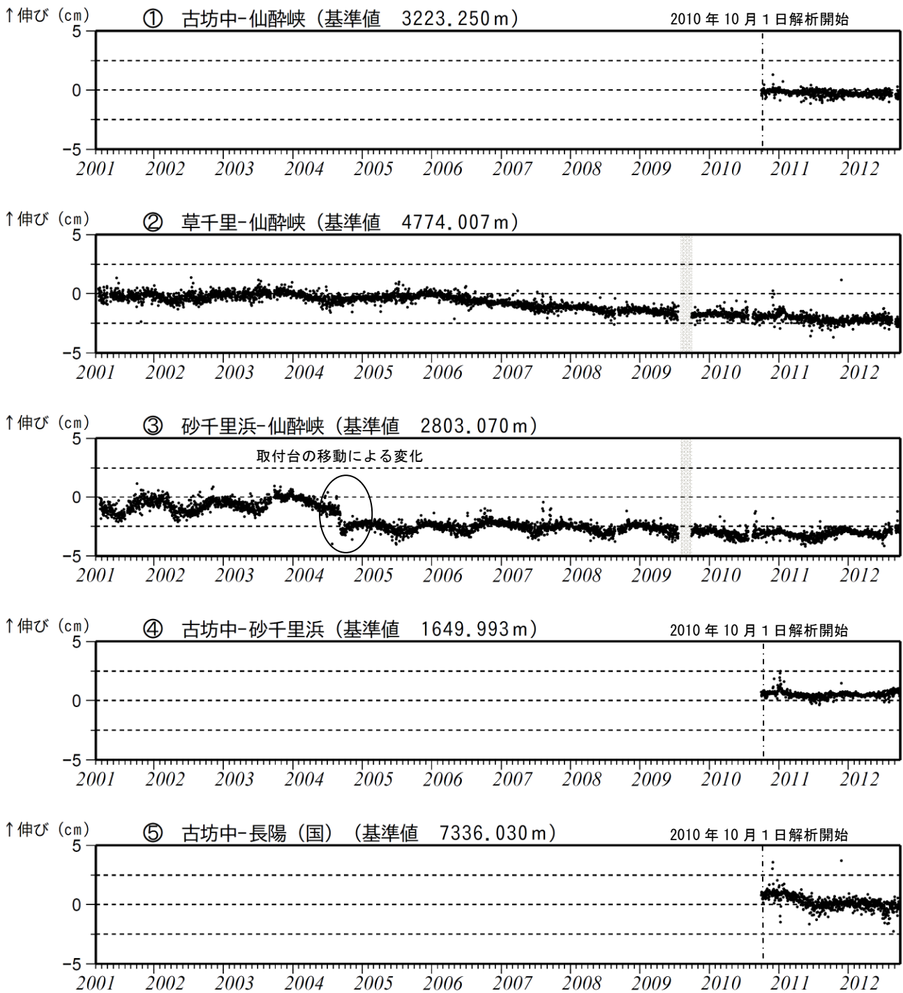
図 8※ 阿蘇山 GPS連続観測による基線長変化（2001 年 3 月～2012 年 9 月） GPS 連続観測では、火山活動によると考えられる変化は認められませんでした。
