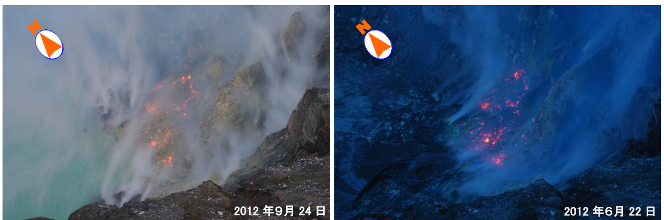
図 14 阿蘇山 中岳第一火口南西側から撮影した中岳第一火口南側火口壁の赤熱 （左：9月24日撮影 右：6月22日撮影） 赤熱現象の領域に特段の変化はありませんでした。
