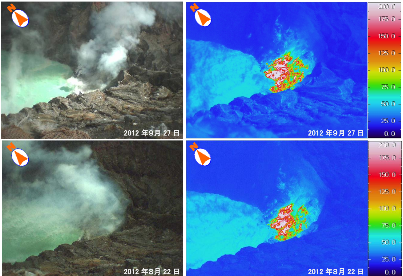
図 13 阿蘇山 赤外熱映像装置による中岳第一火口南側火口壁の地表面温度分布 （左：可視画像 右：赤外画像） （上段：9月27日撮影 下段：8月22日撮影） 温度分布に、特段の変化はありませんでした。
