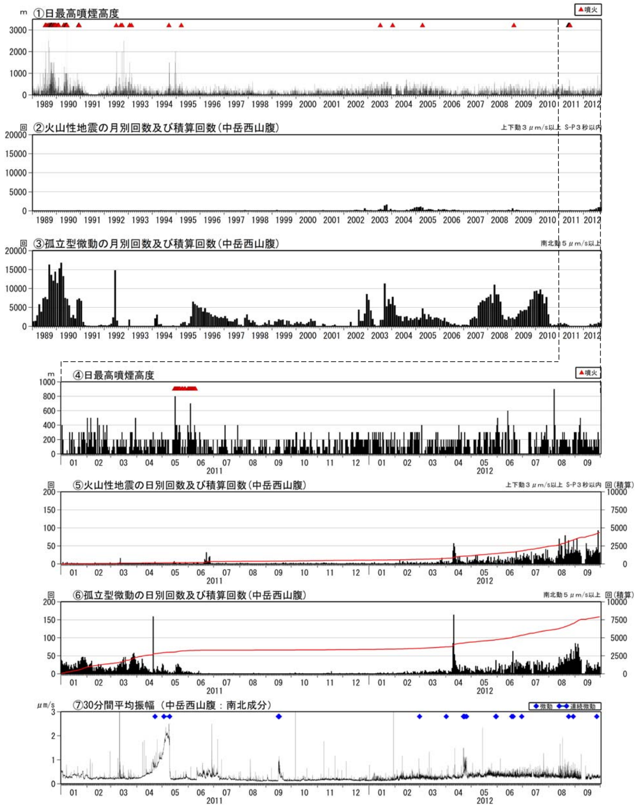
図 4 阿蘇山 火山活動経過図（1989 年 1 月～2012 年 9 月）
