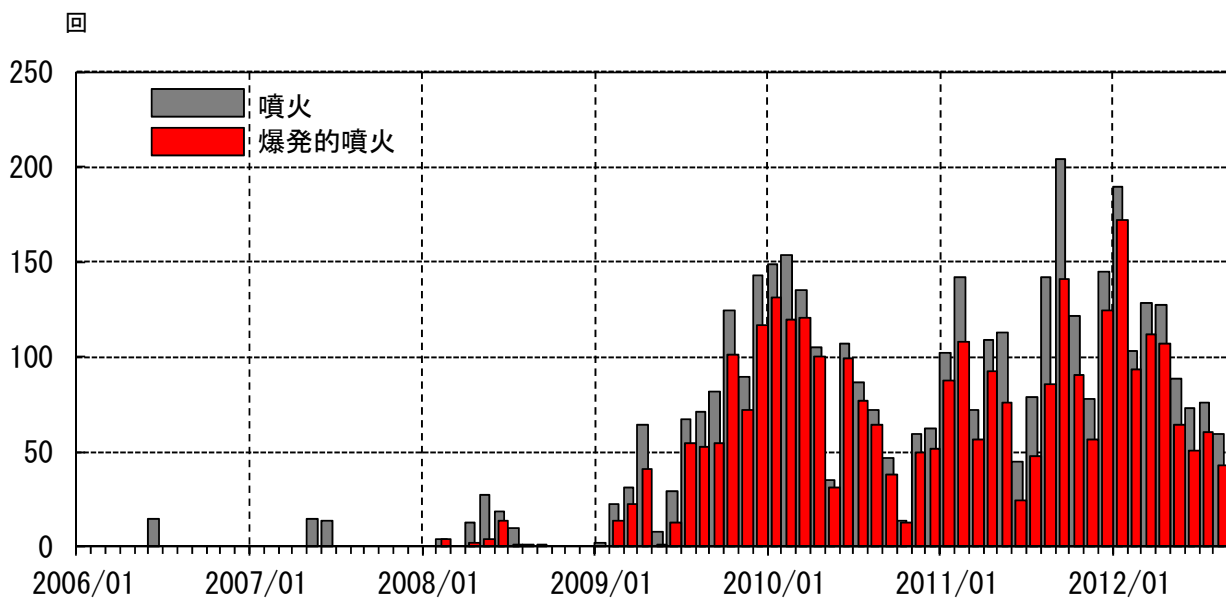
図3 桜島 昭和火口月別噴火回数（灰色）と昭和火口月別爆発回数（赤色） （2006年1月～2012年8月）
