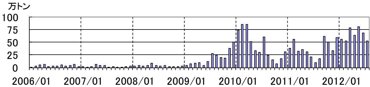
図 10※ 桜島 鹿児島県が実施している降灰の観測データから推定した火山灰の月別総噴出量（2006 年 1 月～2012 年 7 月）
