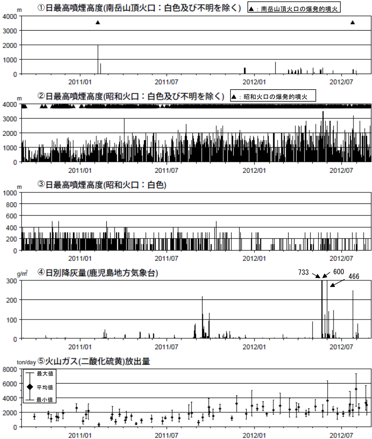
図4 桜島 最近2年間の噴煙、降灰、火山ガス（2010年9月～2012年8月）
