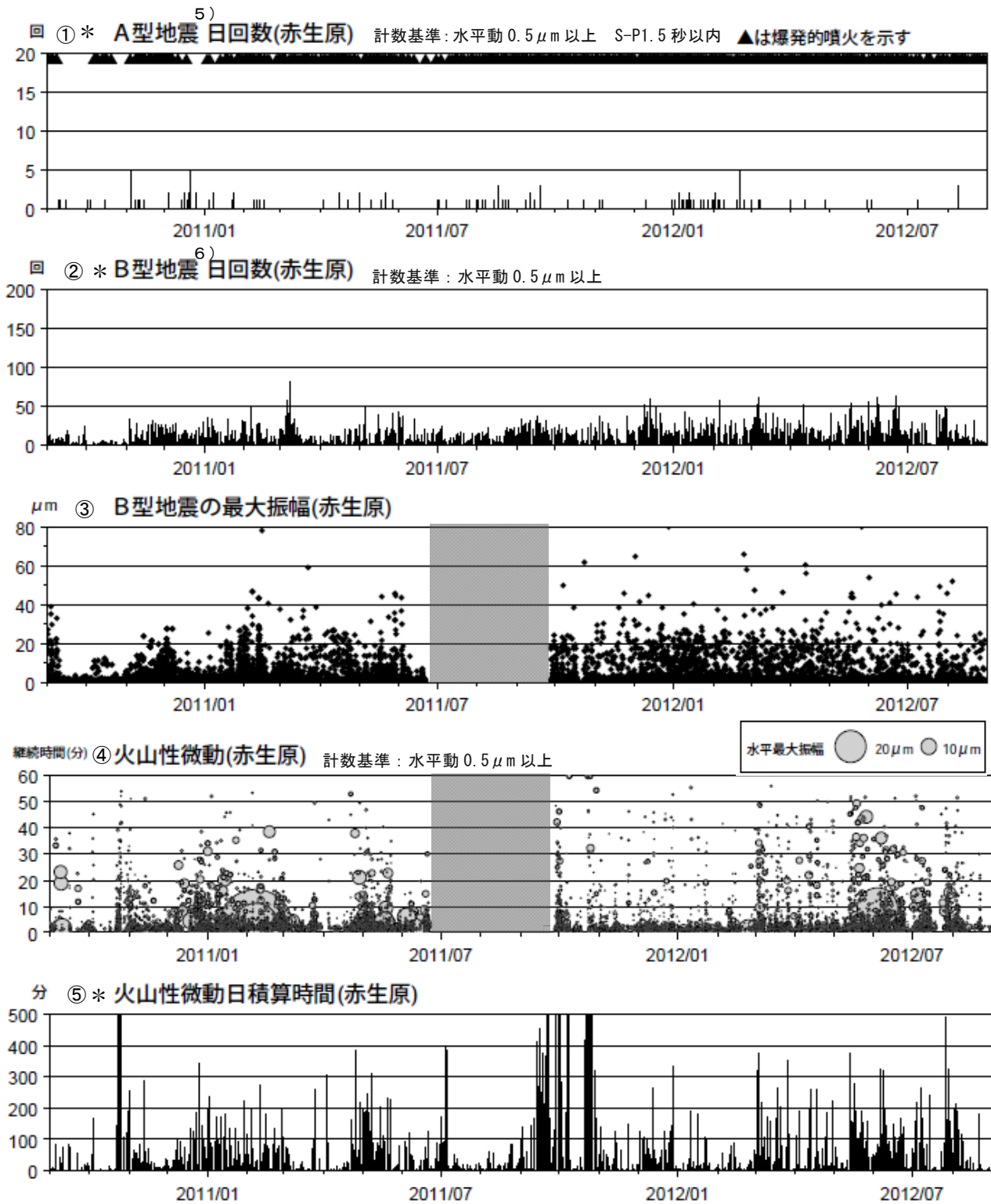
図5 桜島 最近2年間の火山性地震、火山性微動（2010年9月～2012年8月）
