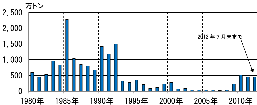
図 11※ 桜島 鹿児島県が実施している降灰の観測データから推定した火山灰の年別総噴出量（1980 年～2012 年）
