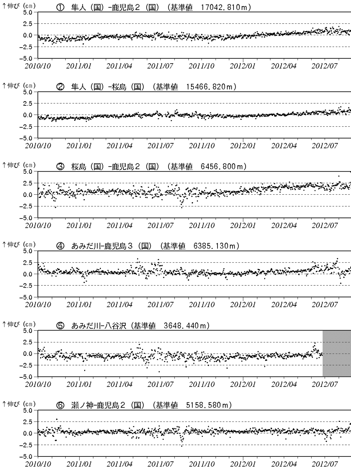
図 8-1※ 桜島 GPS 連続観測による長期の基線長変化（2010 年 10 月～2012 年 8 月）
