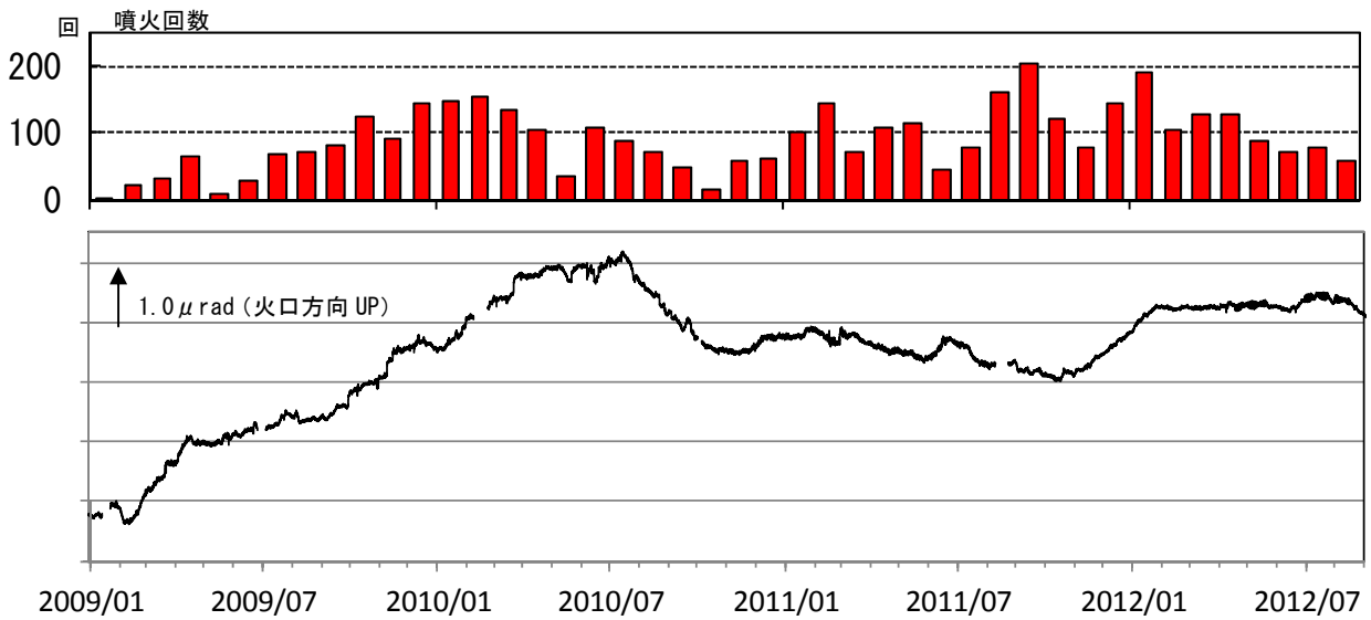
図 7 ※ 桜島 有村観測坑道の水管傾斜計 (大隅河川国道事務所設置) の変化 (2009 年 1 月～2012 年 8 月)
