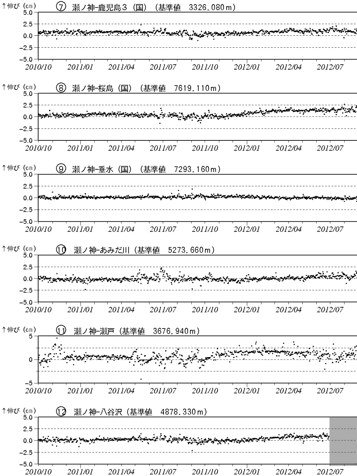
図 8-2※ 桜島 GPS 連続観測による長期の基線長変化（2010 年 10 月～2012 年 8 月） 桜島島内及び始良カルデラ周辺の気象庁・国土地理院の 9 観測点の基線による観測を行っています。 この基線は図 11 の⑦～⑫に対応しています。 灰色の部分は機器障害のため欠測を示しています。
