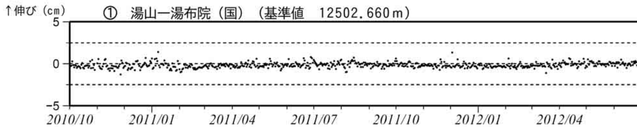
図 2* 鶴見岳・伽藍岳 GPS連続観測による基線長変化（2010年10月～2012年6月30日） < 6月の状況 > 火山活動によると考えられる変化は認められませんでした。 この基線は図3の①に対応しています。
