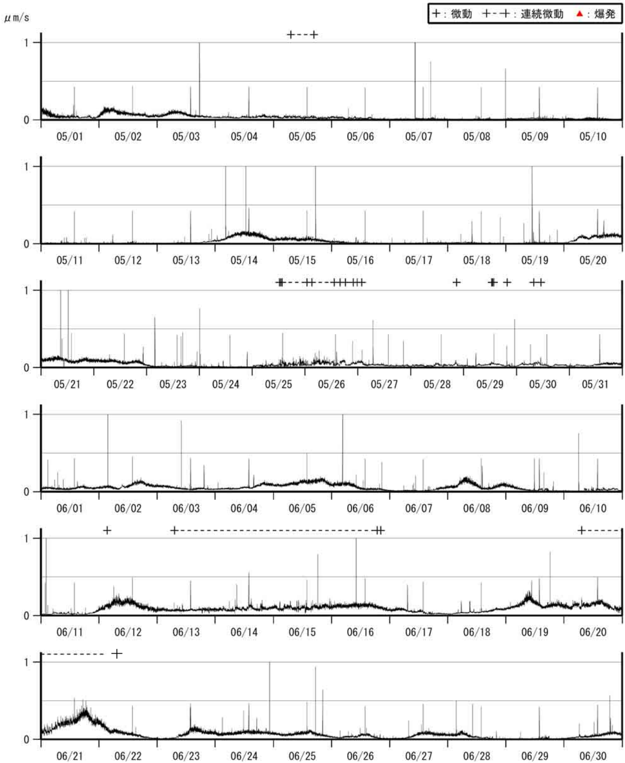
図 4 諏訪之瀬島 1 分間平均振幅の時間変化（ナベタオ上下成分）（2012 年 5 月～ 6 月） < 6 月の状況 > 火山性微動の継続時間の月合計は 132 時間 24 分（5 月：40 時間 11 分）と増加しました。
