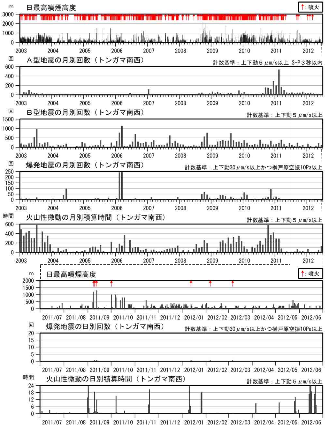
図3 諏訪之瀬島 火山活動経過図（2003年1月～2012年6月）
