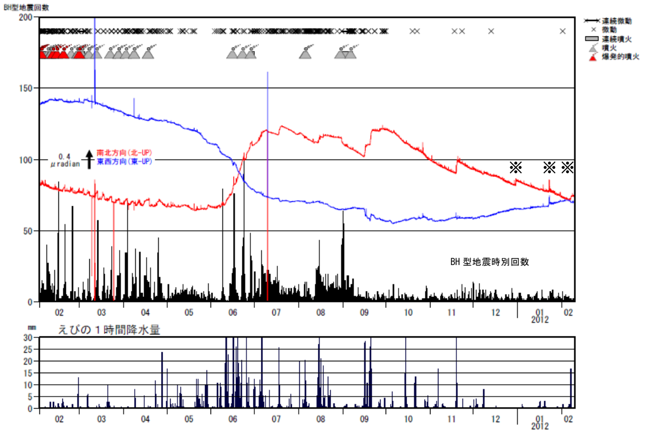
図3 霧島山（新燃岳） BH型地震 2) の時間別回数と高千穂河原傾斜計（新燃岳の南東約3km）の変化（2011年2月～2012年2月9日）
