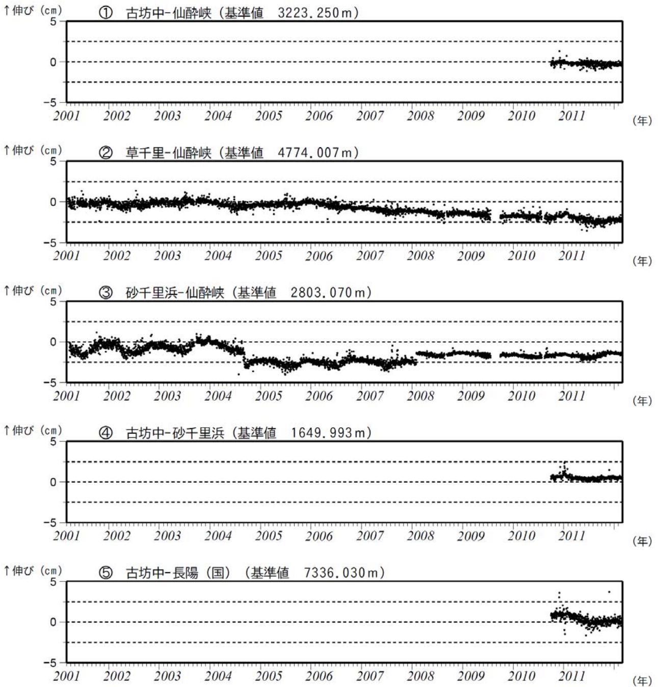
図6※ 阿蘇山 GPS連続観測による基線長変化（2001年3月～2012年2月）
