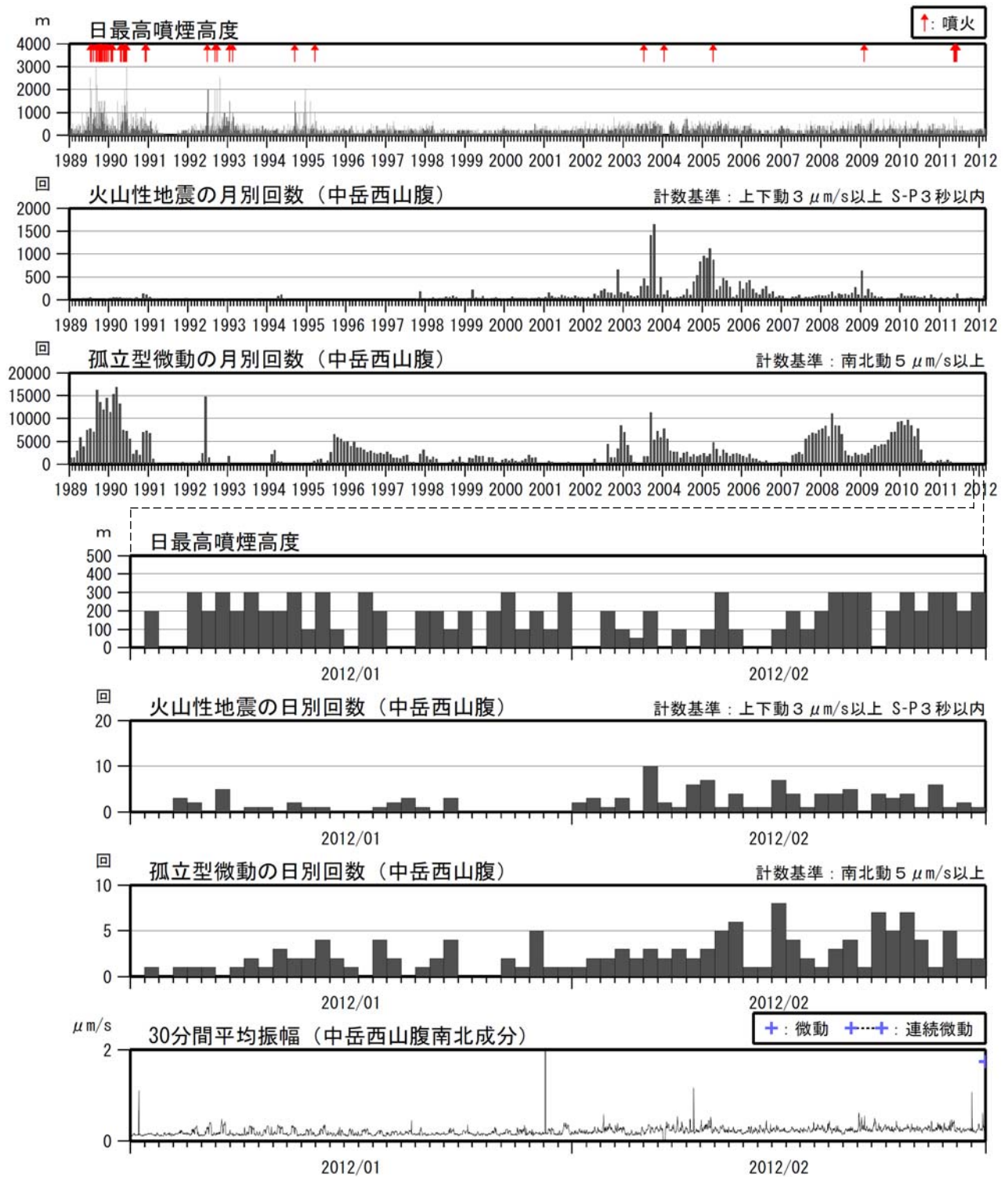
図 2 阿蘇山 噴煙、火山性地震、孤立型微動の状況（1989 年 1 月～2012 年 2 月）
