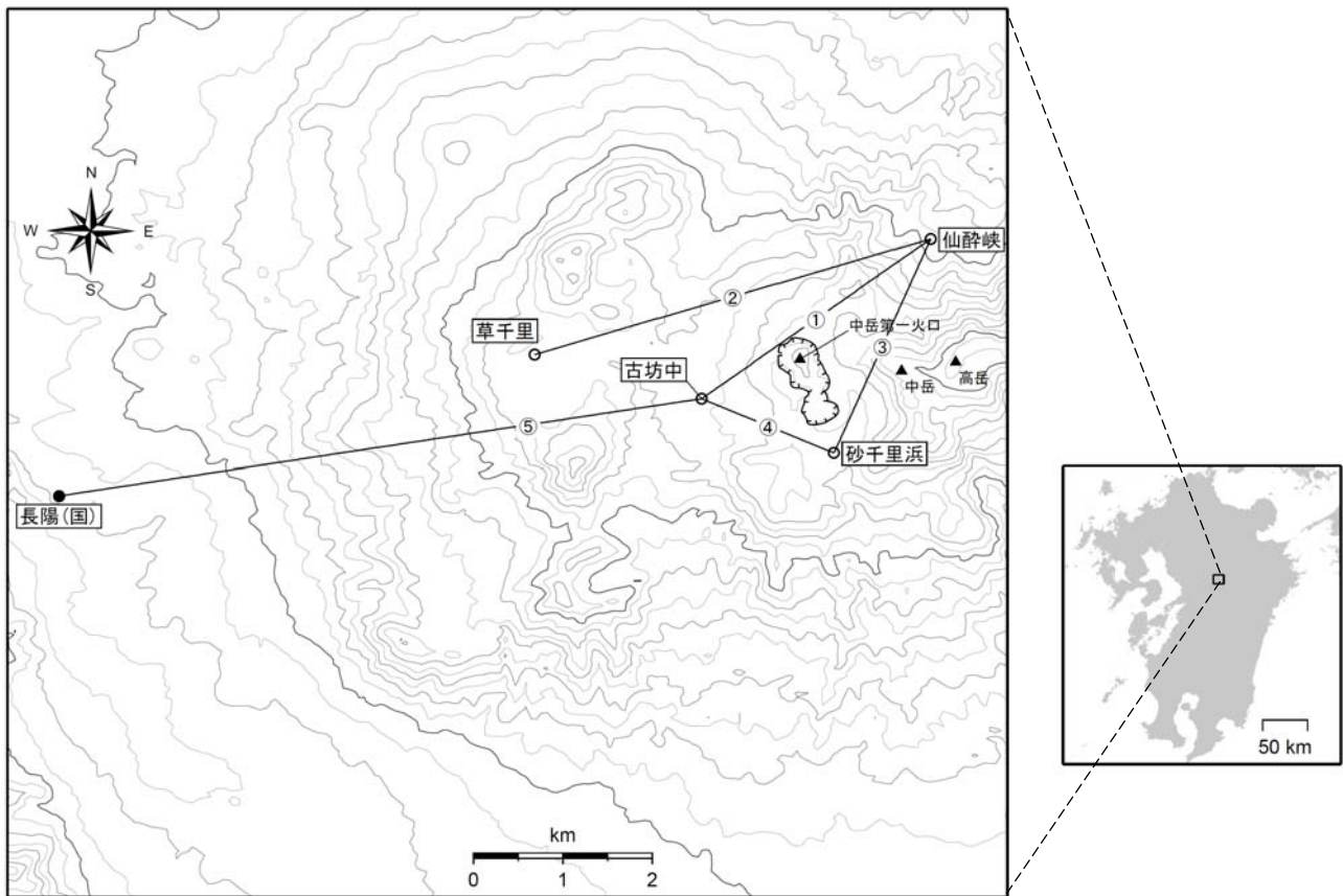
図 5 阿蘇山 GPS 連続観測点と基線番号
