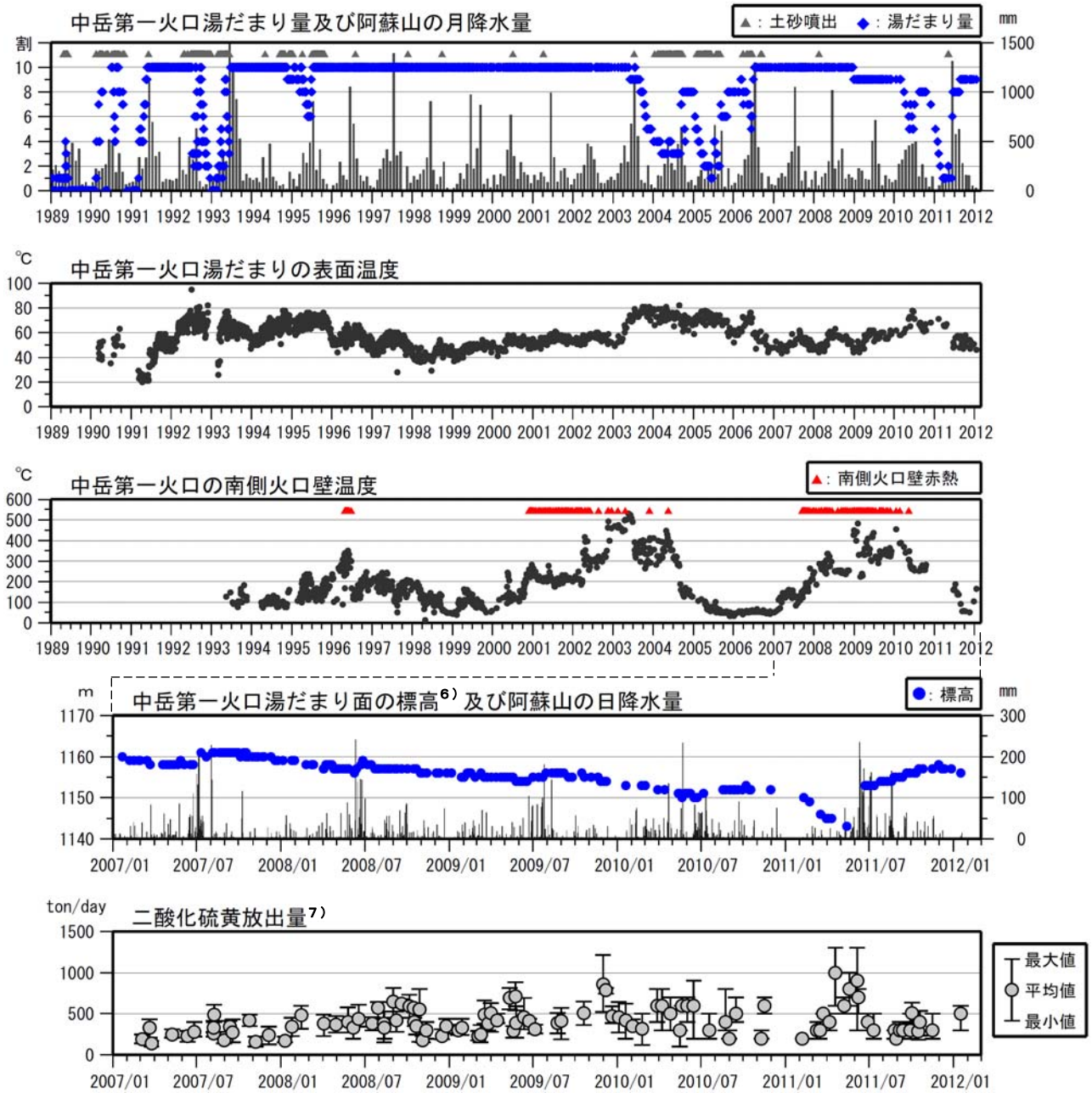
図 3※ 阿蘇山 湯だまり、火口壁、二氧化硫黄放出量の状況（1989 年 1 月～2012 年 2 月） < 2 月の状況 >
