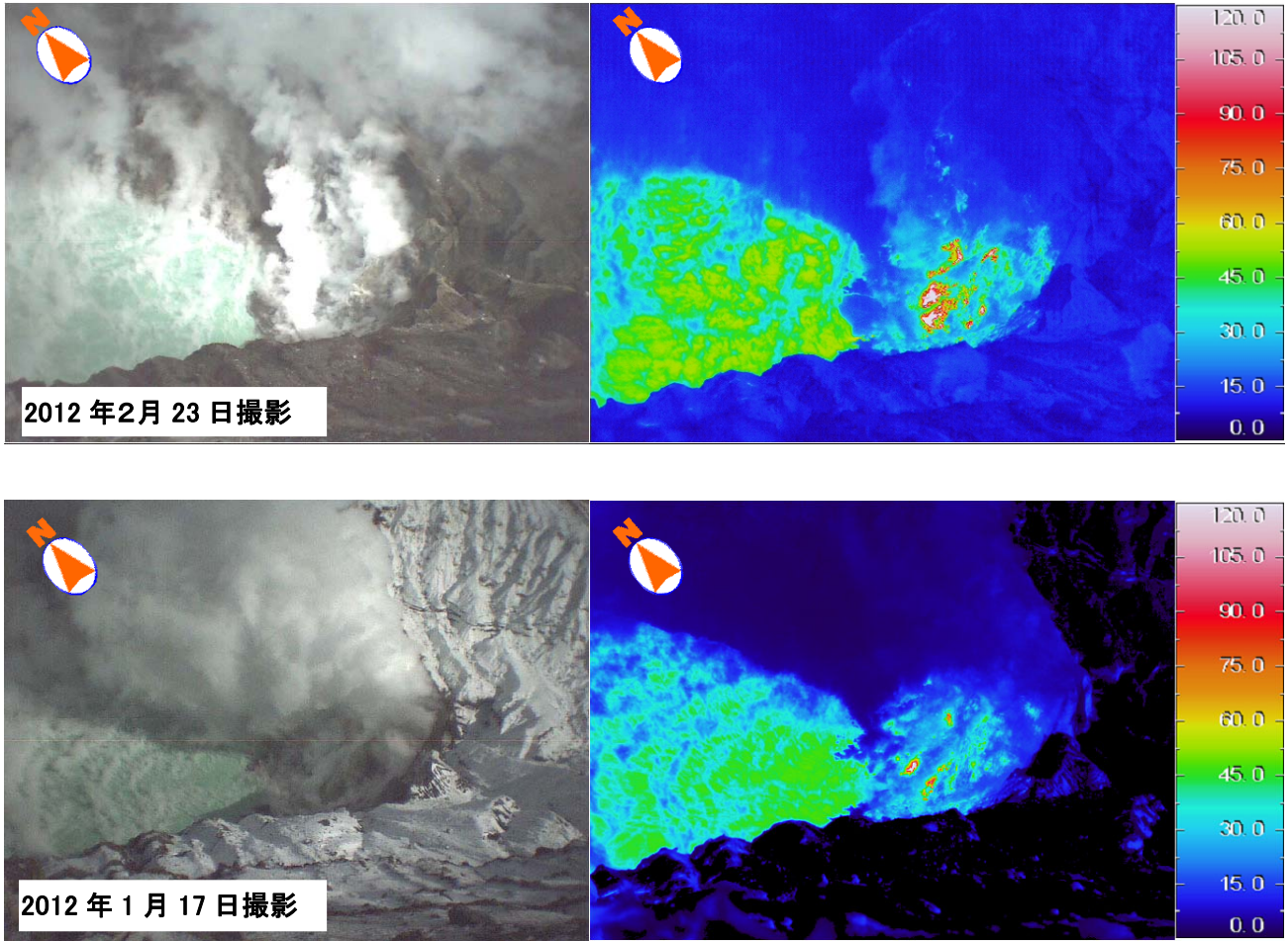
図9 阿蘇山 赤外熱映像装置による中岳第一火口南側火口壁の地表面温度分布 温度分布に特段の変化はありませんでした。
