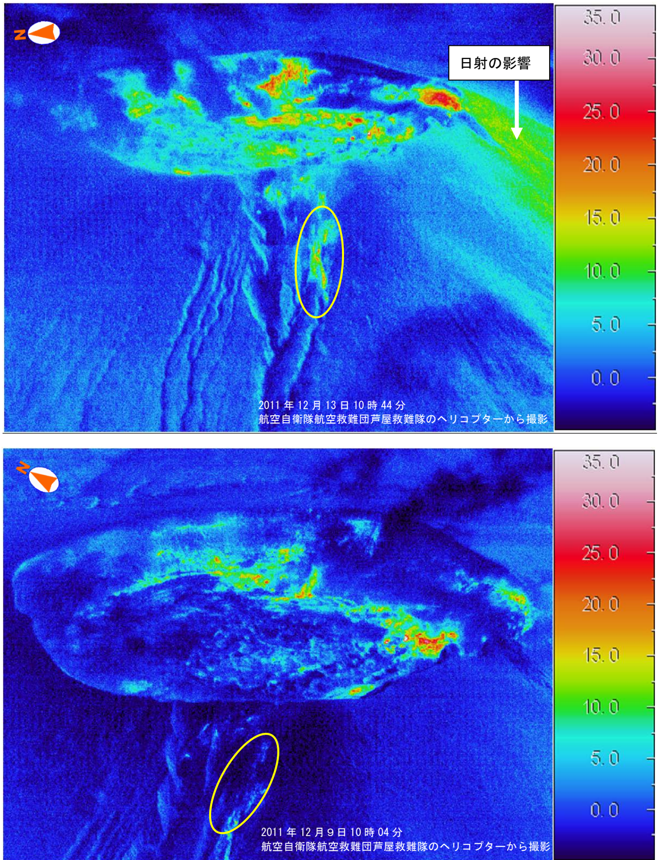
図2 霧島山（新燃岳） 赤外熱映像装置による火口付近の地表面温度分布 前回（9日）と比較して地表面温度分布に大きな変化はなく、火口内に蓄積された溶岩の縁辺部が比較的高温でした。また、西側斜面の割れ目の一部では、噴気は観測されませんでした。前回の調査と同様にやや温度の高い部分が認められました。
