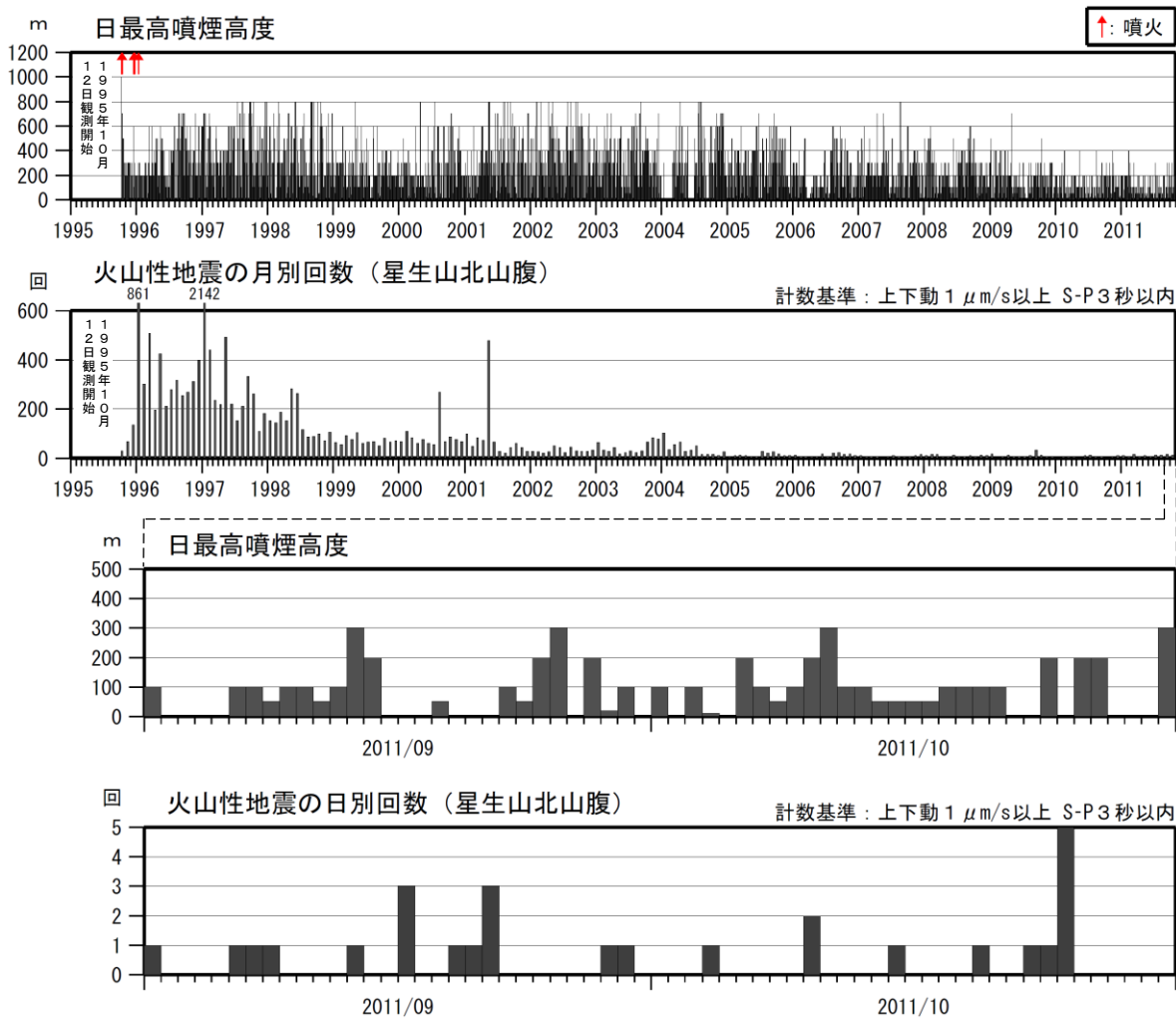
図 2 九重山 火山活動経過図（1995年10月～2011年10月）
