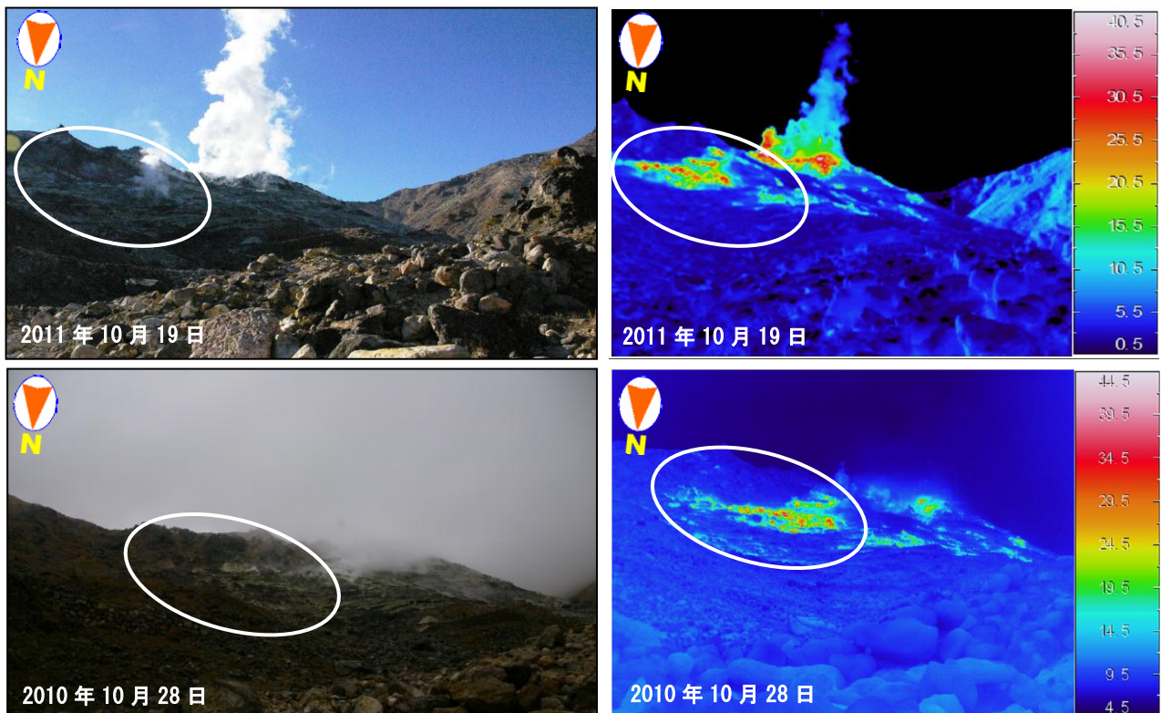
図 9 九重山 赤外熱映像装置による A 領域（白丸）の地表面温度分布（A 領域定点から撮影） 前回（2010 年 10 月 28 日）の観測と比べて熱異常域の分布に特段の変化は認められませんでした。
