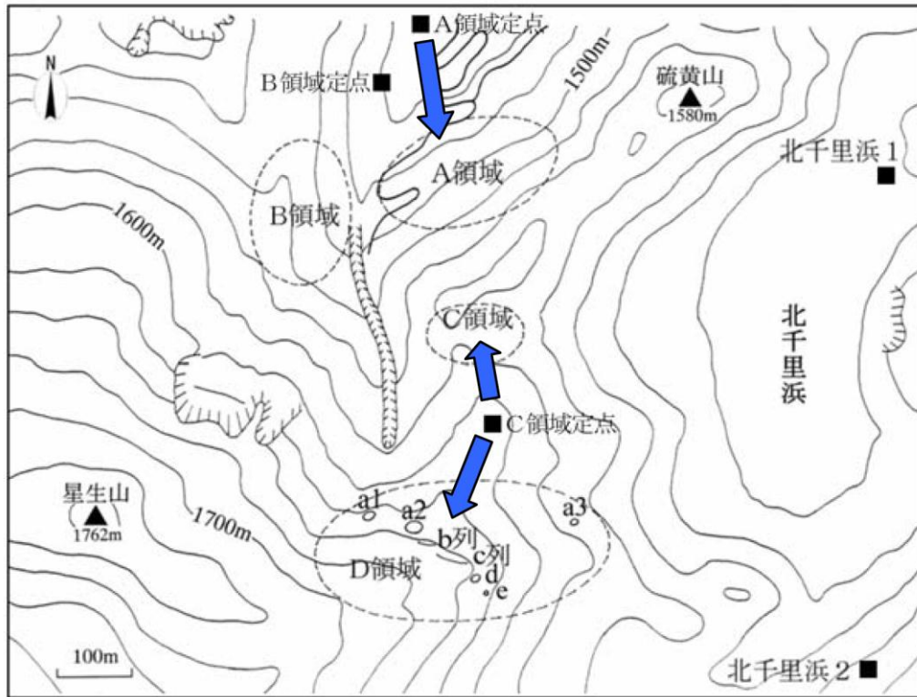
図 8 九重山 目視・熱観測点配置図
