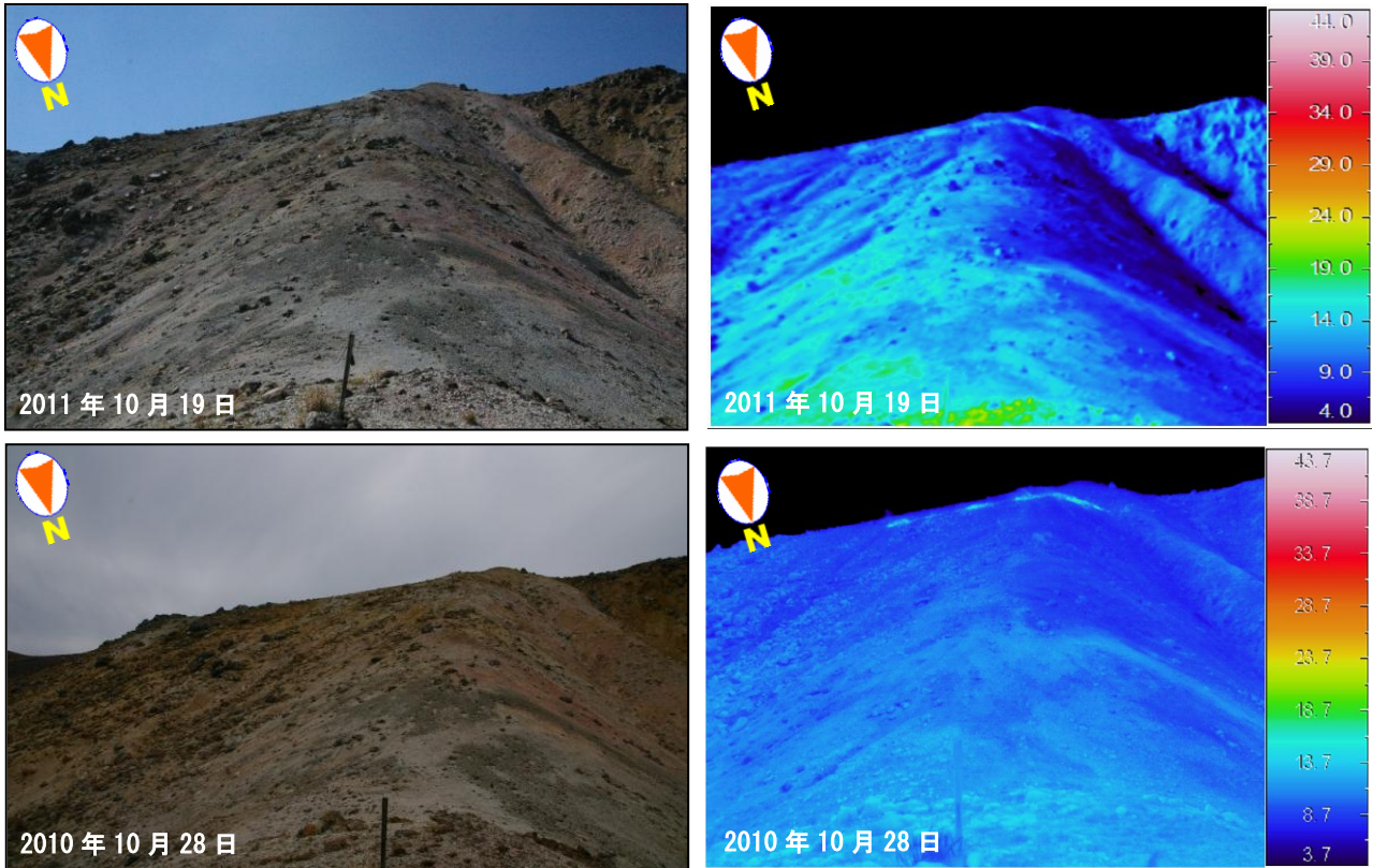
図 10 九重山 赤外熱映像装置によるD領域b火孔列の地表面温度分布（C領域定点から撮影） 前回（2010年10月28日）の観測と比べて熱異常域の分布に特段の変化は認められませんでした。
