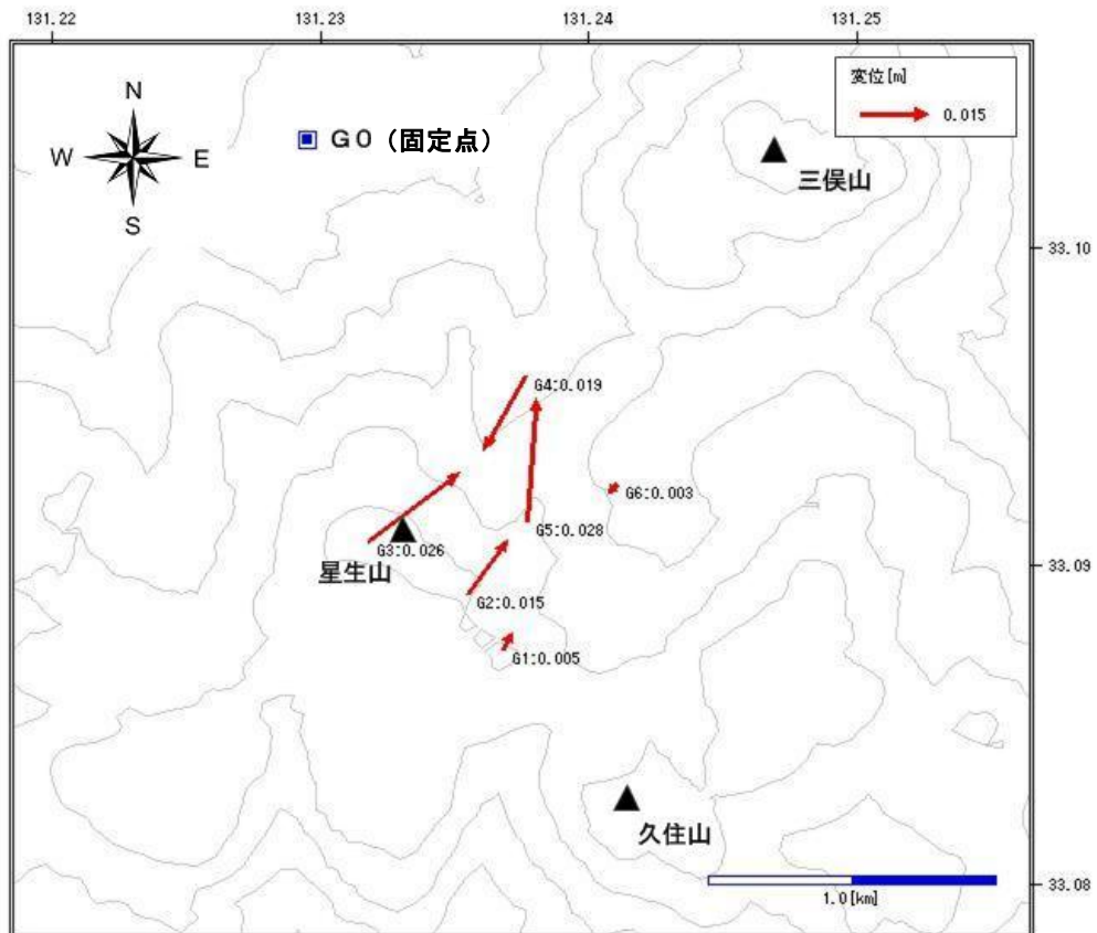
図6 九重山 GPS 繰り返し観測による変位ベクトル（2010年10月～2011年10月） 火山活動によると考えられる変化は認められませんでした。山体の収縮傾向が引き続き観測されました。
