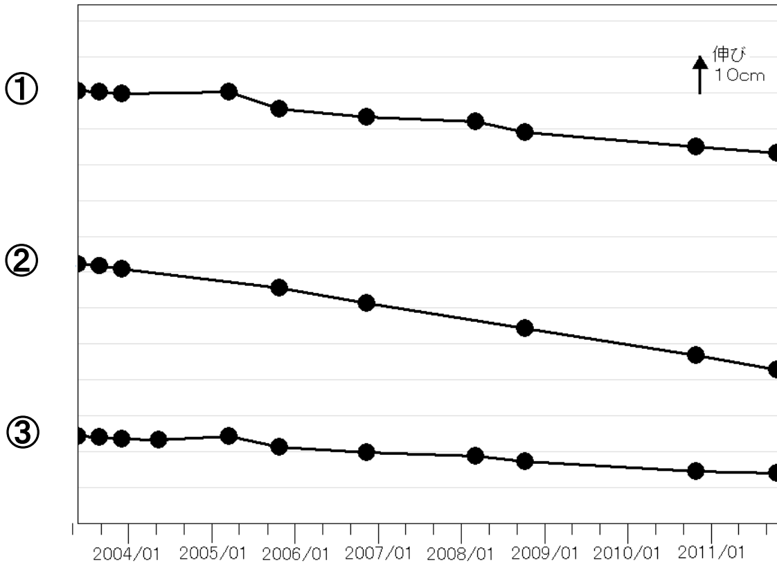
図7 九重山 GPS 繰り返し観測による基線長変化（2003年5月～2011年10月） 火山活動によると考えられる変化は認められませんでした。山体の収縮傾向が引き続き観測されました。
