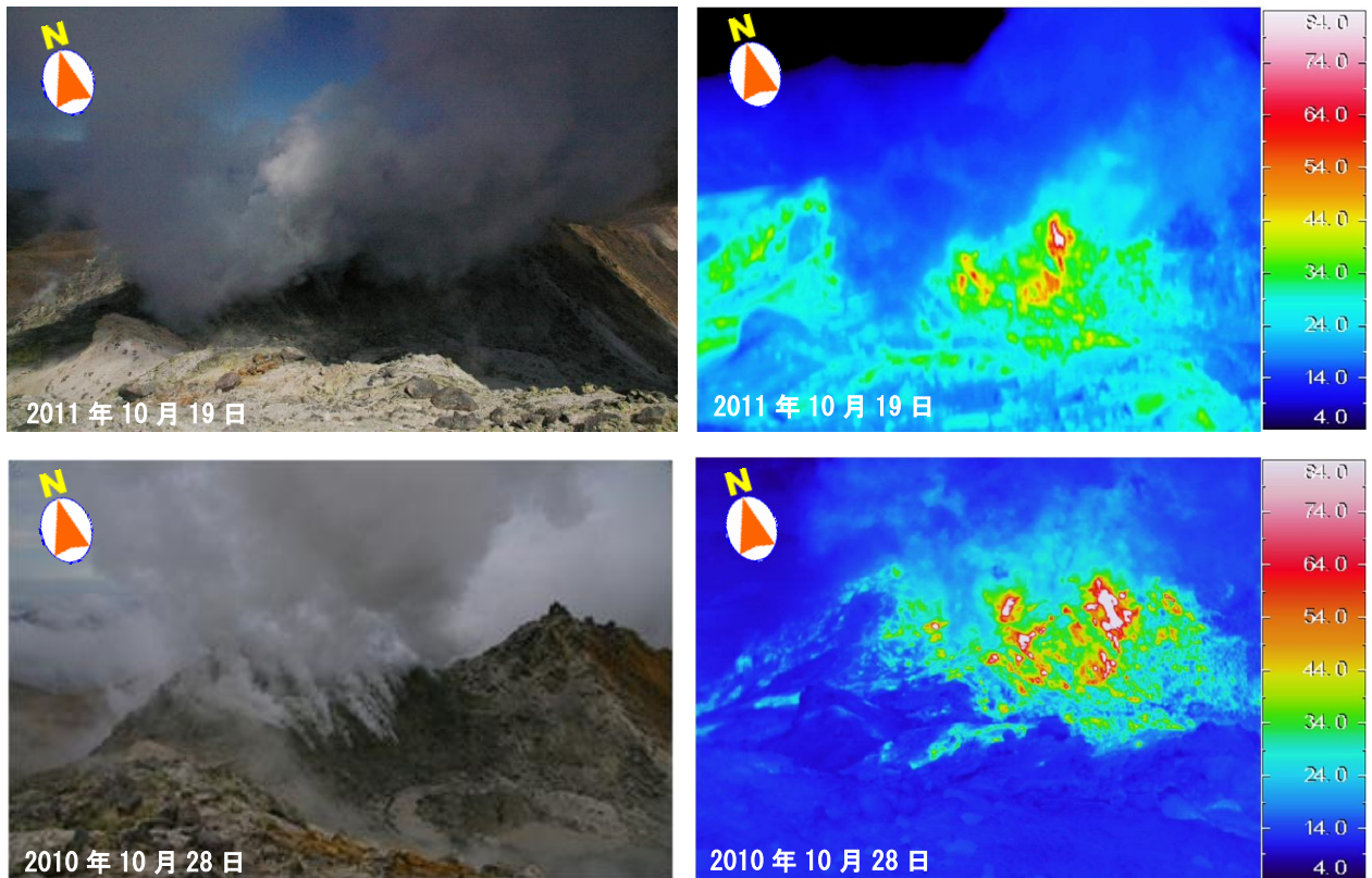
図 11 九重山 赤外熱映像装置によるC領域の地表面温度分布（C領域定点から撮影） 前回（2010年10月28日）の観測と比べて熱異常域の分布に特段の変化は認められませんでした。
