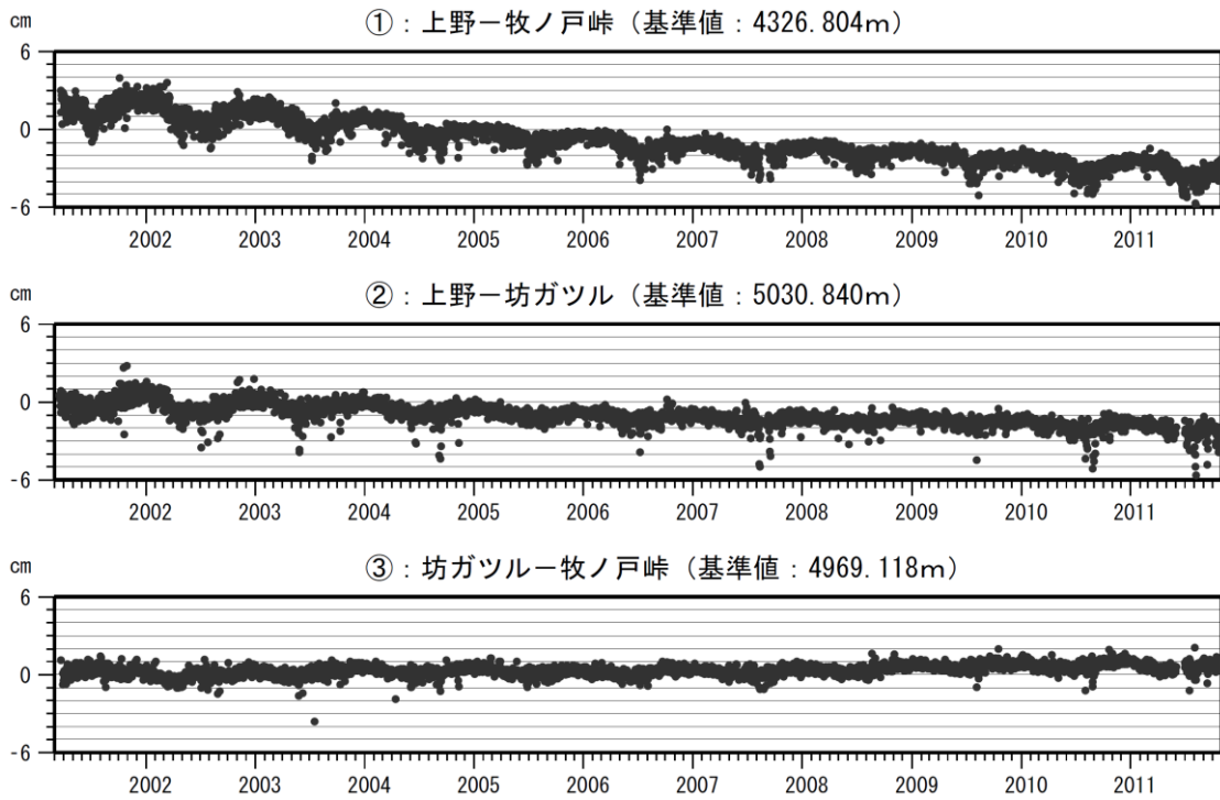
図 3 九重山 GPS 連続観測による基線長変化（2001 年 3 月～2011 年 10 月） ①、②の基線に長期的な縮みの傾向がみられていましたが、2008 年以降鈍化しています。 この基線は図 4 の①～③に対応しています。
