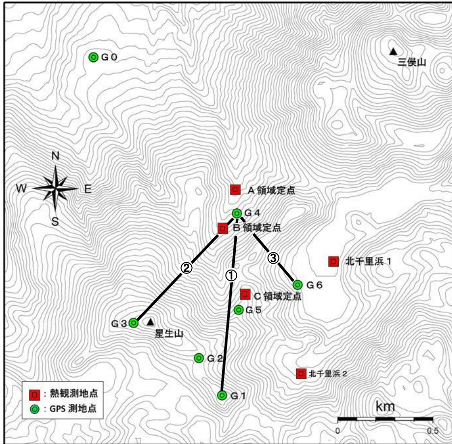
図5 九重山 GPS 繰り返し観測、目視・熱観測 観測点配置図
