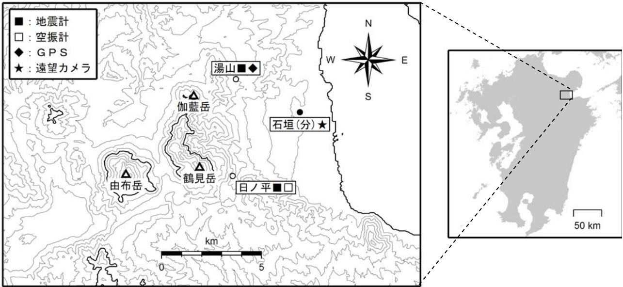
図 2 鶴見岳・伽藍岳 観測点配置図
