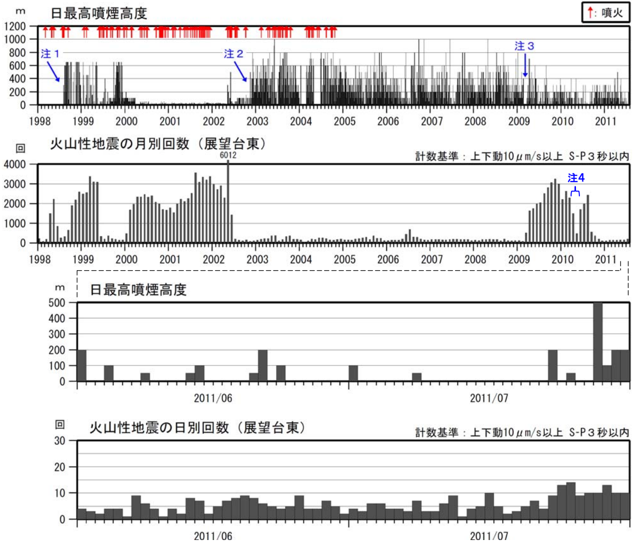
図2 薩摩硫黄島 火山活動経過図（1998年1月～2011年7月）
