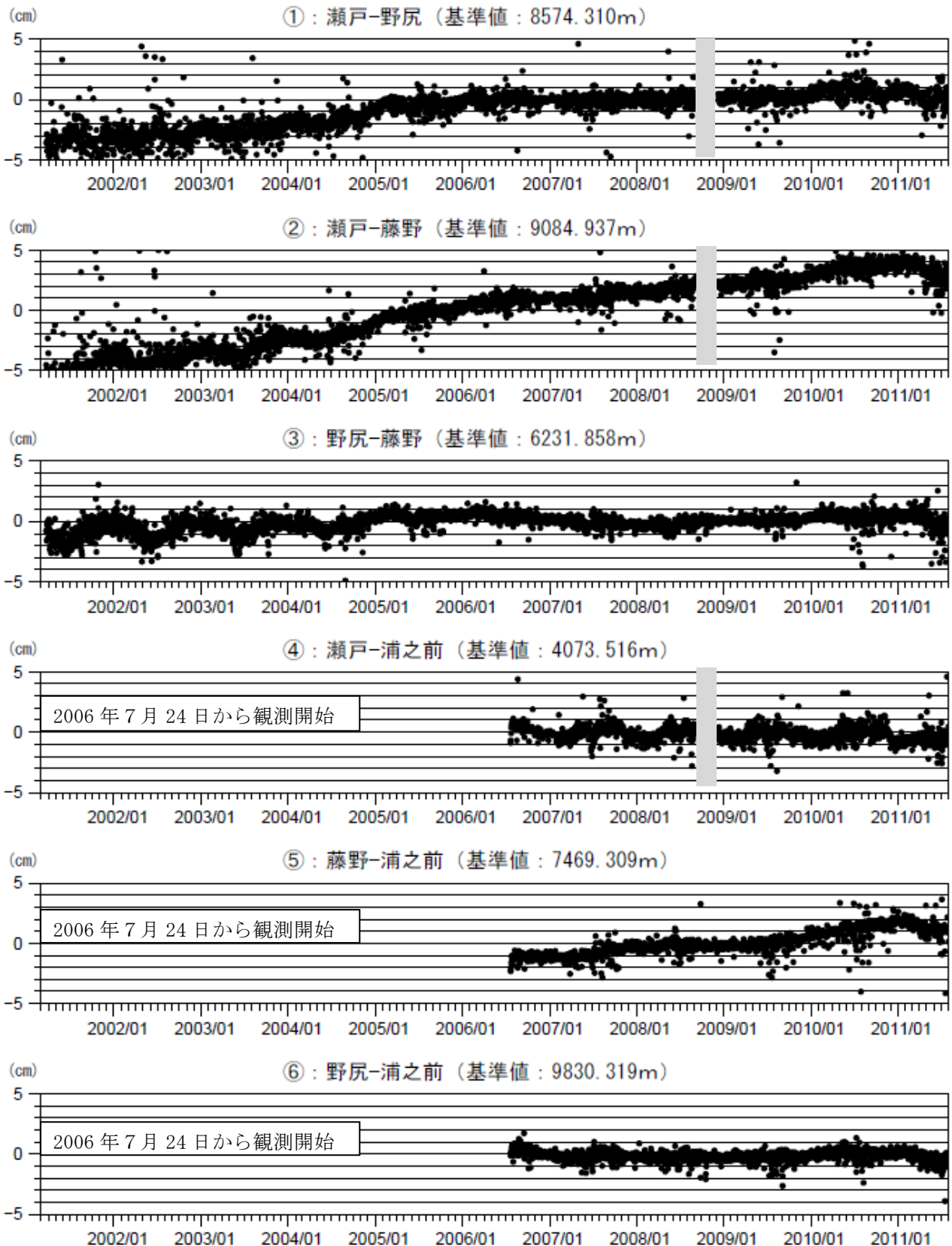
図9 桜島 GPS 連続観測による長期の基線長変化（2001年3月～2011年7月）
