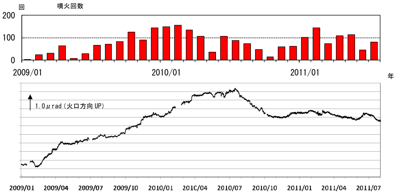
図 8※ 桜島 有村観測坑道の水管傾斜計 (大隅河川国道事務所設置) の変化 (2009 年 1 月～2011 年 7 月)
