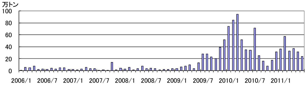
図 12※ 桜島 鹿児島県が実施している降灰量観測による月別降灰量
