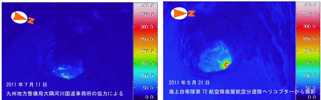
図 15 桜島 赤外熱映像装置による昭和火口内の表面温度分布 （左：2011 年 7 月 11 日、右：2011 年 5 月 31 日） ・今回確認した溶岩に対応した部分に高温の領域が認められました。 ・前回（5 月 31 日）と比べて特段の変化はありません。
