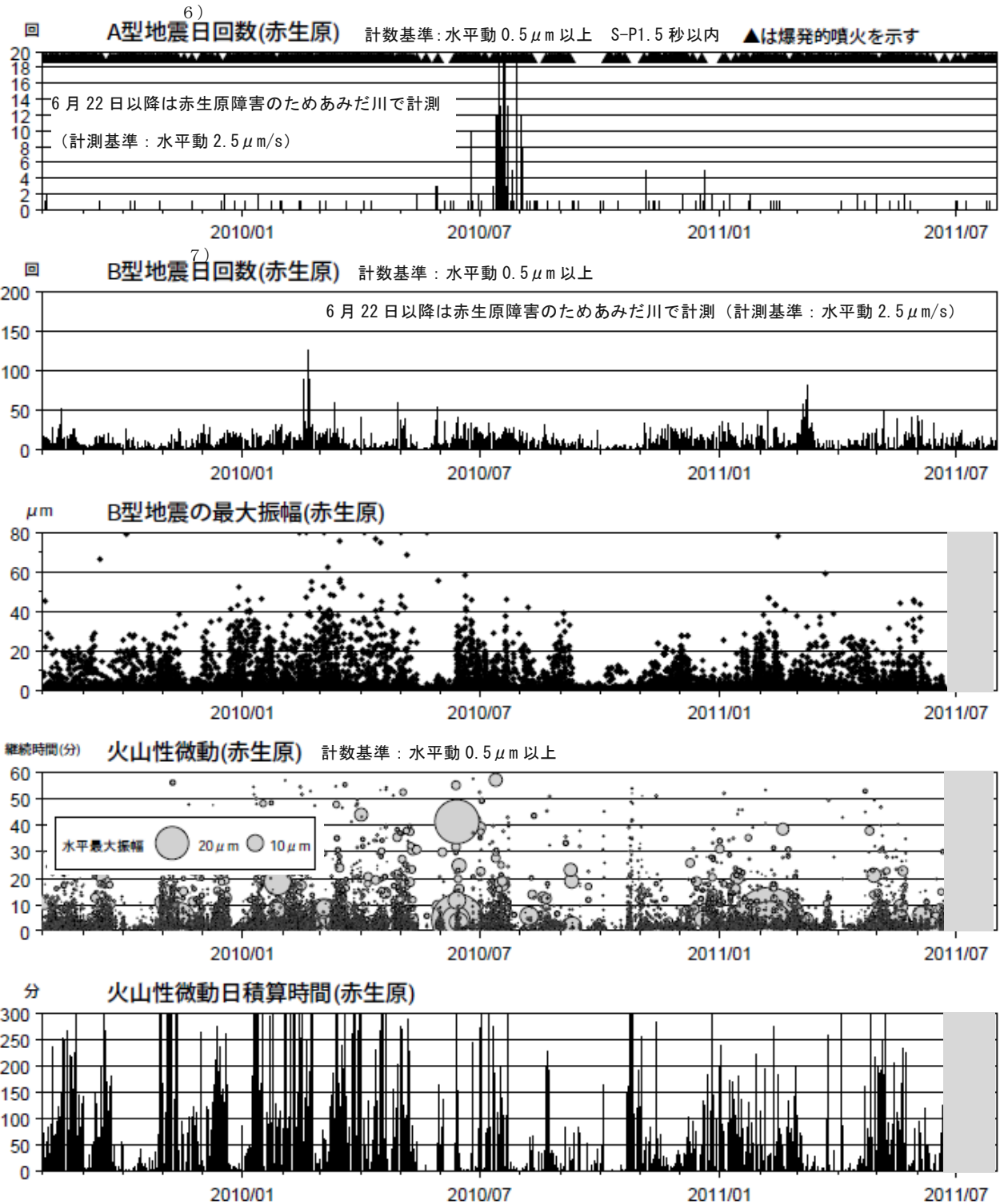
図6 桜島 最近2年間の火山性地震、火山性微動（2009年8月～2011年7月）
