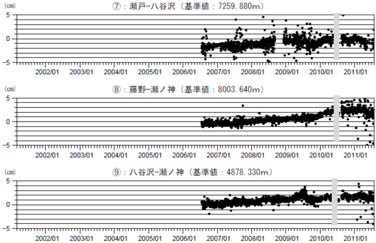
図 10 桜島 GPS 連続観測による長期の基線長変化（2006 年 7 月～2011 年 7 月）
