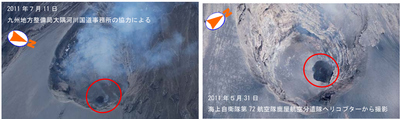
図 14 桜島 昭和火口内の状況（左：2011 年 7 月 11 日、右：2011 年 5 月 31 日） ・火口底に溶岩（図中赤丸）が上昇している様子が認められました。また、溶岩中央部に赤熱した部分が認められました。 ・この溶岩は火口底部北東側に位置し直径 30～40m 程度でした。
