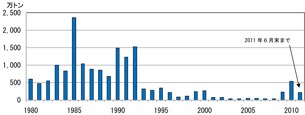
図 13※ 桜島 鹿児島県が実施している降灰量観測による年別降灰量
