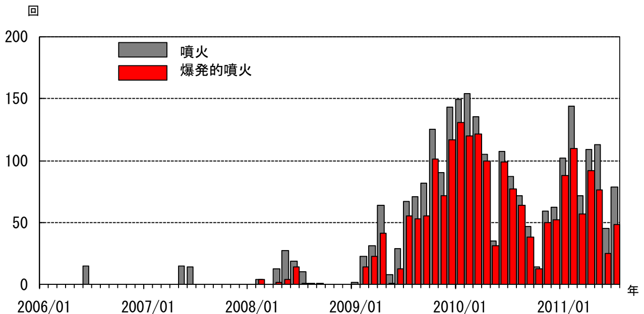
図 4 桜島 昭和火口月別噴火回数（灰色）と昭和火口月別爆発回数（赤色） （2006 年 1 月～2011 年 7 月）
