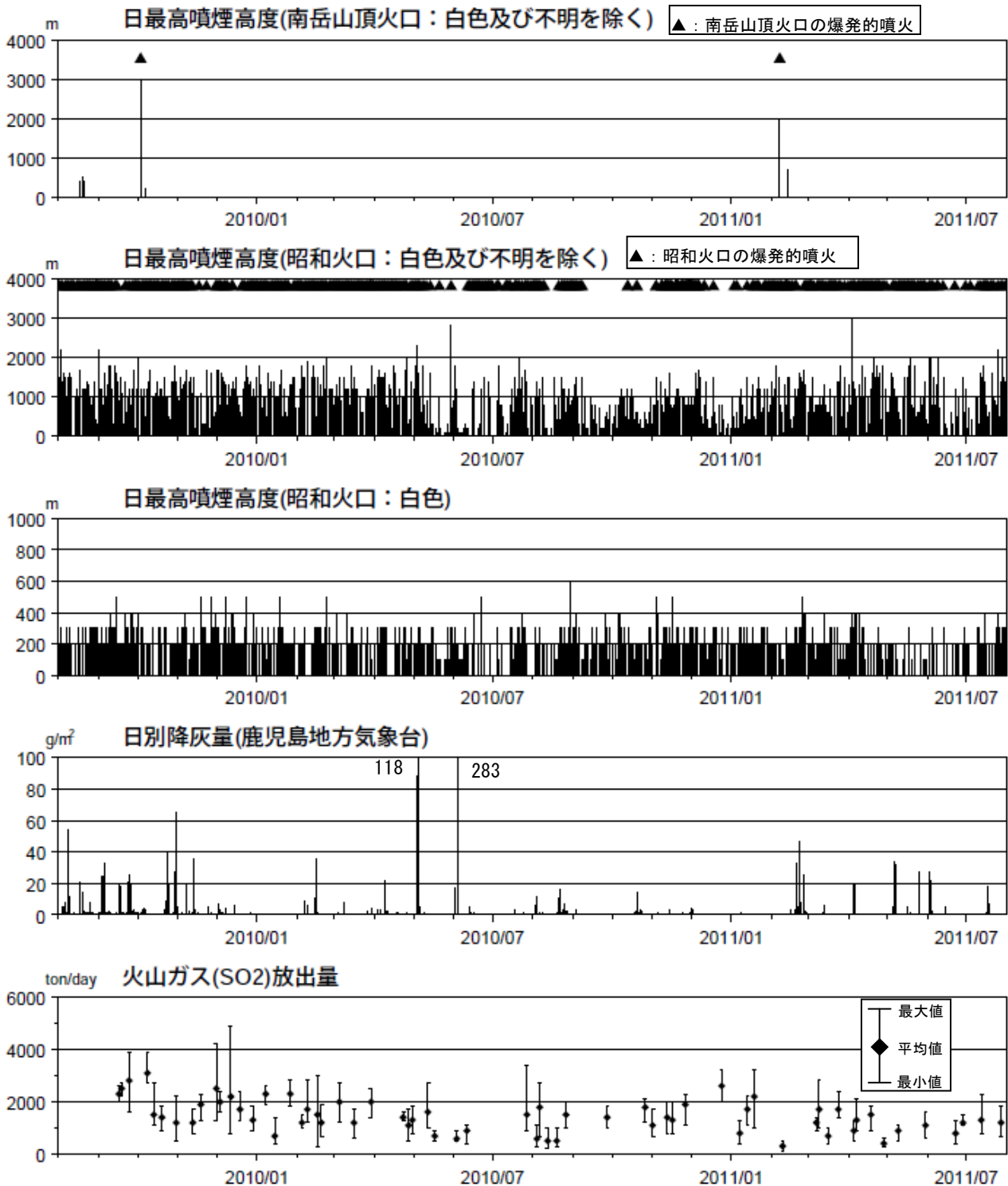
図5 桜島 最近2年間の噴煙、降灰、火山ガス（2009年8月～2011年7月）
