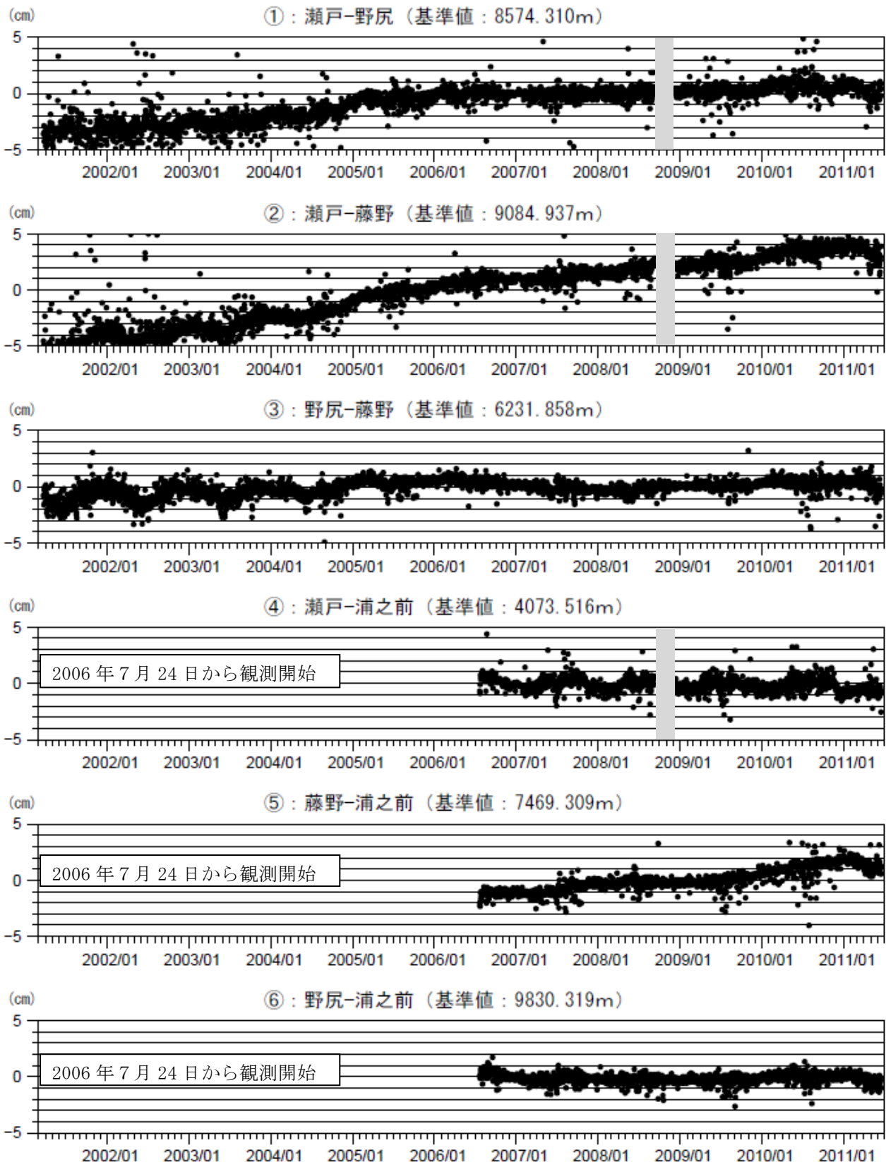
図 10 桜島 GPS 連続観測による長期の基線長変化（2001 年 3 月～2011 年 6 月）
