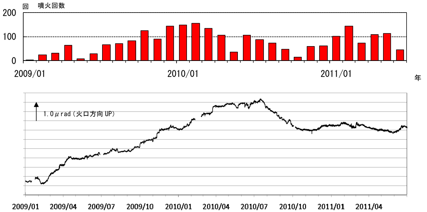
図 9※ 桜島 有村観測坑道の水管傾斜計（大隅河川国道事務所設置）の変化 （2009 年 1 月～2011 年 6 月） 特段の変化は認められませんでした。
