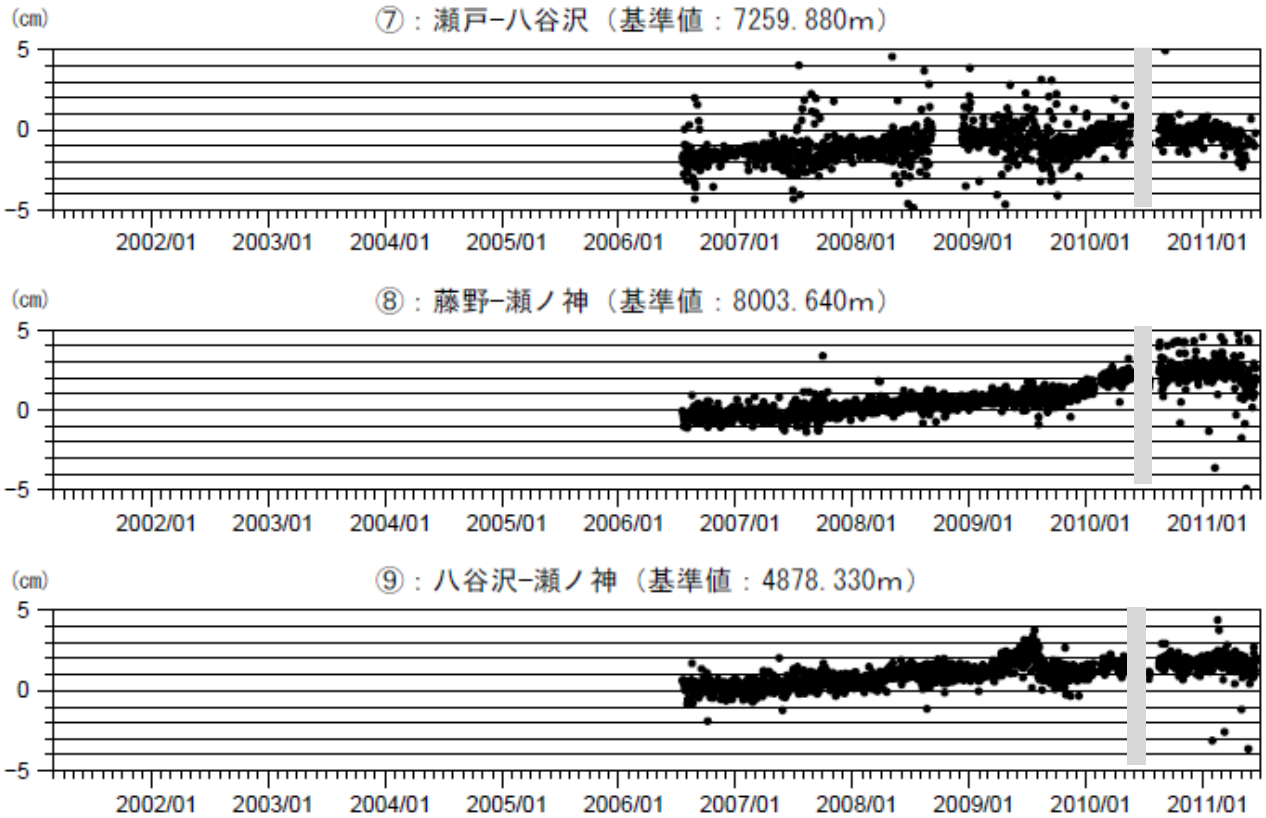
図 11 桜島 GPS 連続観測による長期の基線長変化（2006 年 7 月～2011 年 6 月）
